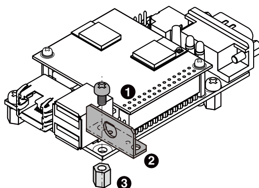
図 6.159 Armadillo-640 へのアンテナ固定金具の固定
