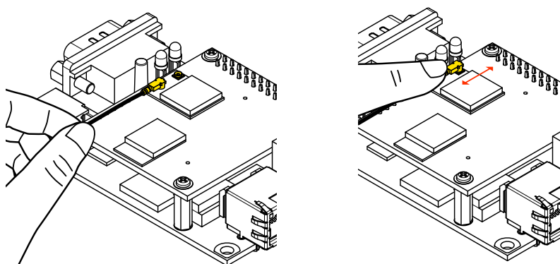
図 6.151 アンテナケーブルコネクタのセット
