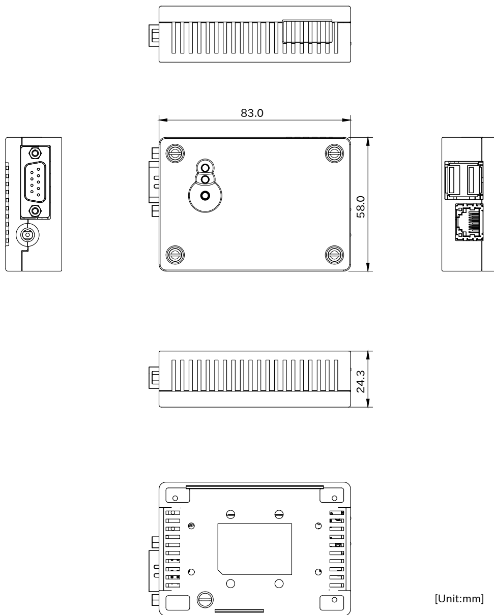
図 6.127 樹脂ケース形状図
