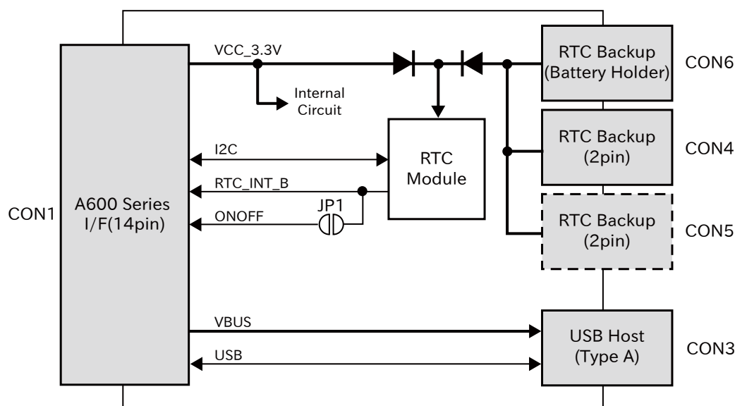
図 6.131 RTC オプションモジュールのブロック図
