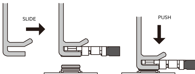
図 6.150 挿抜治具によるアンテナケーブルコネクタの嵌合
