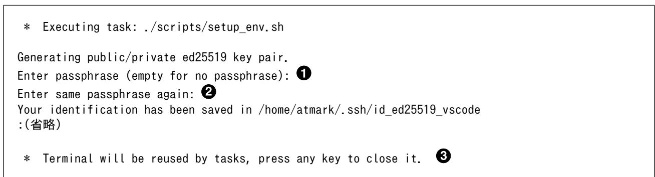
図 3.131 SSH 用の鍵を生成する
