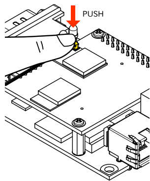
図 6.152 アンテナケーブルコネクタの嵌合
