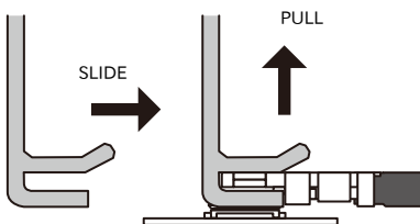
図 6.161 挿抜治具によるアンテナケーブルコネクタの抜去
