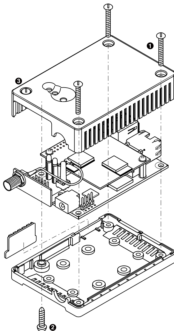
図 6.153 ケースの組み立て
