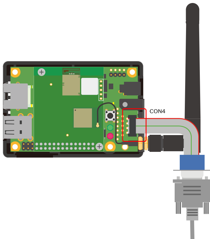
図 6.155 CON4 をシリアルコンソールとして使用する場合の接続例
