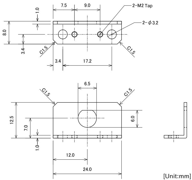
図 6.169 アンテナ固定金具 形状図
