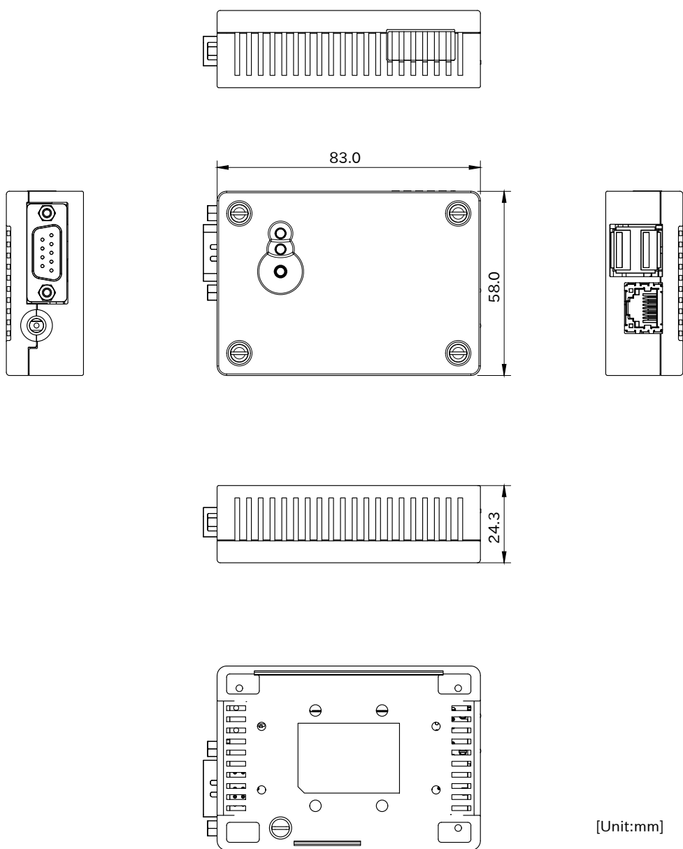
図 6.135 樹脂ケース形状図
