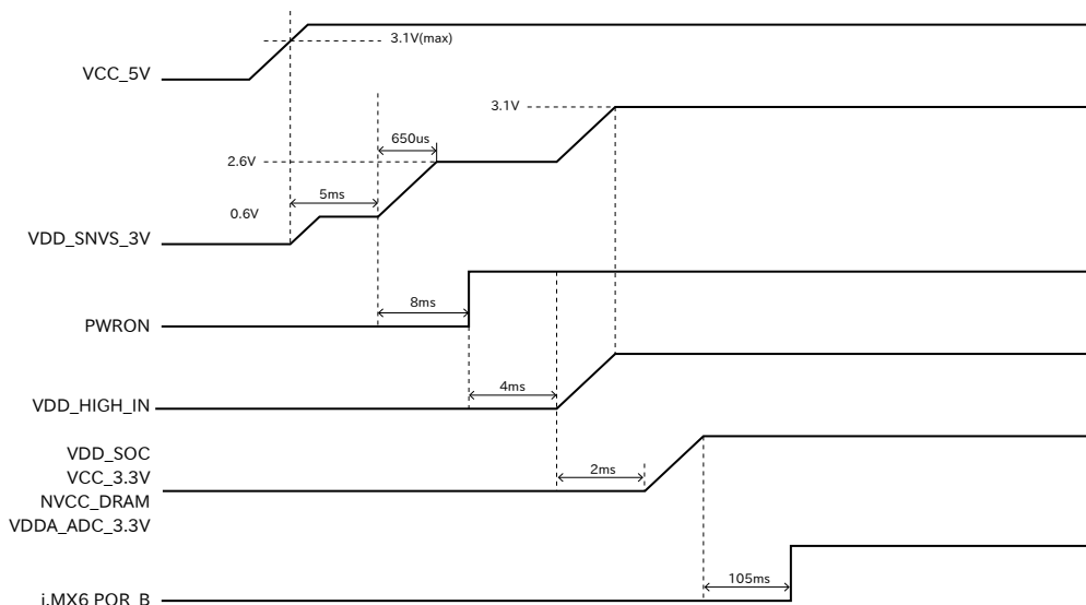
図 3.26 電源シーケンス
