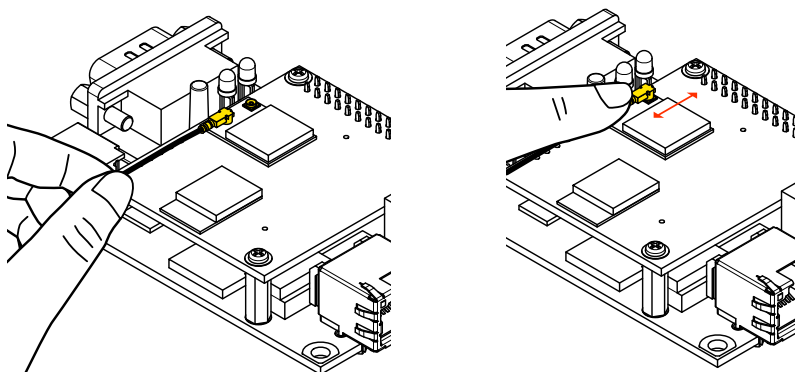
図 6.159 アンテナケーブルコネクタのセット
