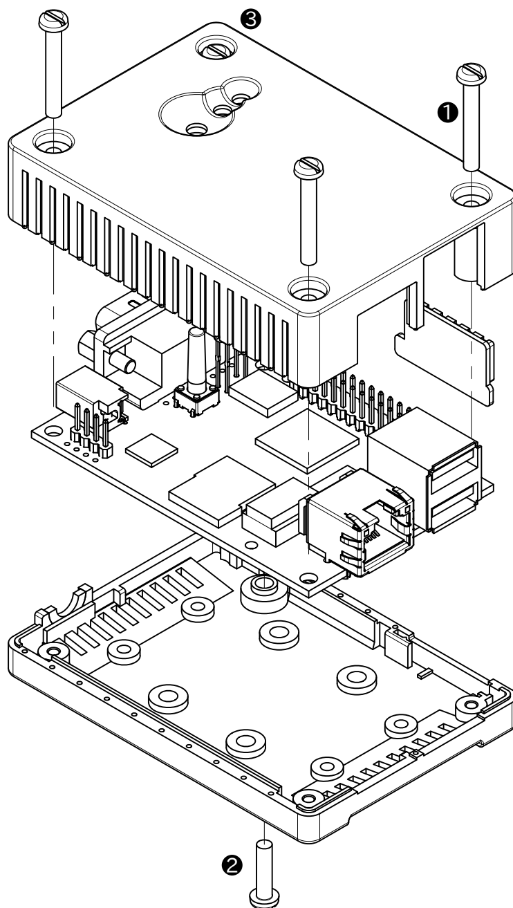
図 6.134 Armadillo-600 シリーズ オプションケース(樹脂製)の組み立て
