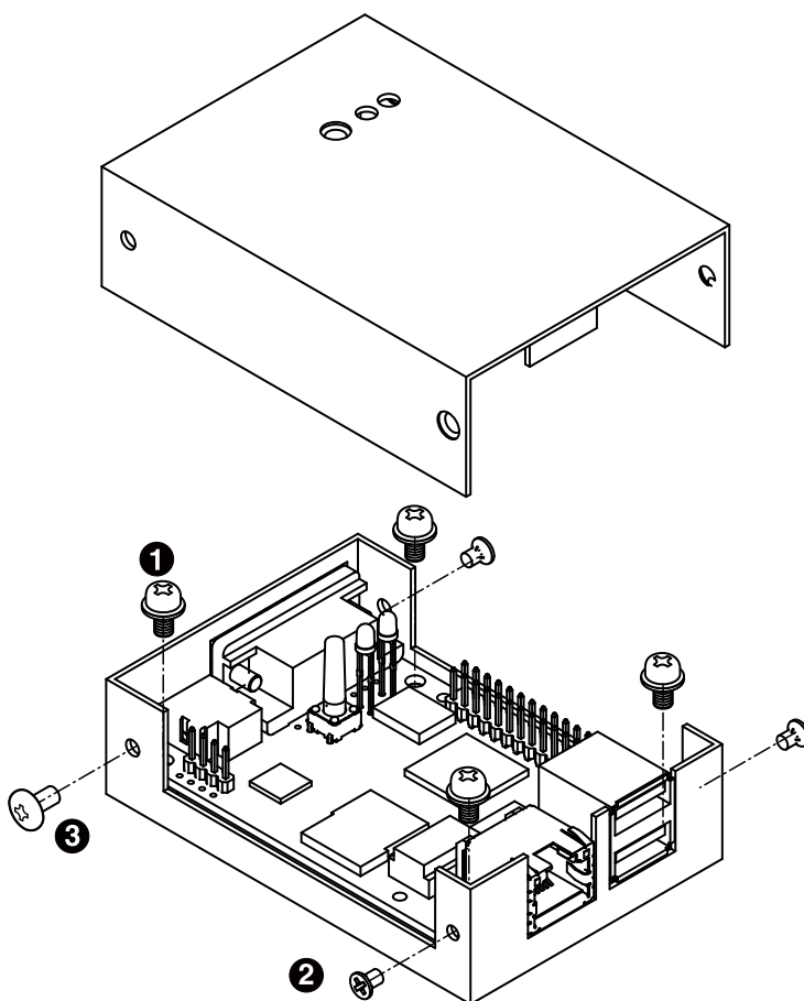
図 6.136 Armadillo-600 シリーズ オプションケース(金属製)の組み立て
