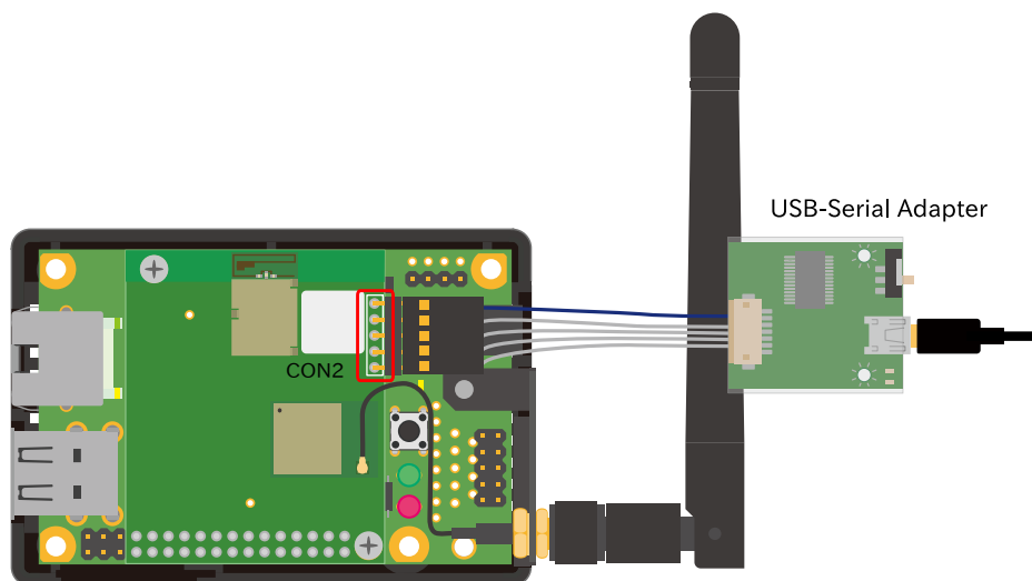
図 6.154 オプションモジュールの CON2 をシリアルコンソールとして使用する場合の接続例
