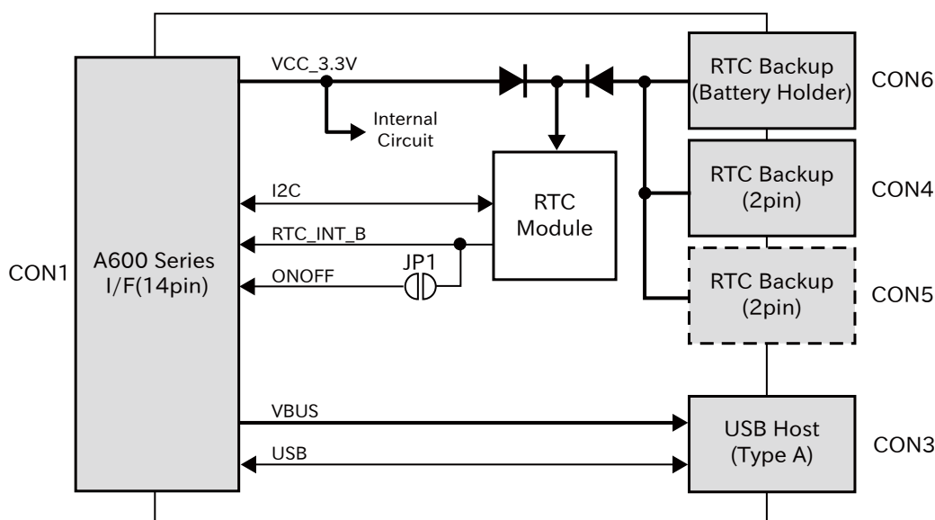
図 6.139 RTC オプションモジュールのブロック図
