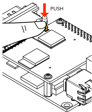
図 6.160 アンテナケーブルコネクタの嵌合
