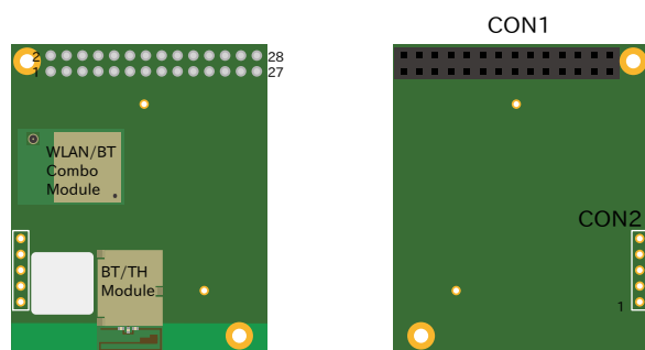
図 6.148 WLAN コンボ、BT/TH オプションモジュールのインターフェース
