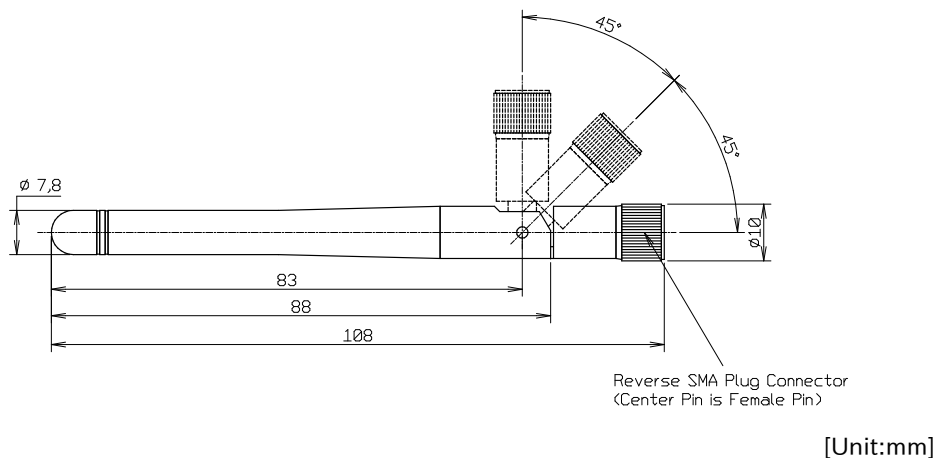
図 6.162 無線 LAN 用 外付けアンテナ 08 形状図
