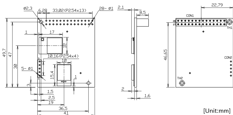
図 6.149 WLAN コンボ、BT/TH オプションモジュール形状図
