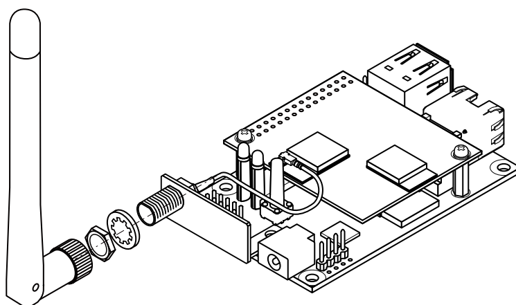
図 6.152 外付けアンテナの組み立て(オプションケース対応のアンテナ固定金具使用)
