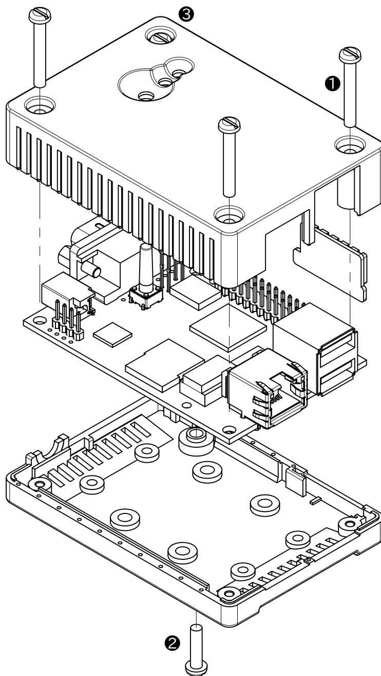
図 6.138 Armadillo-600 シリーズ オプションケース(樹脂製)の組み立て
