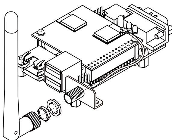
図 6.155 外付けアンテナの組み立て(OP-MNT-ANT-MET-00 使用)
