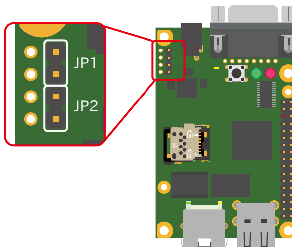
図 3.18 JP1、JP2 の位置
