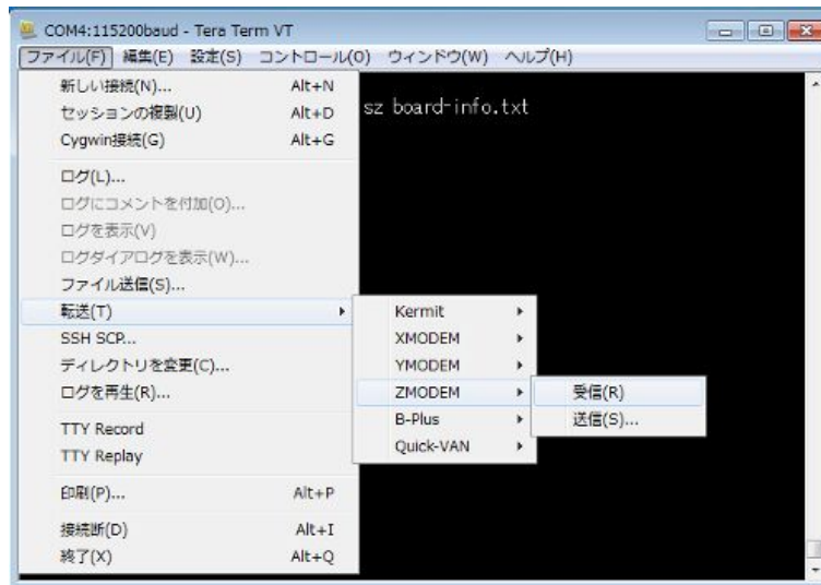
図 7.3 ZMODEM の選択
