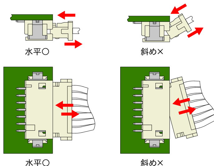
図 3.20 挿抜角度
