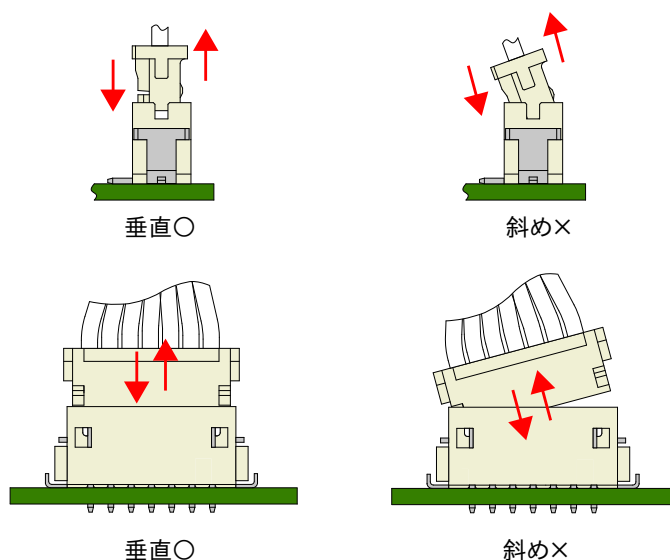
図 3.9 挿抜角度
