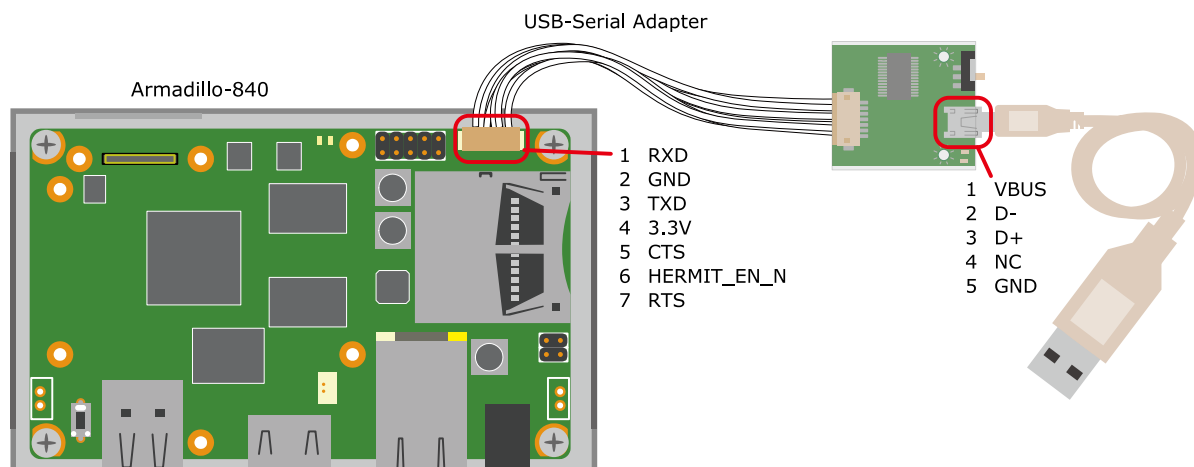
図 19.19 開発用 USB シリアル変換アダプタの配線
