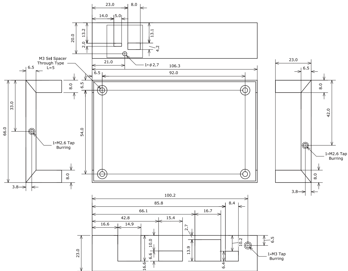
図 19.12 Armadillo-840 オプションケース(金属製)下板寸法図
