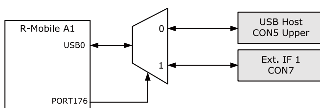
図 17.2 USB の切り替え
