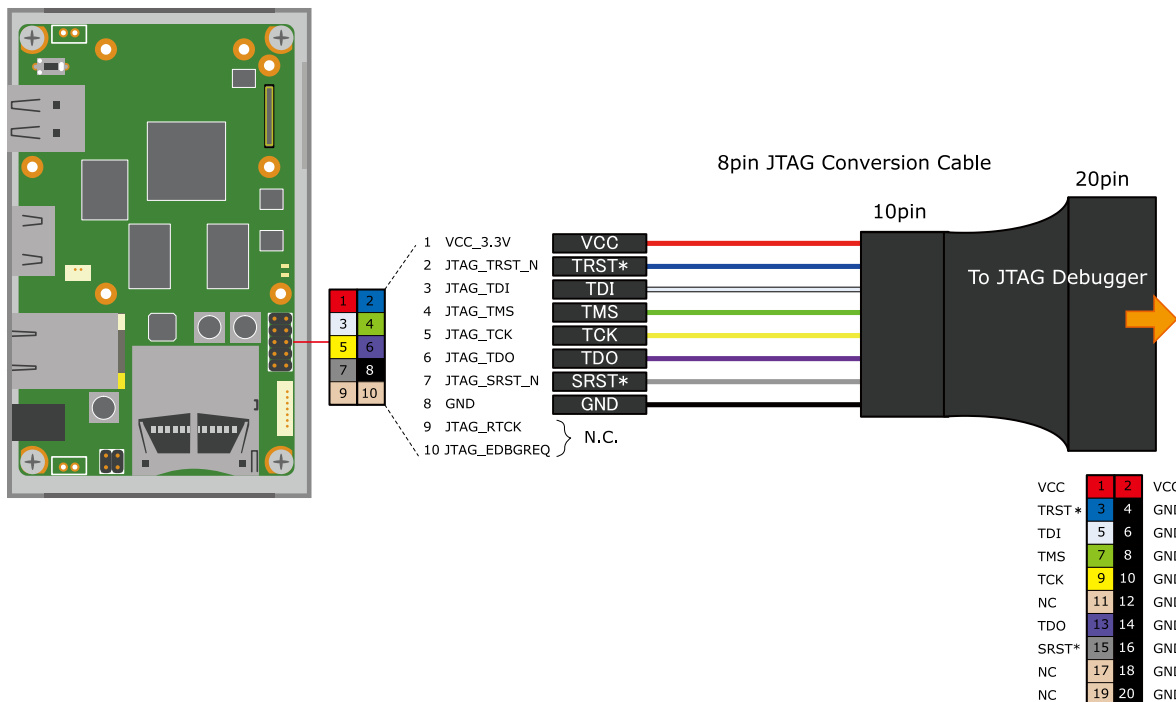
図 19.21 8 ピン JTAG 変換ケーブルの接続図
