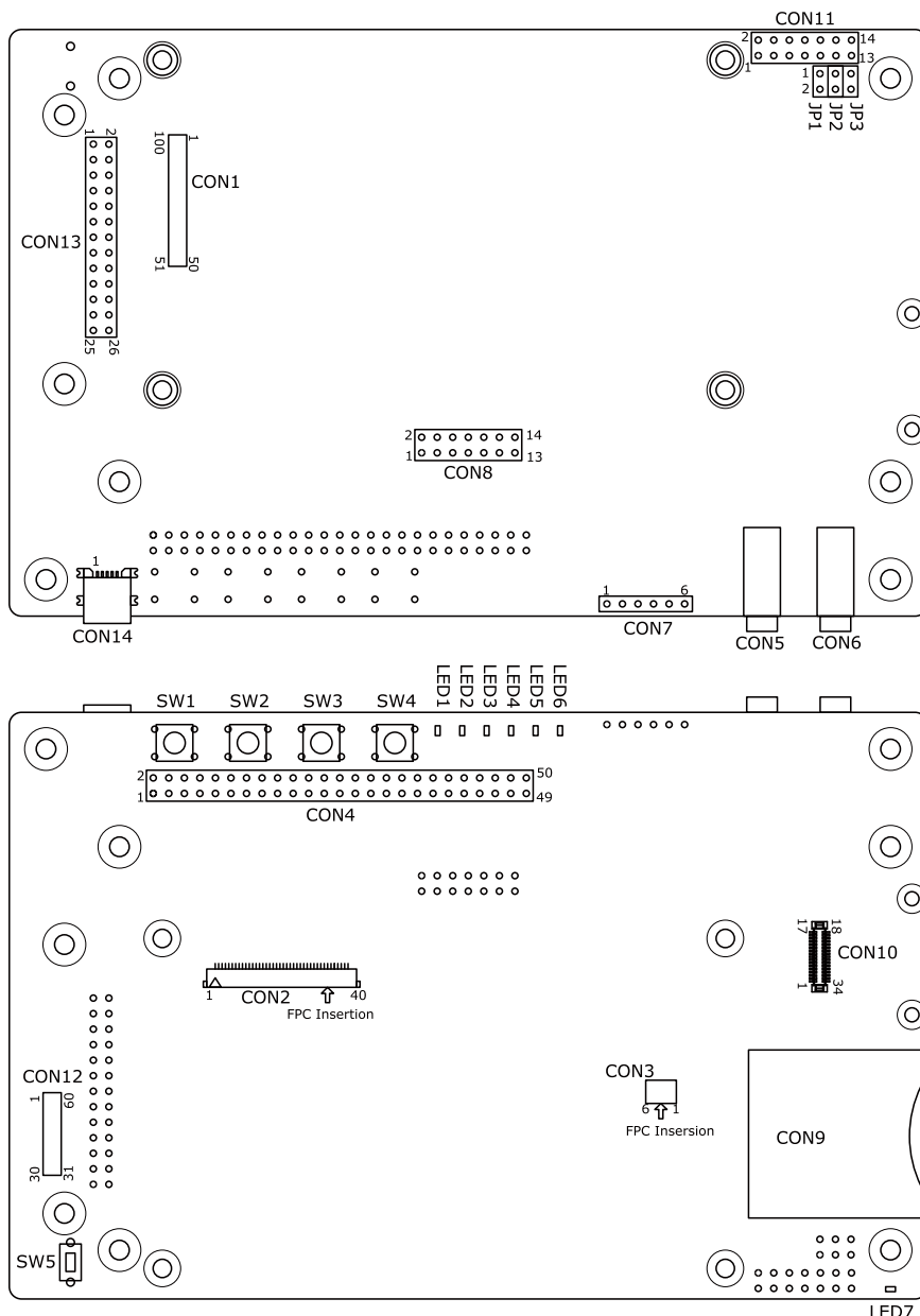
図 19.2 Armadillo-840 拡張ボード 01(C コネクタ用) インターフェースレイアウト図
