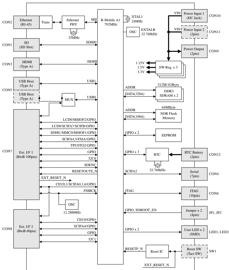
図 3.4 Armadillo-840 ブロック図
