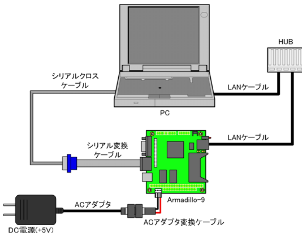
図 2.1. Armadillo-9 接続例
