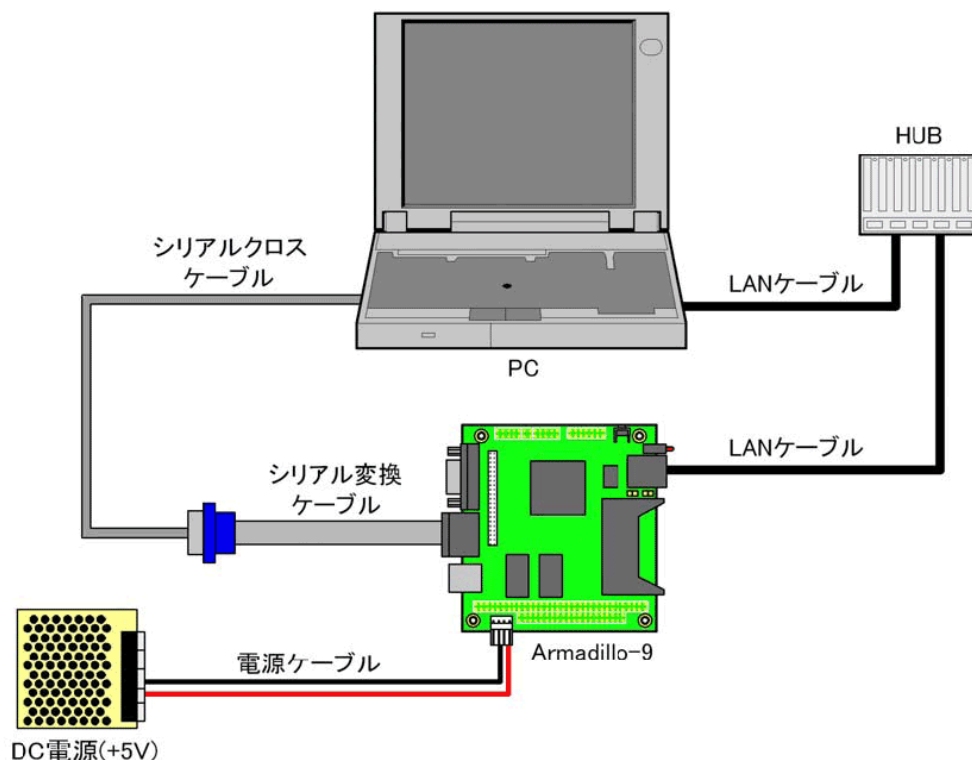
図 2.2. 接続図
