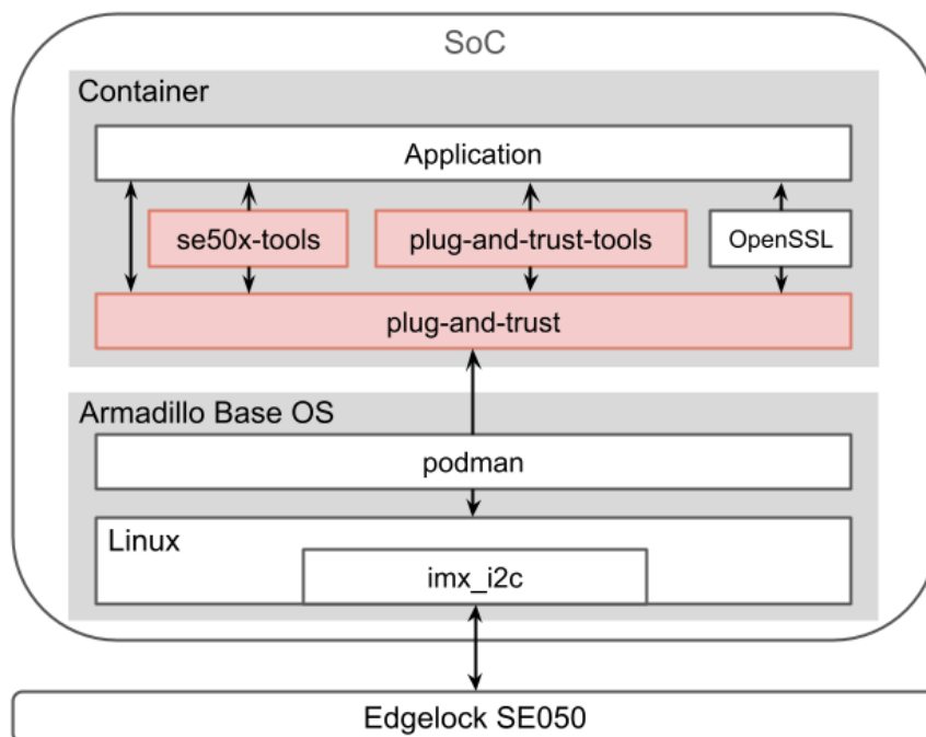
図 10.118 Plug &amp; Trust Middleware の周辺のソフトウェアスタック
