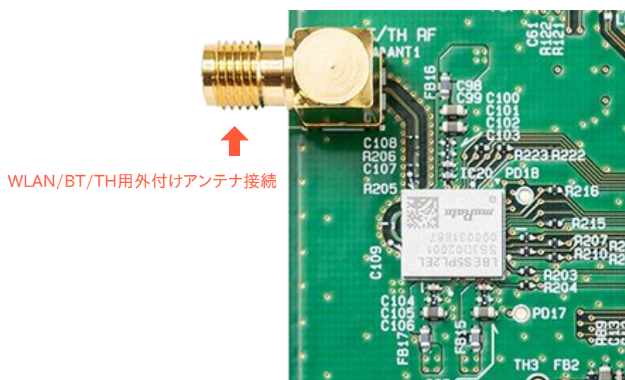
図 5.80 WLAN/BT/TH 用外付けアンテナ接続
