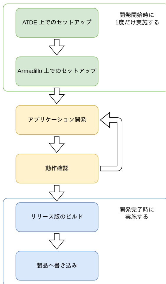
図 7.101 CUI アプリケーション開発の流れ
