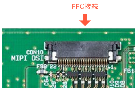
図 5.118 MIPI DSI FFC 接続
