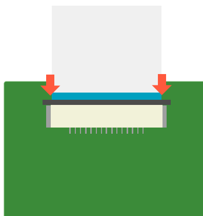
図 5.116 MIPI CSI インターフェース FFC 接続方法
