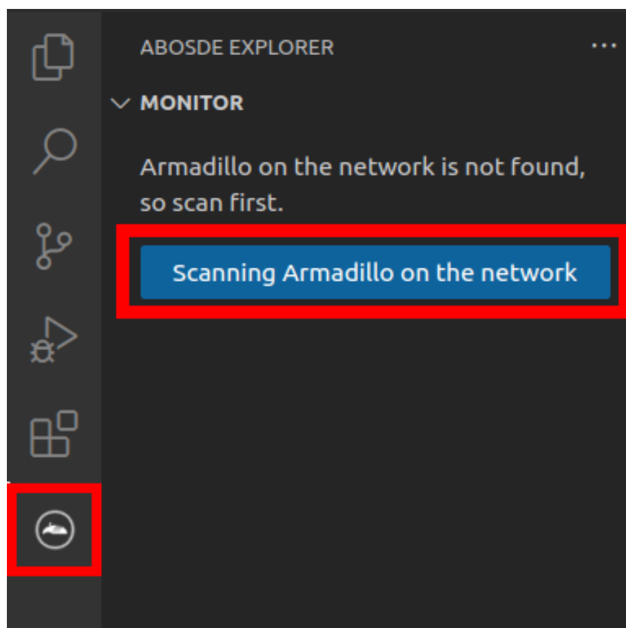
図 7.86 ABOSDE で ローカルネットワーク上の Armadillo をスキャンする
