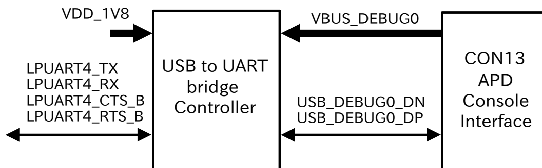
図 5.122 APD 用コンソールインターフェース回路構成
