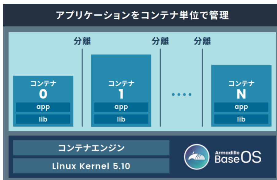
図 2.2 コンテナによるアプリケーションの運用
