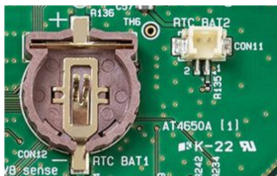
図 5.131 RTC バックアップインターフェース
