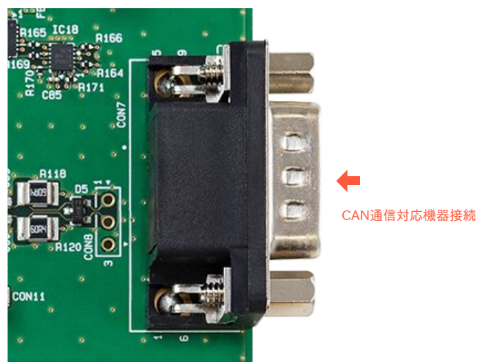
図 5.113 CAN 通信対応機器接続
