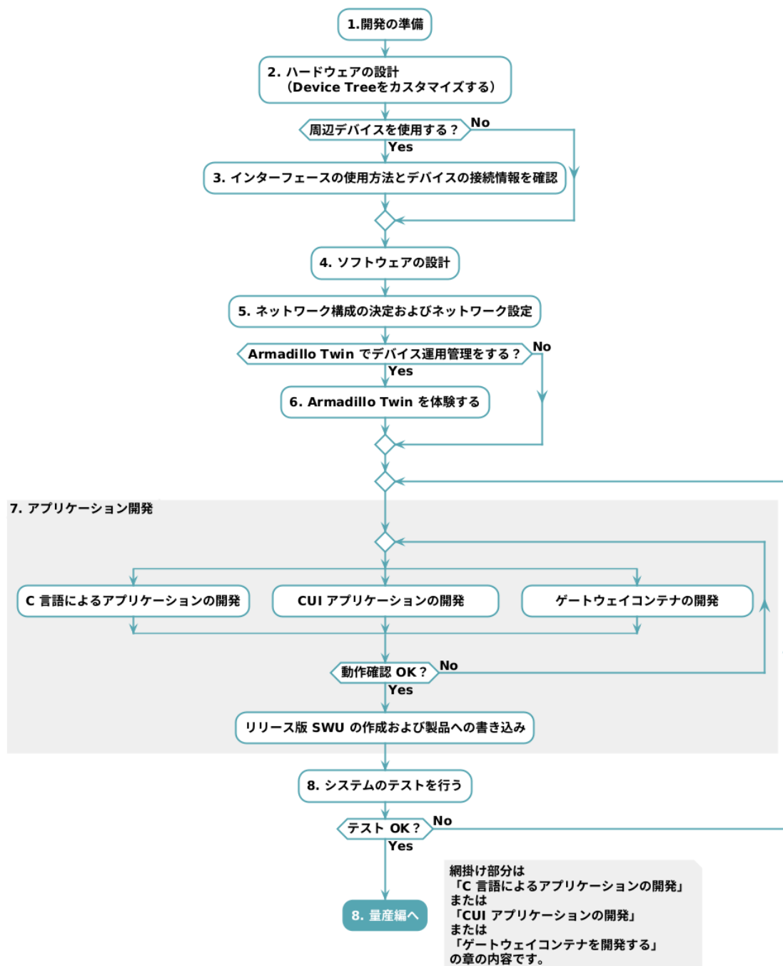
図 7.37 アプリケーション開発の流れ
