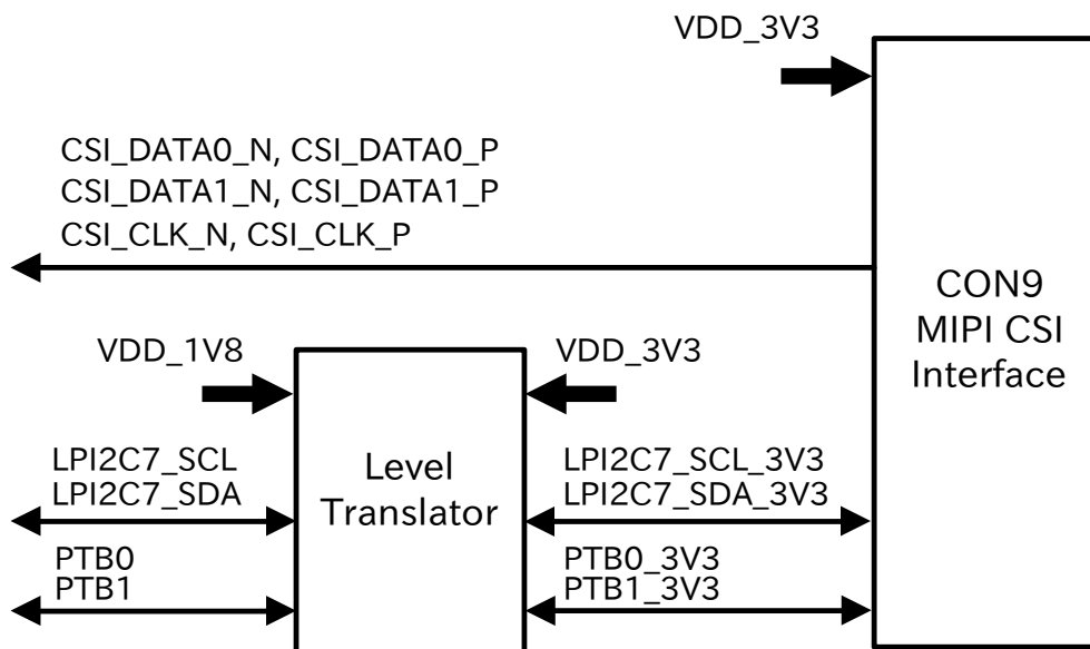
図 5.117 MIPI CSI インターフェース回路構成
