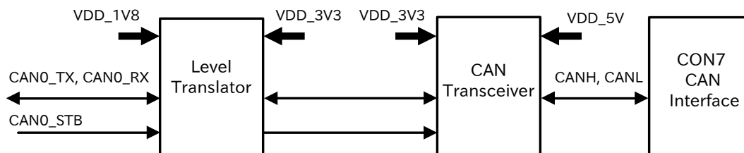
図 5.114 CAN インターフェース回路構成
