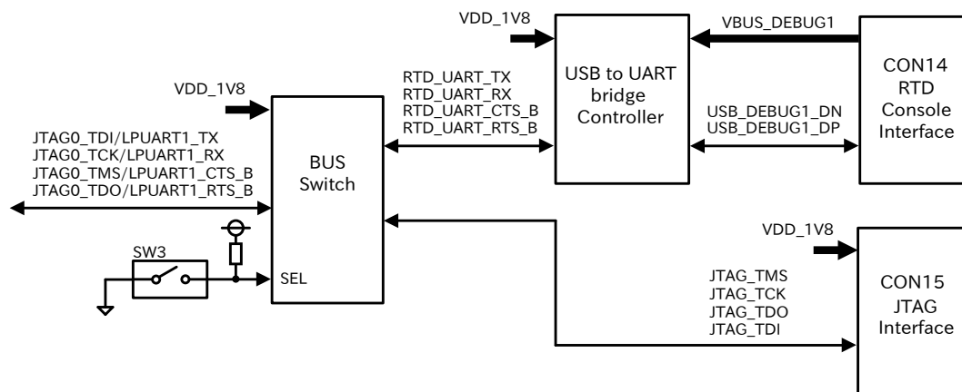
図 5.126 RTD 用コンソールインターフェース回路構成
