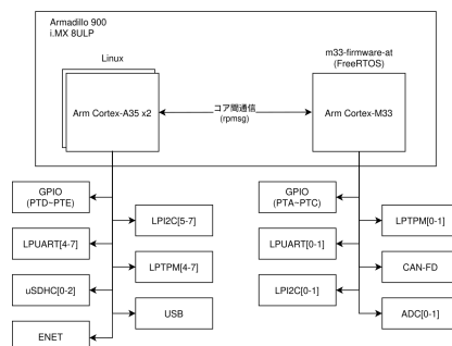
図 7.49 Armadillo-900 で使用している i.MX 8ULP の簡易構造
