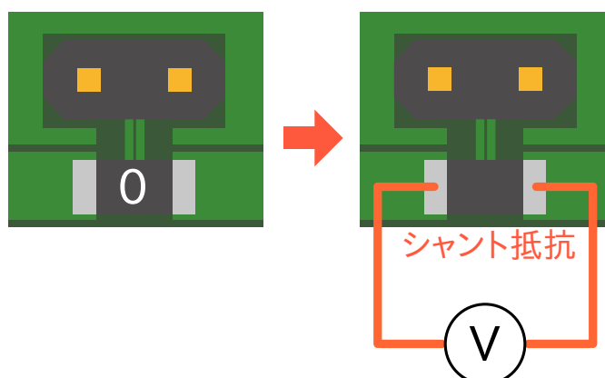
図 5.176 電流測定(シャント抵抗に電圧計を接続)
