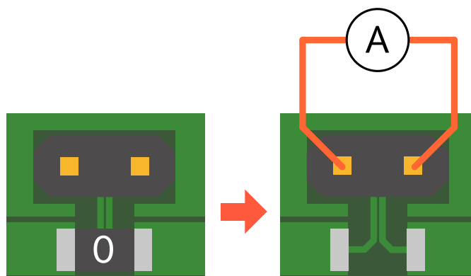
図 5.175 電流測定(ピンヘッダに電流計を接続)
