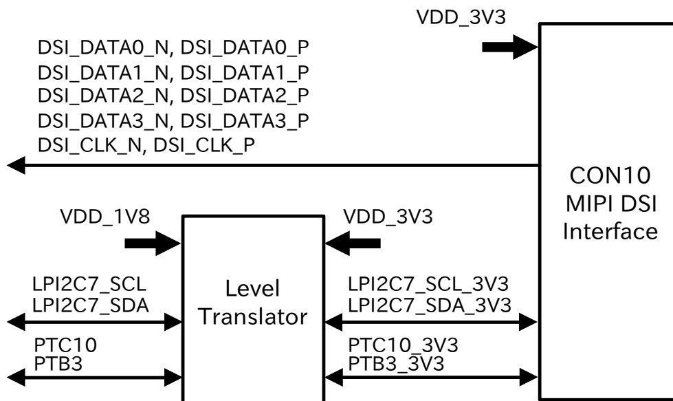
図 5.120 MIPI DSI インターフェース回路構成
