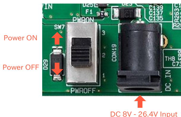
図 5.73 電源入力
