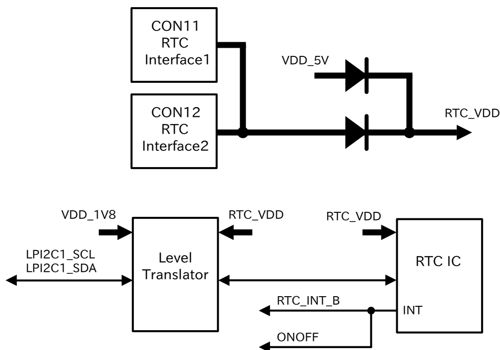
図 5.132 RTC バックアップインターフェース回路構成
