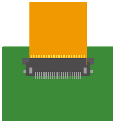
図 5.119 MIPI DSI インターフェース FFC 接続方法
