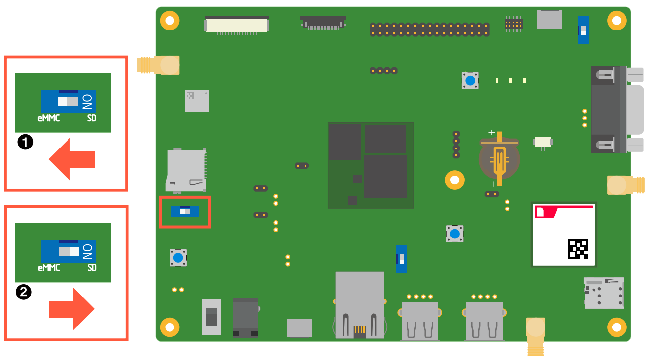
図 5.171 スイッチの状態と起動デバイス
