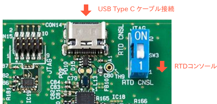
図 5.123 USB Type C ケーブル接続/切替スイッチ制御
