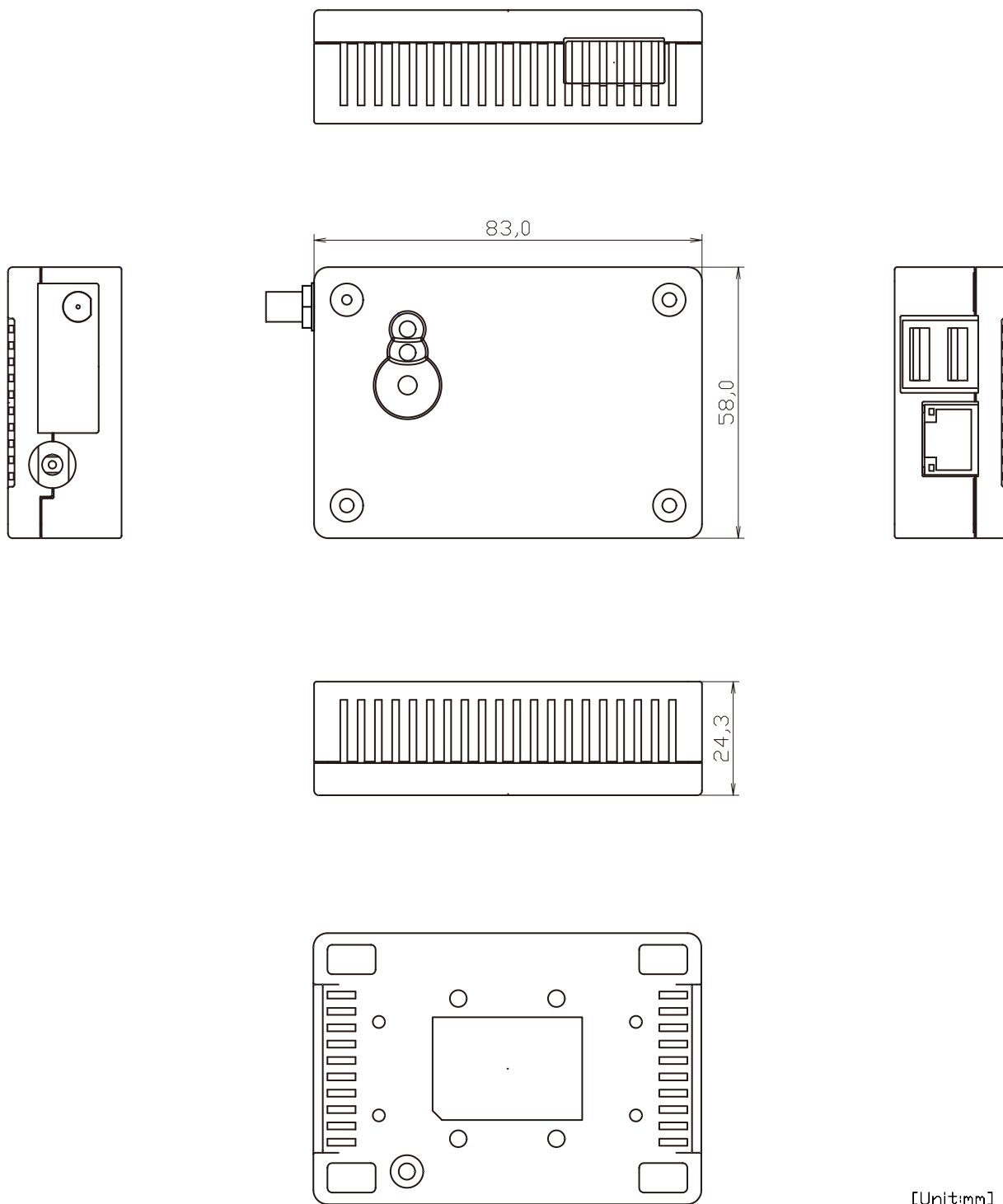
図 19.1 筐体寸法図
