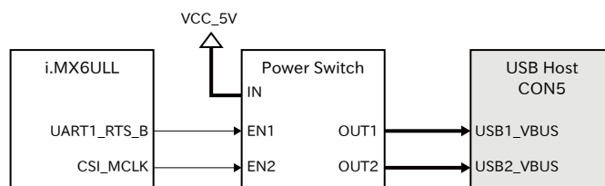
図 18.5 USB ホストインターフェースの電源制御
