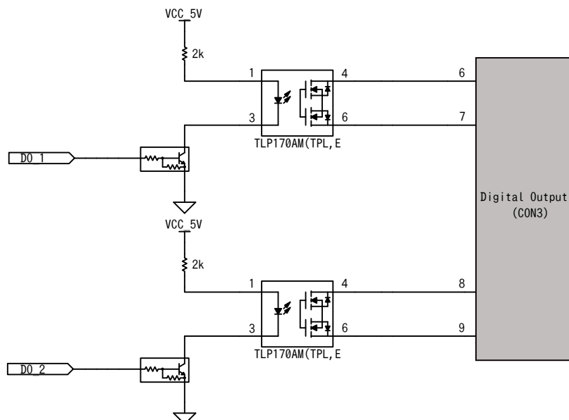
図 20.8 CON3 デジタル出力部
