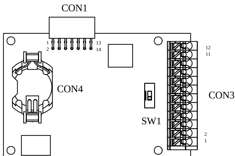
図 20.6 Armadillo-IoT ゲートウェイ A6 U1 モデル用 拡張 I/O ボード 01 インターフェースレイアウト
