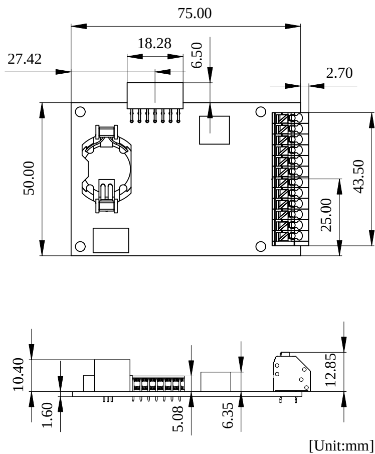
図 20.12 基板形状およびコネクタ中心寸法
