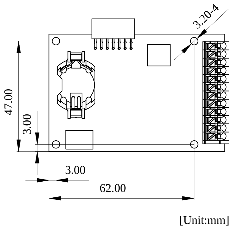
図 20.13 固定穴寸法
