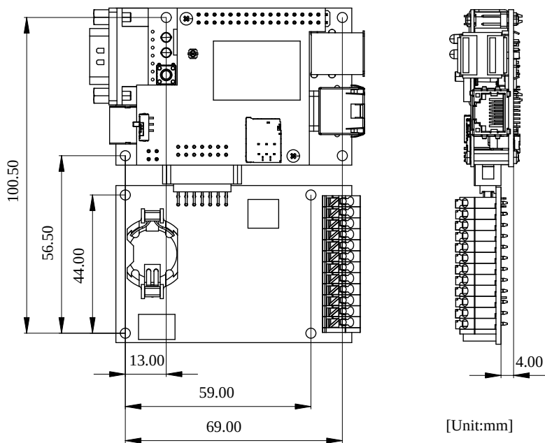
図 20.14 組立後固定穴寸法
