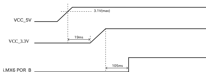
図 17.2 電源シーケンス
