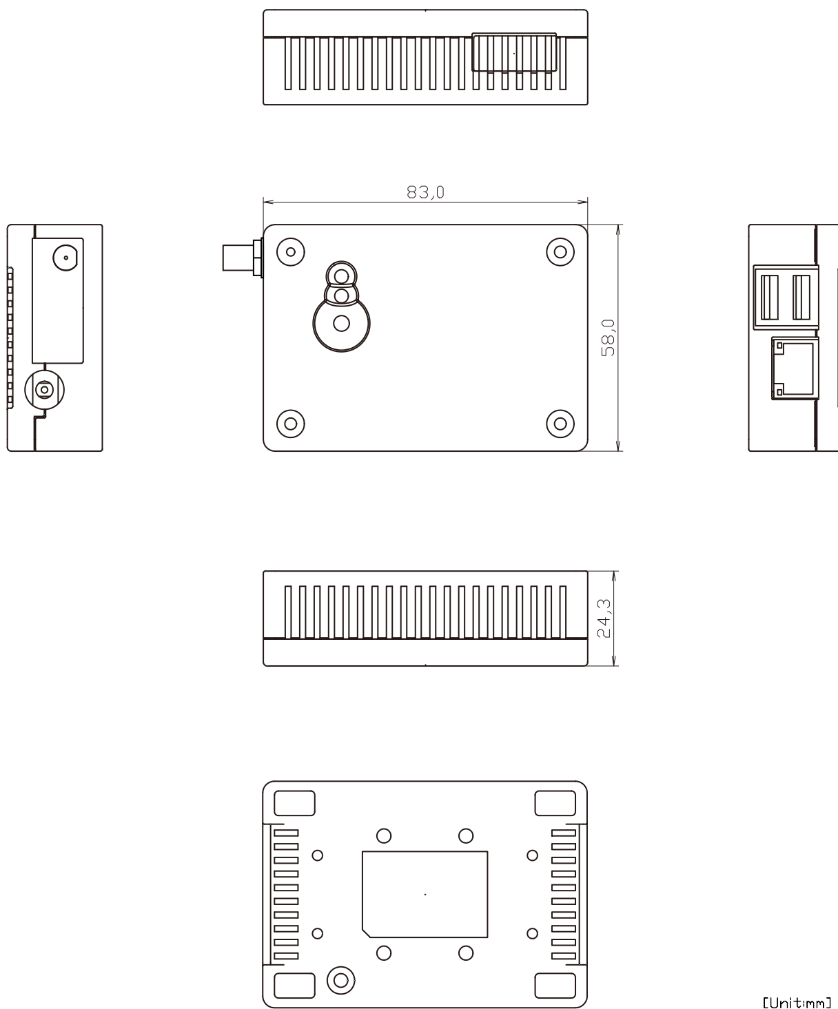
図 19.1 筐体寸法図
