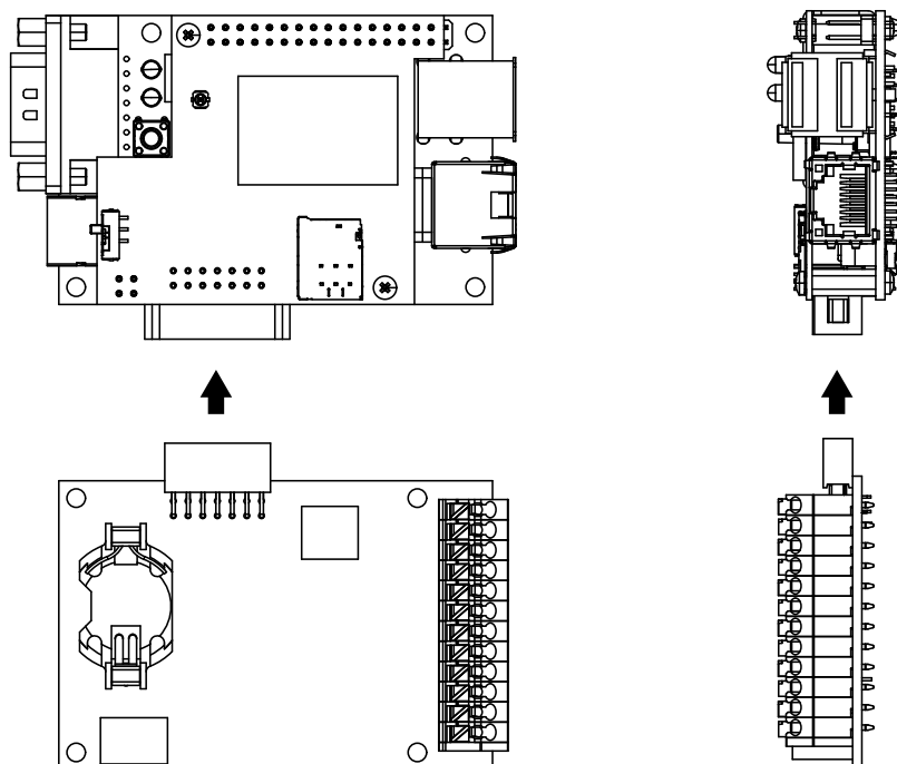
図 20.10 組み立て図
