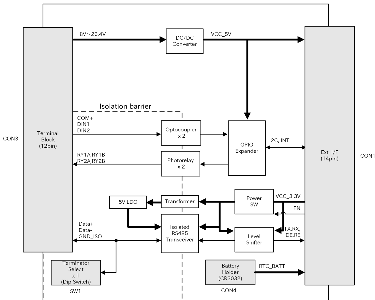
図 20.5 Armadillo-IoT ゲートウェイ A6 U1 モデル用 拡張 I/O ボード 01 ブロック図
