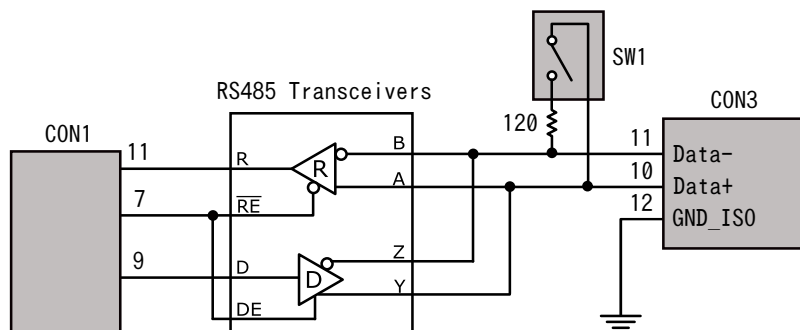
図 20.9 RS-485 トランシーバ周辺回路
