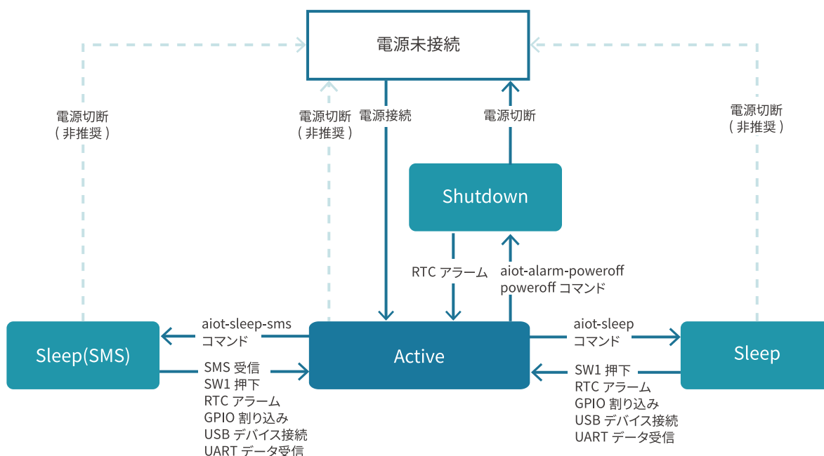
図 7.1 状態遷移図
