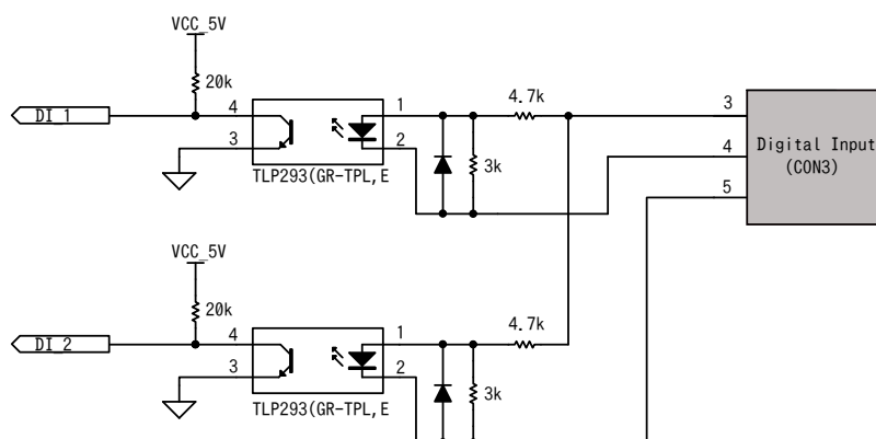
図 20.7 CON3 デジタル入力部
