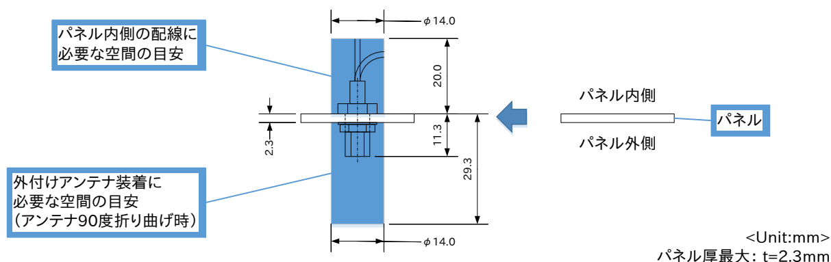
図 20.4 アンテナコネクタ取り付け時の参考図
