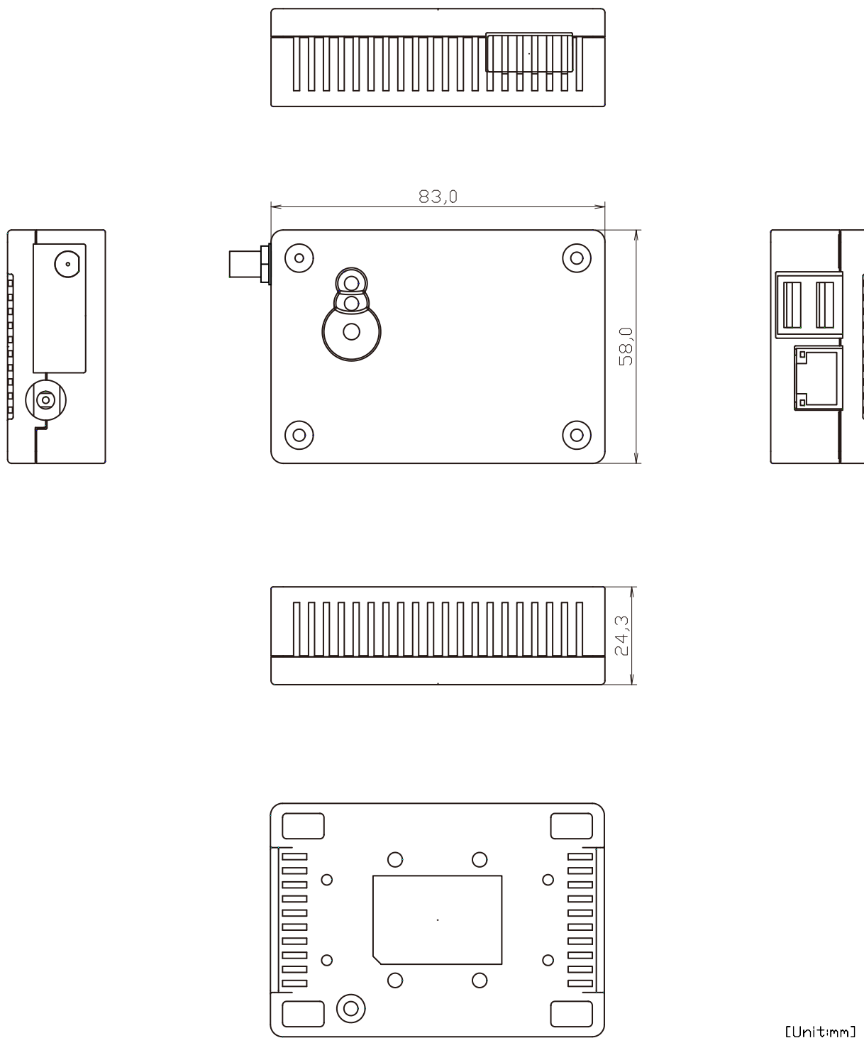
図 19.1 筐体寸法図
