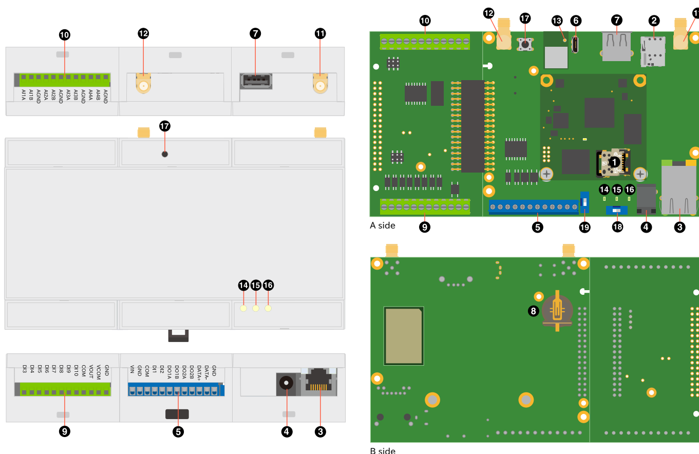
図 3.9 Armadillo-IoT ゲートウェイ A6E +Di8+Ai4 の外観
