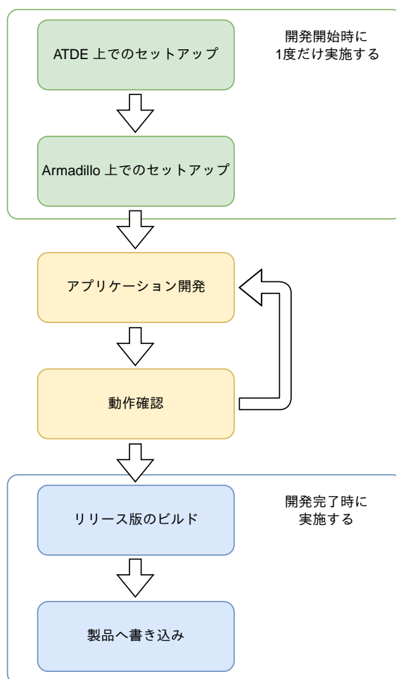
図 11.1 ゲートウェイアプリケーション開発の流れ
