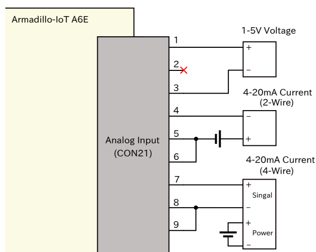
図 15.17 CON21 アナログ入力接続例
