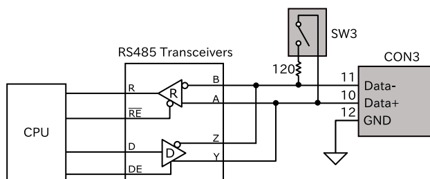
図 15.15 CON6 RS485 トランシーバ周辺回路
