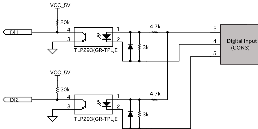
図 15.13 CON6 接点入力周辺回路
