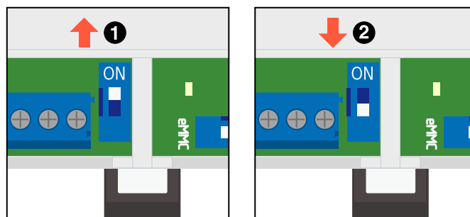
図 15.27 スwitchの状態と終端抵抗の ON/OFF
