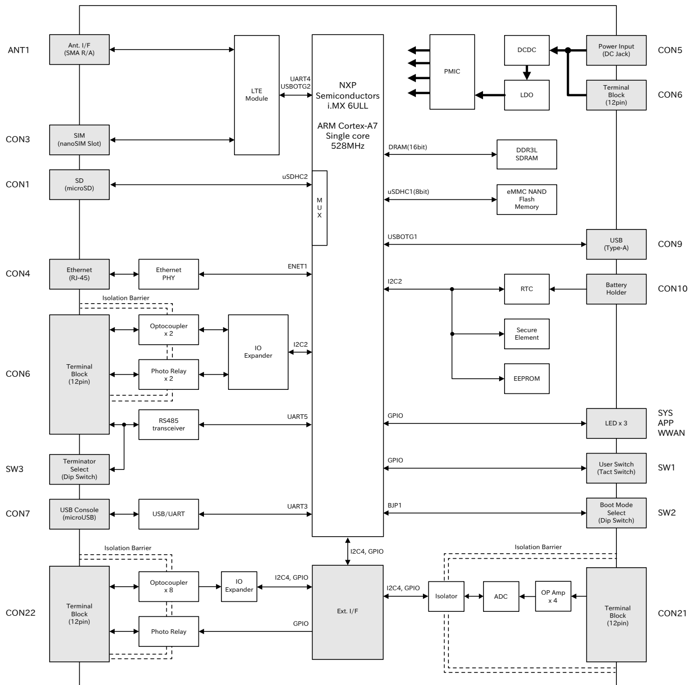
図 3.12 ブロック図(AG6223-C01D0, AG6223-C01Z)
