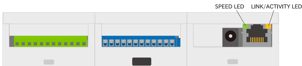
図 15.11 CON4 LAN LED
