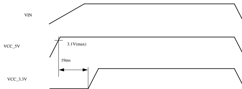
図 15.2 電源シーケンス
