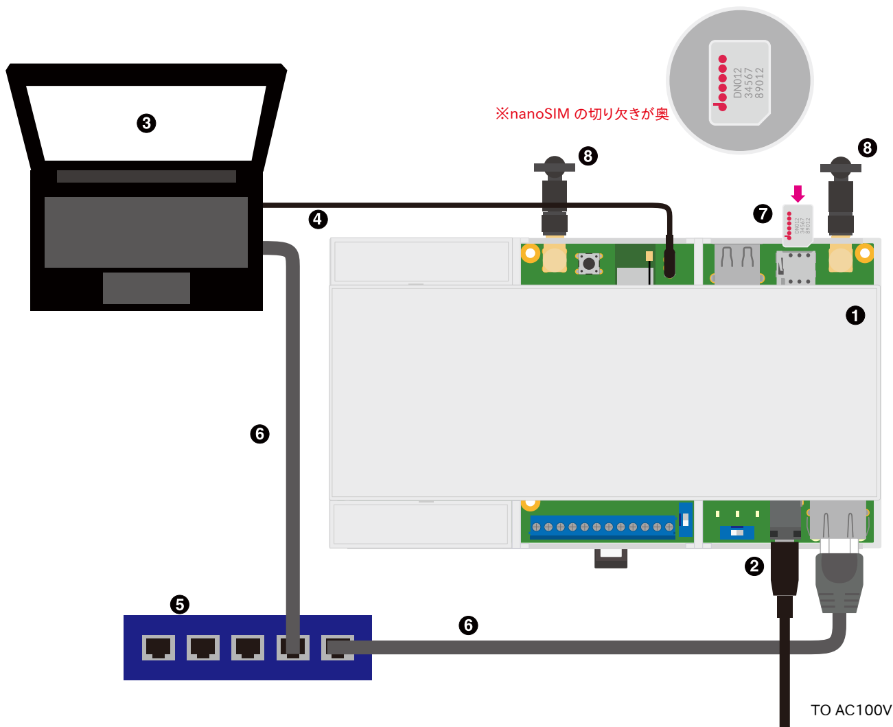
図 4.12 Armadillo-IoT ゲートウェイ A6E +Di8+Ai4 の接続例
