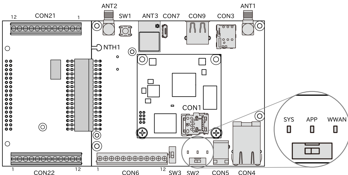
図 15.3 Armadillo-IoT ゲートウェイ A6E +Di8+Ai4 のインターフェース 表面
