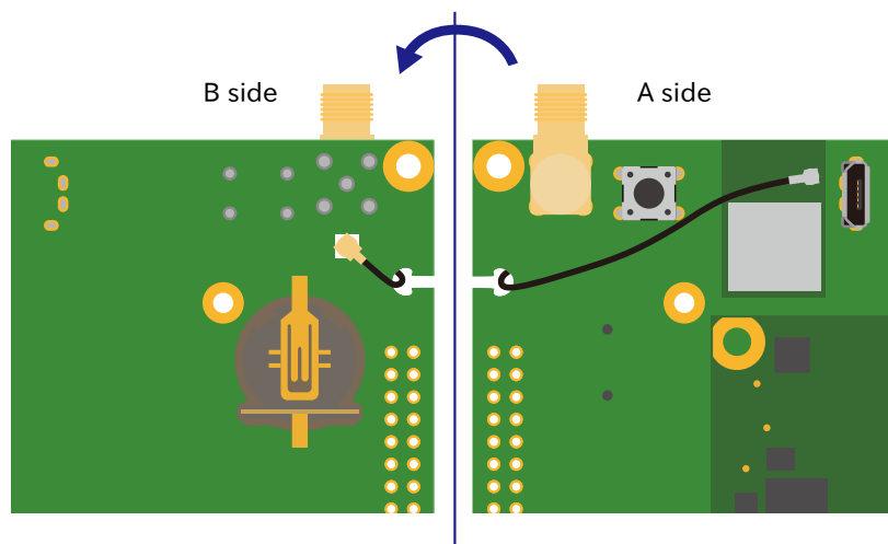
図 15.23 ANT2 カスタマイズ例：同軸ケーブル接続図
