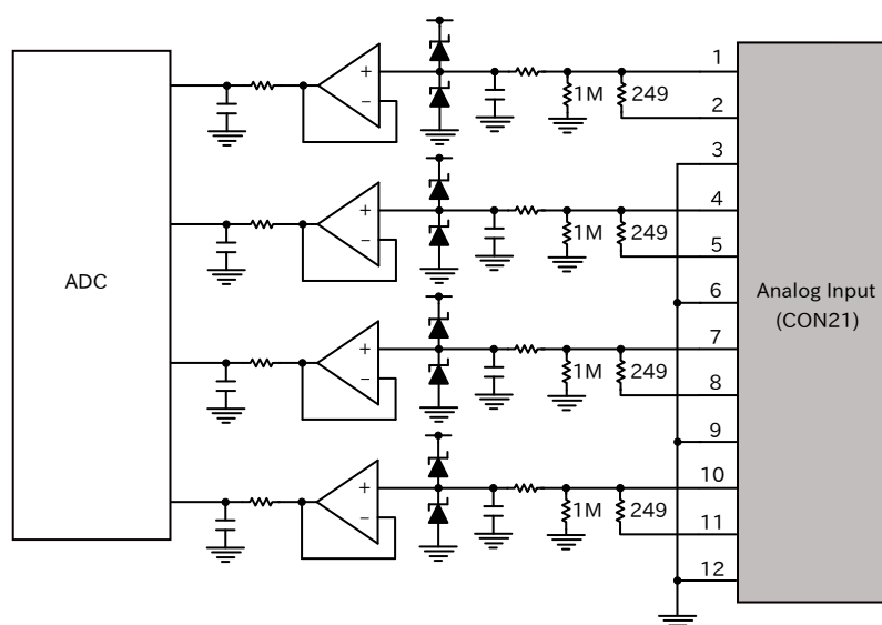
図 15.16 CON21 アナログ入力周辺回路
