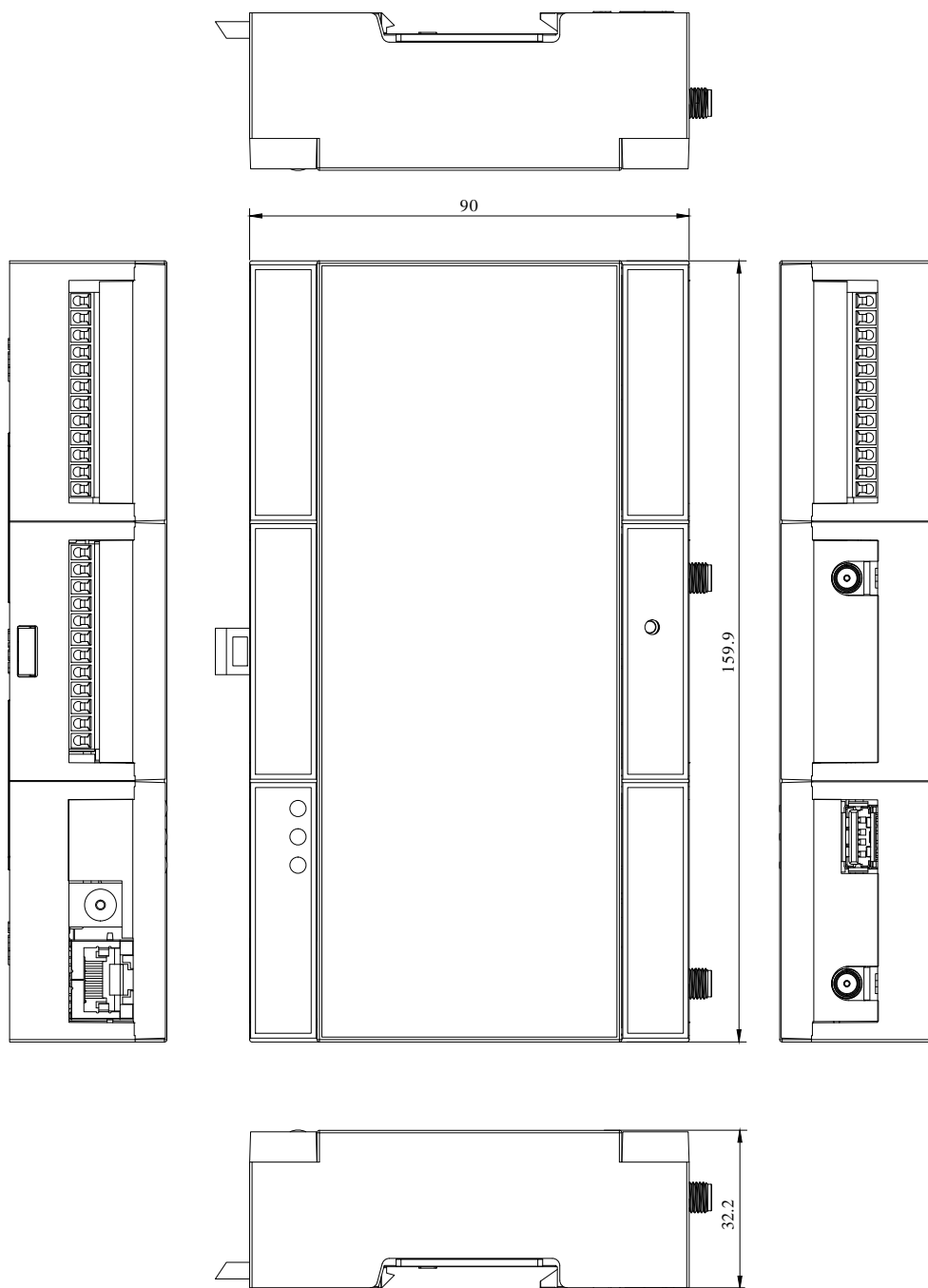
図 15.28 筐体形状
