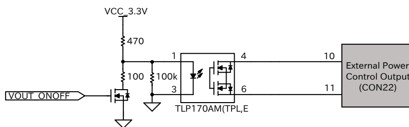
図 15.19 CON22 外部電源制御出力周辺回路
