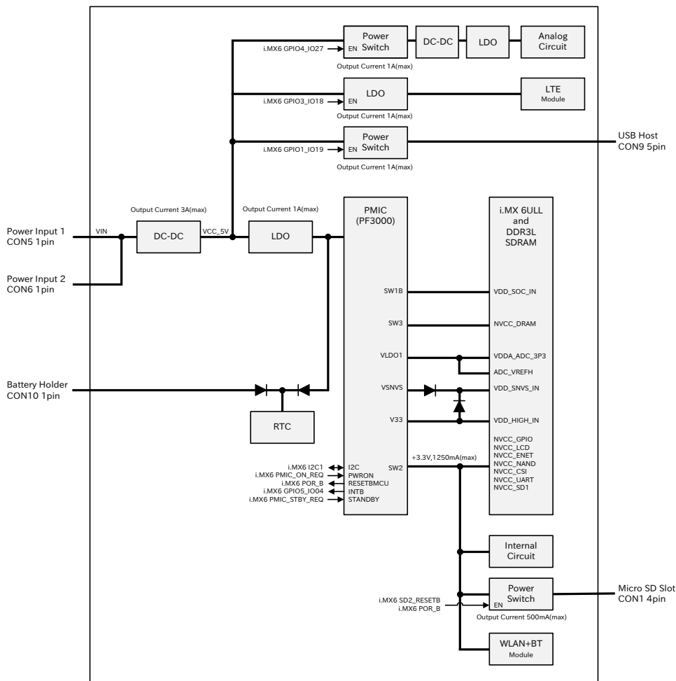
図 15.1 電源回路の構成
