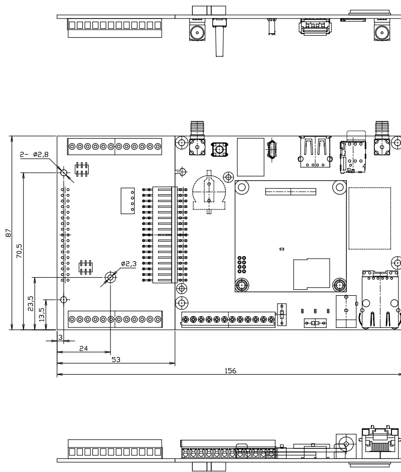
図 15.30 基板形状および固定穴寸法 2
