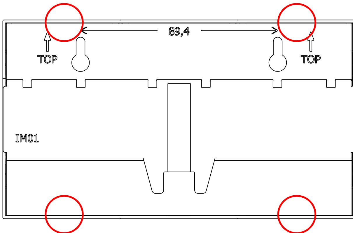
図 15.39 ケースボトムのカム
