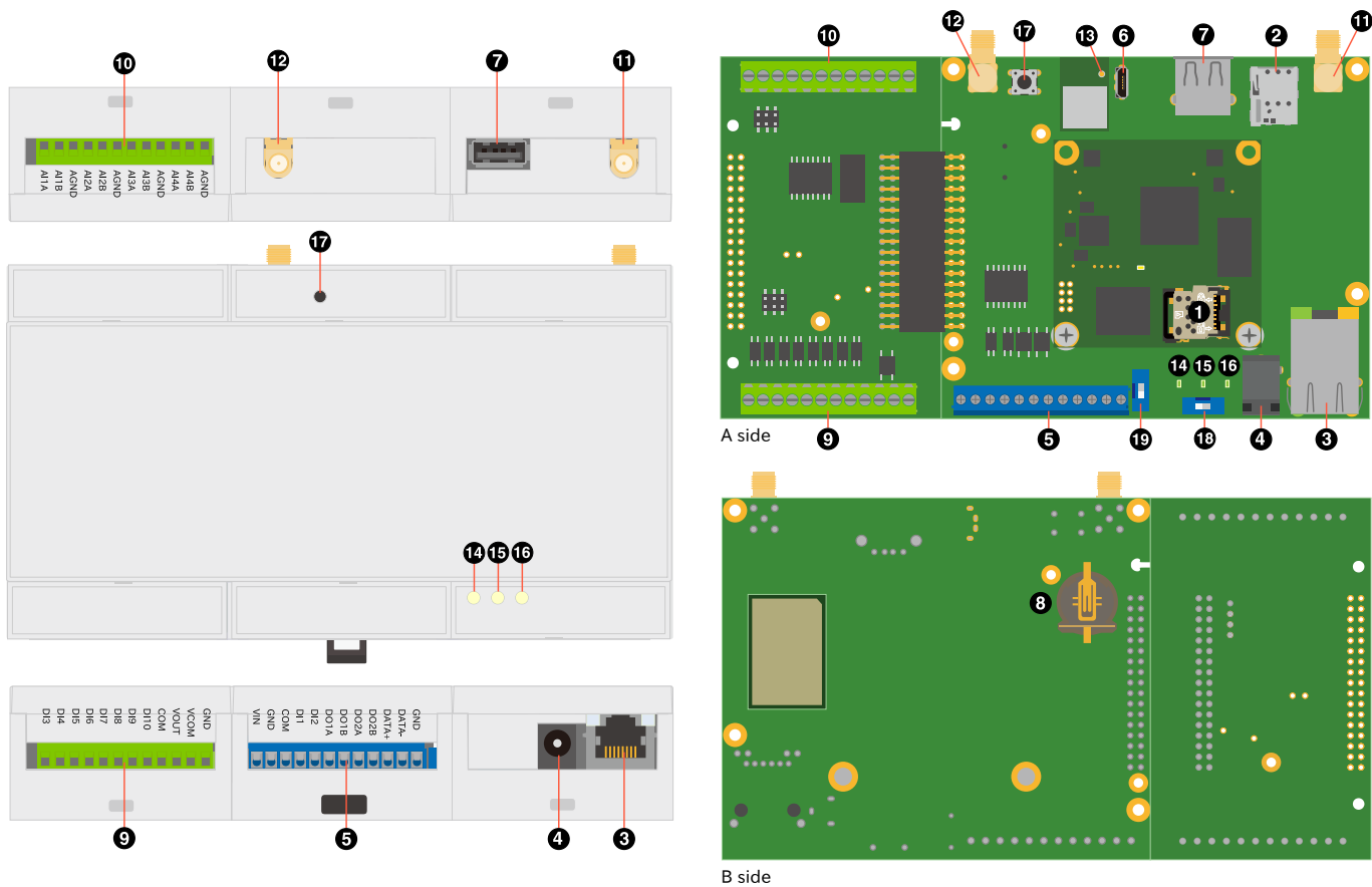
図 4.11 インターフェースレイアウト
