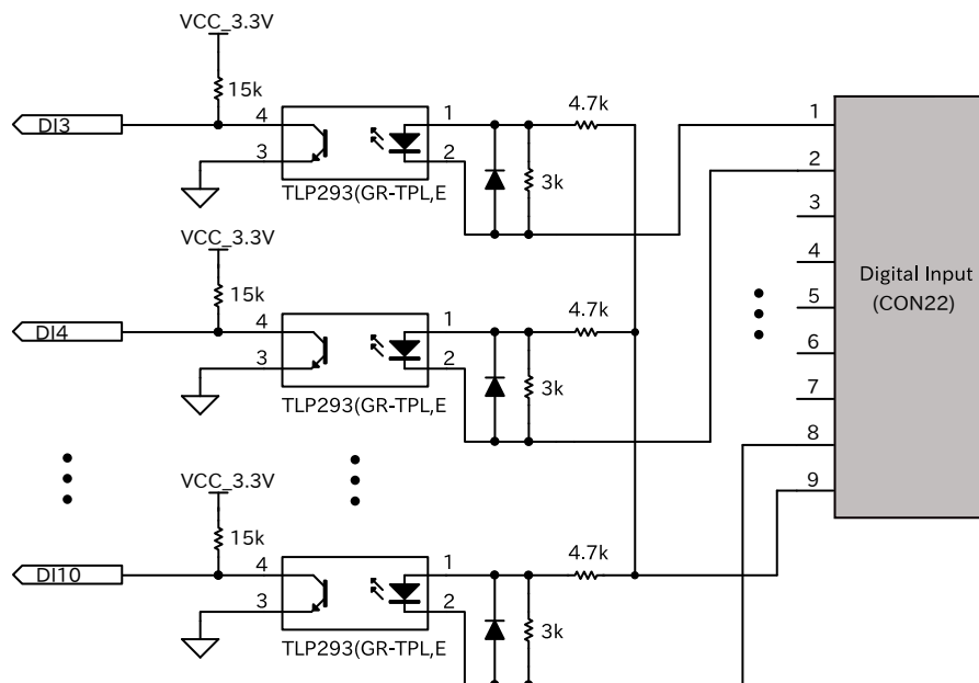
図 15.18 CON22 接点入力周辺回路
