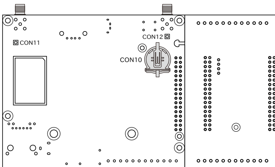
図 15.4 Armadillo-IoT ゲートウェイ A6E +Di8+Ai4 のインターフェース 裏面
