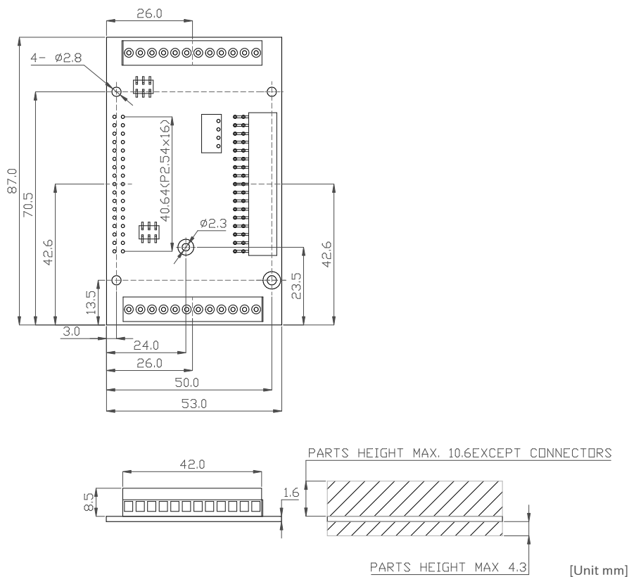
図 6.211 +Di8+Ai4 拡張基板基板形状図
