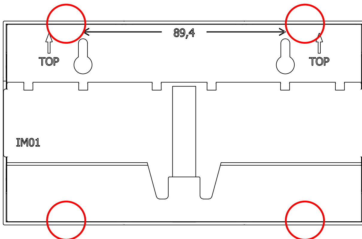
図 3.34 ケースボトムのカギ
