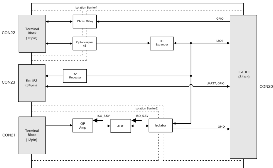
図 6.212 +Di8+Ai4 拡張基板のブロック図
