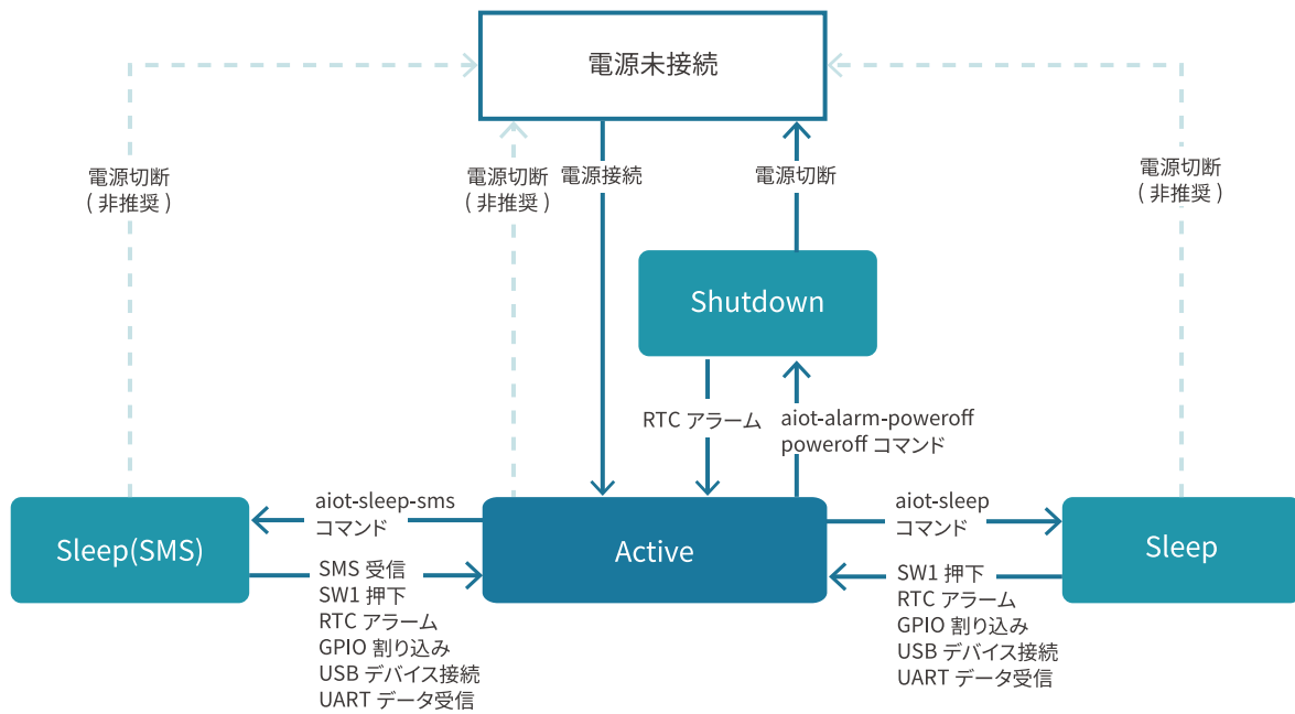
図 3.122 状態遷移図
