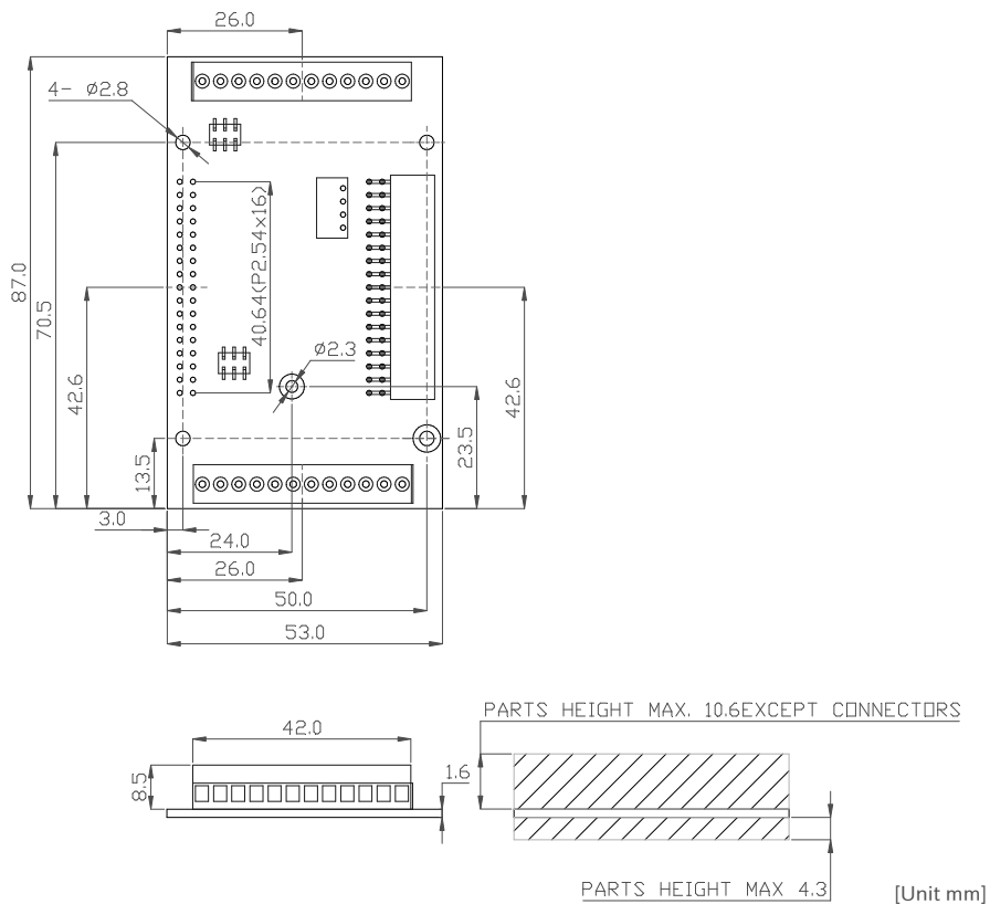
図 6.214 +Di8+Ai4 拡張基板基板形状図
