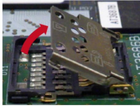
図 3.39 カバーを開ける
