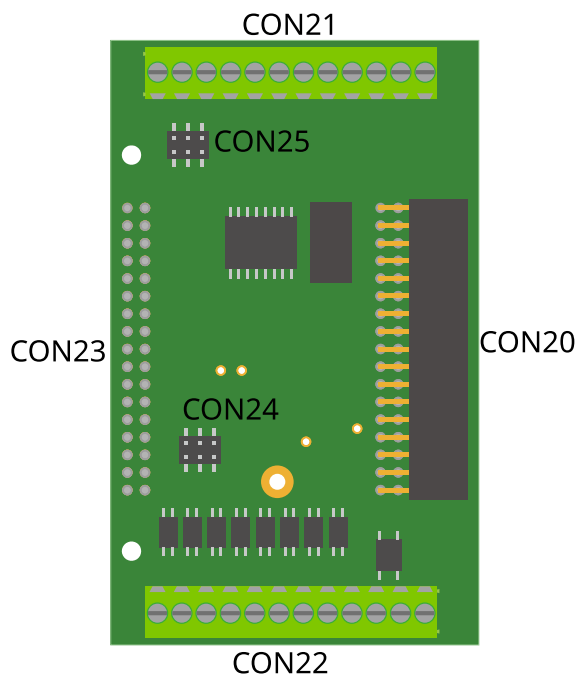
図 6.213 +Di8+Ai4 拡張基板のインターフェースレイアウト
