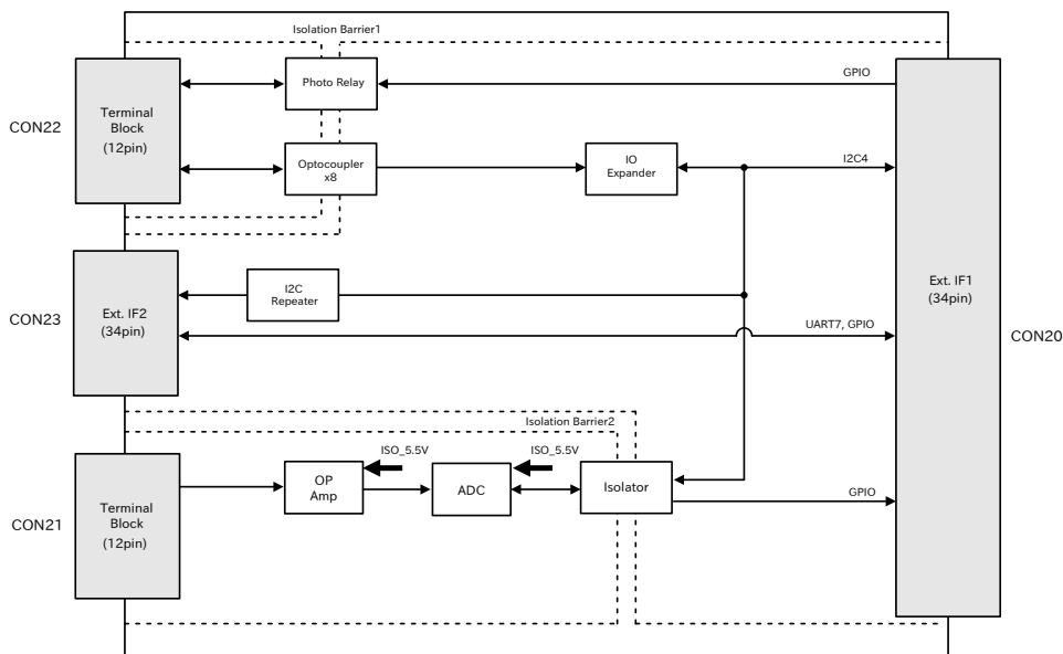
図 6.189 +Di8+Ai4 拡張基板のブロック図
