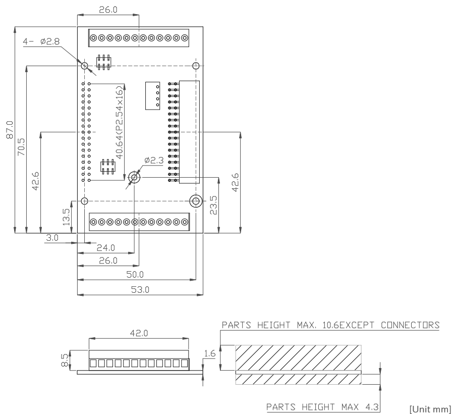
図 6.191 +Di8+Ai4 拡張基板基板形状図
