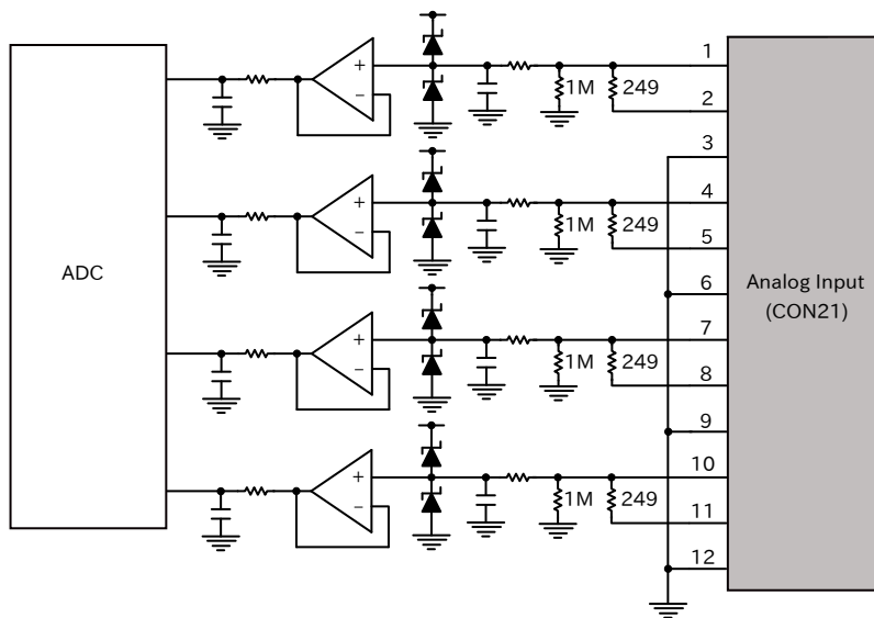
図 3.101 CON21 アナログ入力周辺回路
