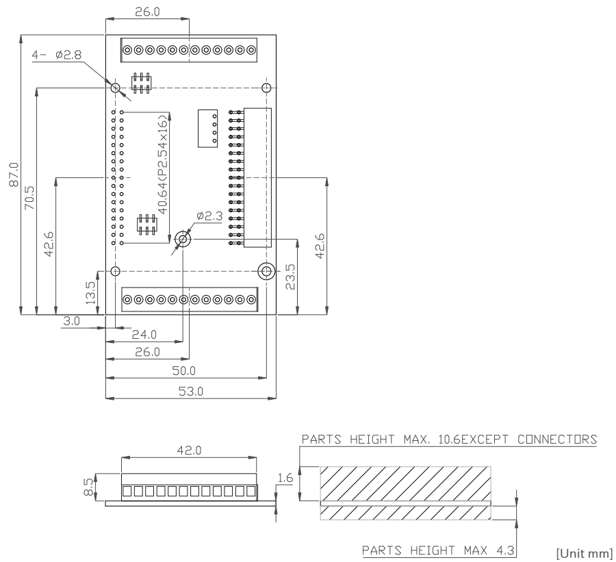
図 6.199 +Di8+Ai4 拡張基板基板形状図
