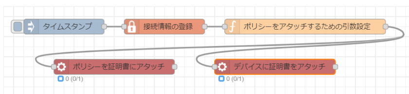
図 4.78 デバイスにポリシーをアタッチするフロー
