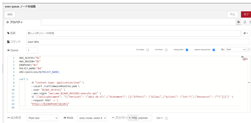
図 4.65 [新しいポリシーの作成] ノードのプロパティ内容
