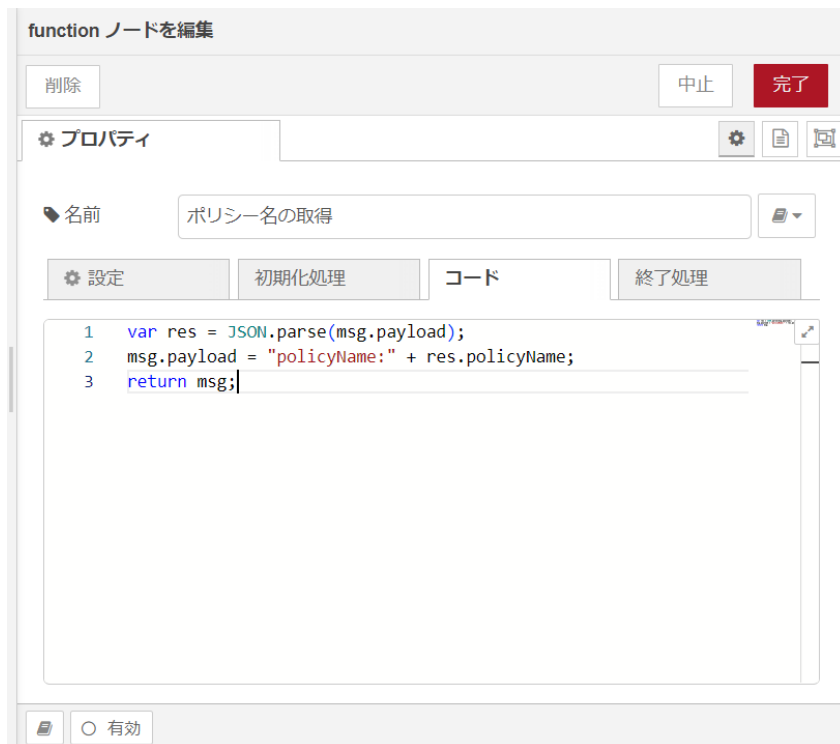
図 4.66 [ポリシー名の取得] ノードのプロパティ内容
