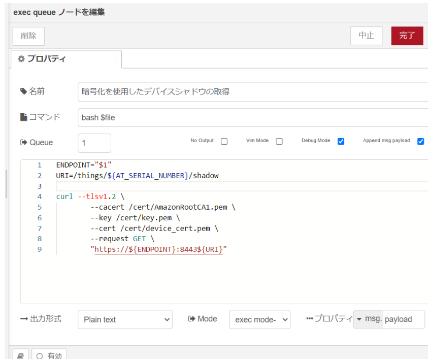
図 4.83 [暗号化を使用したデバイスシャドウの取得] ノードのプロパティ内容
