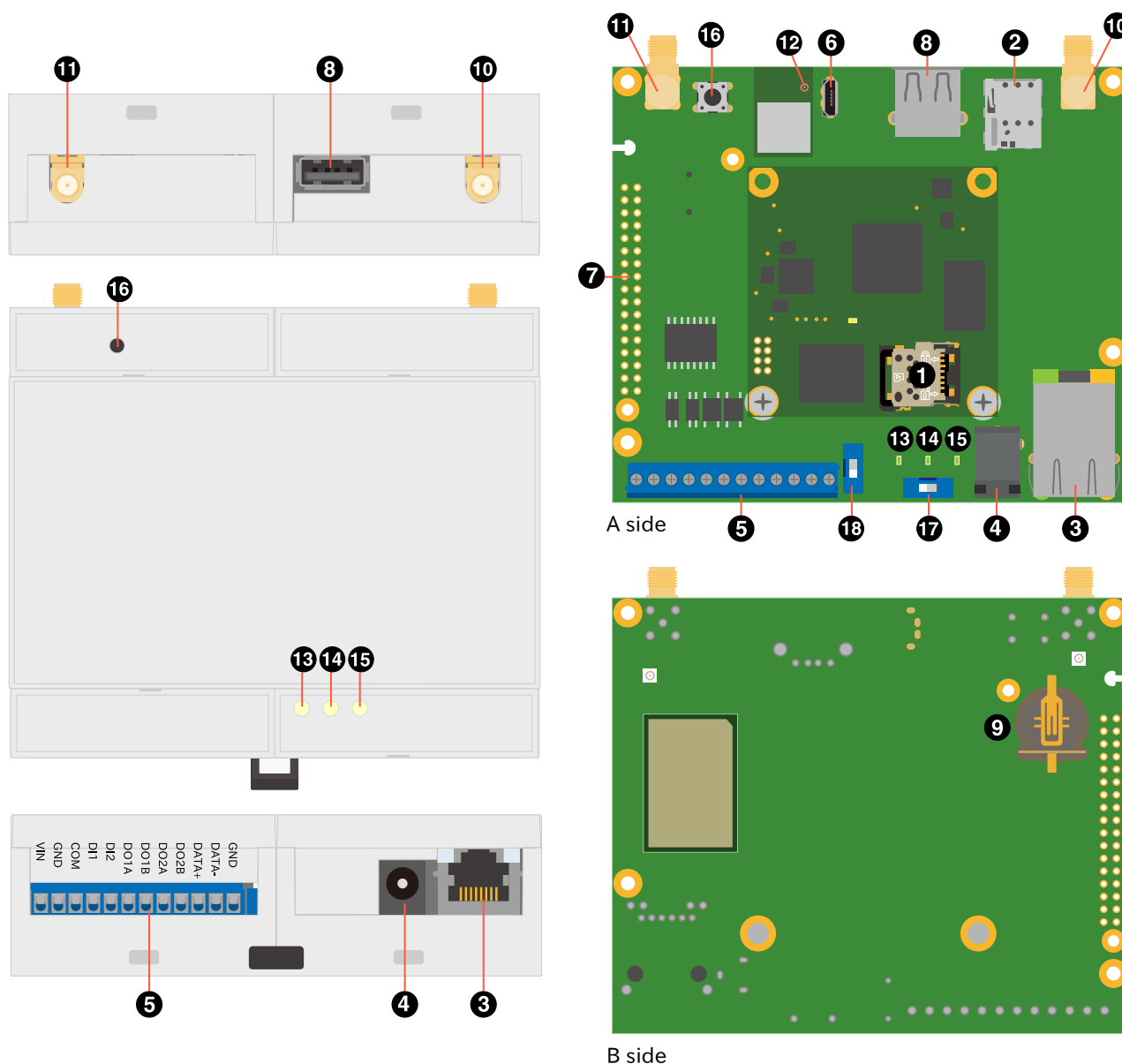
図 3.4 Armadillo-IoT ゲートウェイ A6E インターフェースレイアウト
