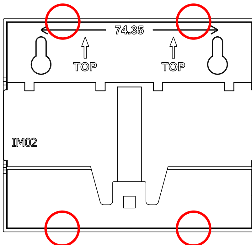
図 3.10 ケースボトムのツメ
