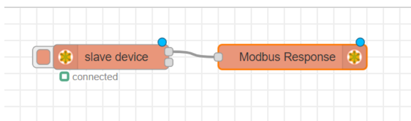
図 4.34 RS-485 を使用した Modubus RTU 読み出し用フロー
