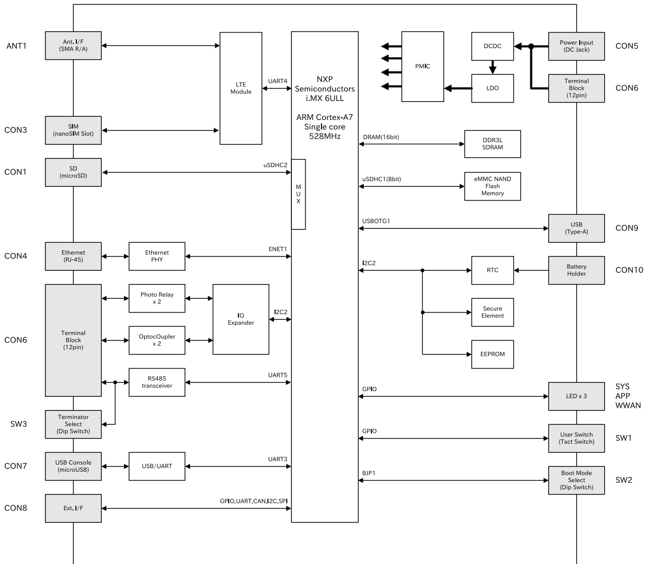
図 3.8 Armadillo-IoT ゲートウェイ A6E ブロック図
