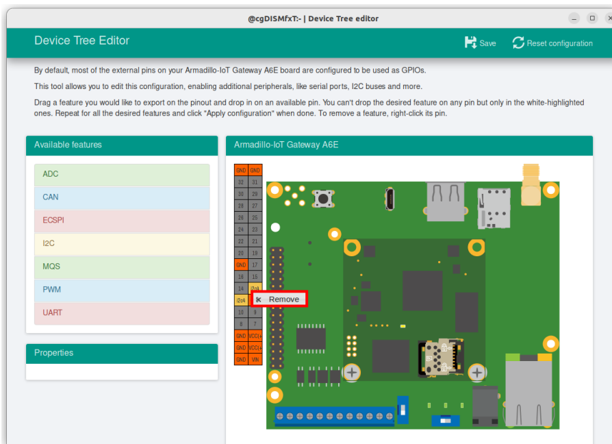
図 10.142 I2C4(SCL/SDA) の削除
