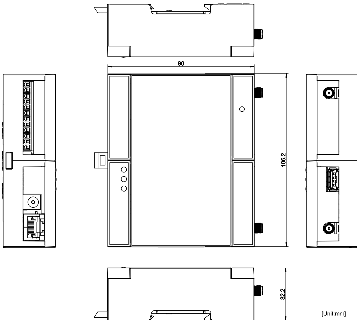
図 14.23 筐体形状
