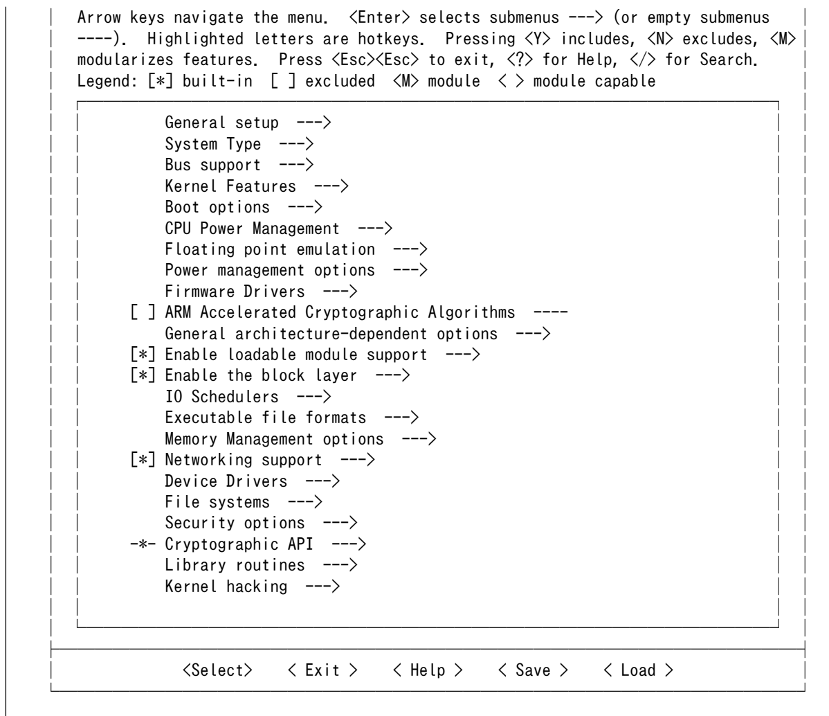
図 10.115 Linux カーネルコンフィギュレーション設定画面
