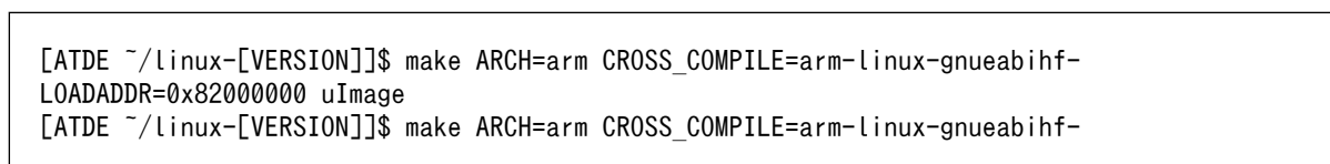
図 10.116 Linux カーネルコンフィギュレーションの変更
