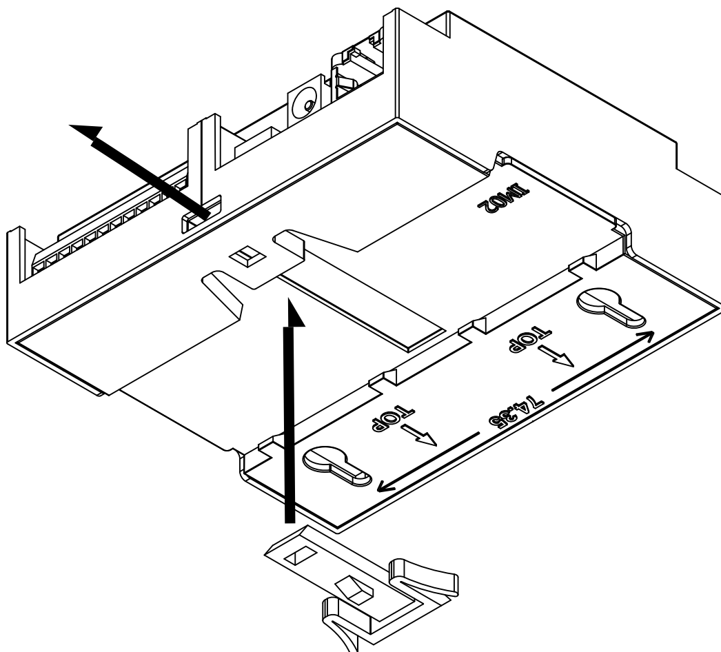
図 14.28 フック取り付け 1
