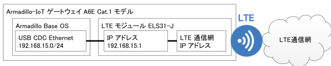
図 7.17 Cat.1 モデル (ELS31-J) LTE ネットワーク構成
