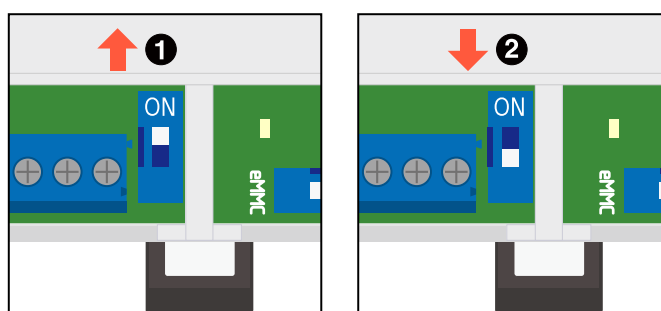
図 14.22 スイッチの状態と終端抵抗の ON/OFF
