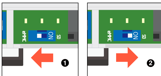
図 14.21 スイッチの状態と起動デバイス
