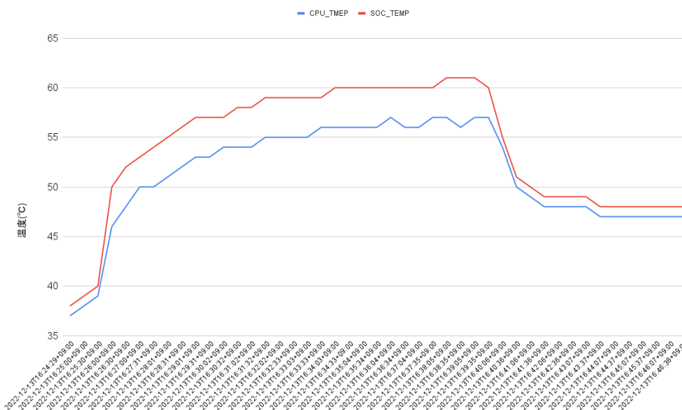
図 10.161 Armadillo-IoT ゲートウェイ G4 で取得した温度のグラフ
