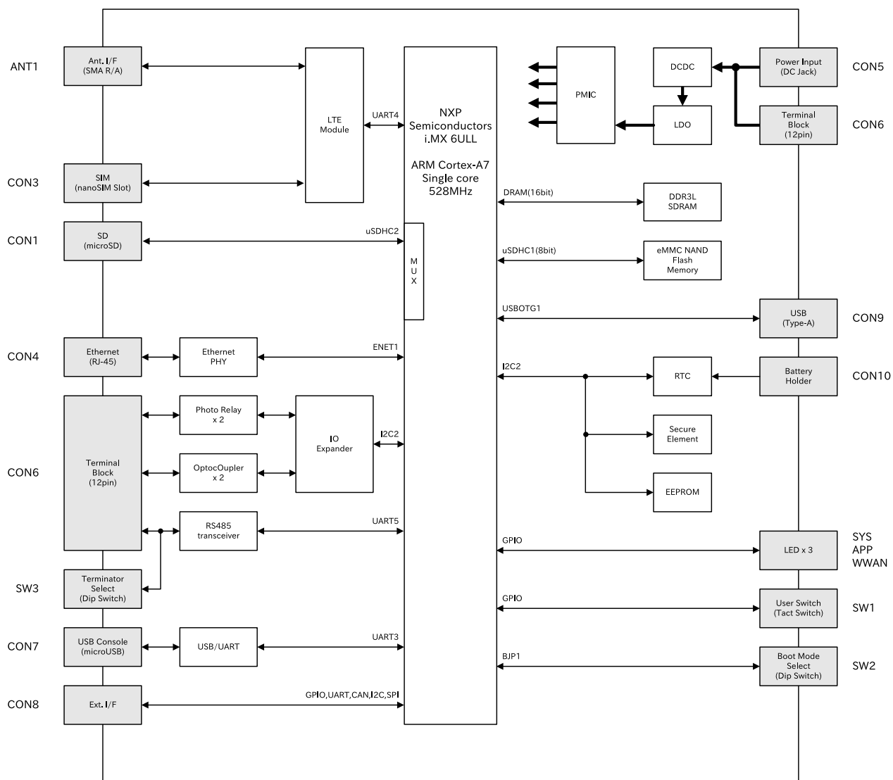
図 3.10 Armadillo-IoT ゲートウェイ A6E ブロック図
