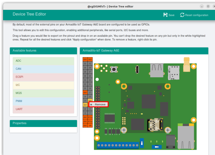
図 10.143 I2C4(SCL/SDA) の削除
