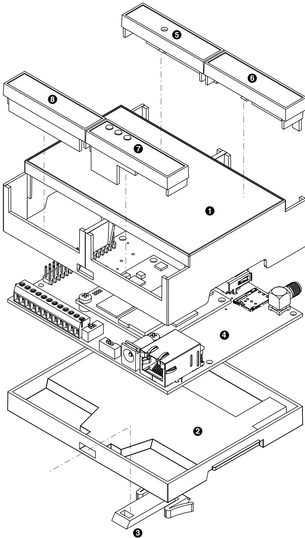
図 14.27 ケースモデル展開図
