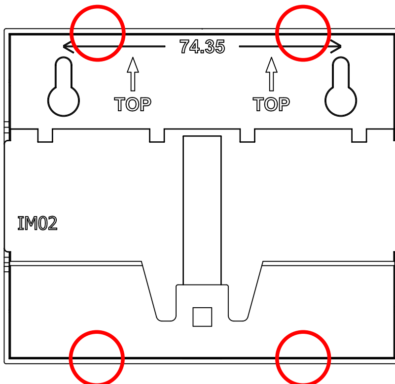
図 14.31 ケースボトムのツメ
