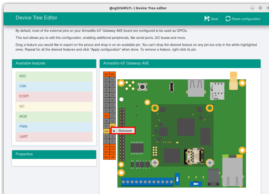
図 10.169 I2C4(SCL/SDA) の削除
