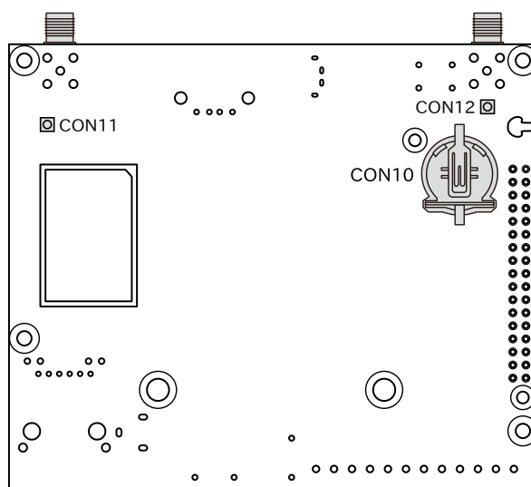
図 14.4 Armadillo-IoT ゲートウェイ A6E のインターフェース 裏面
