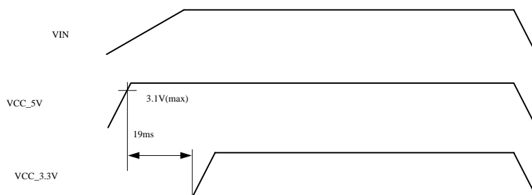
図 14.2 電源シーケンス
