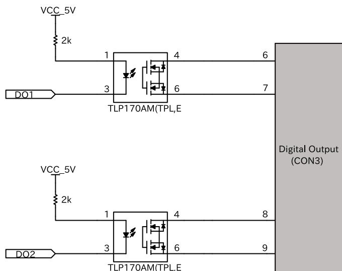
図 14.14 CON6 接点出力周辺回路
