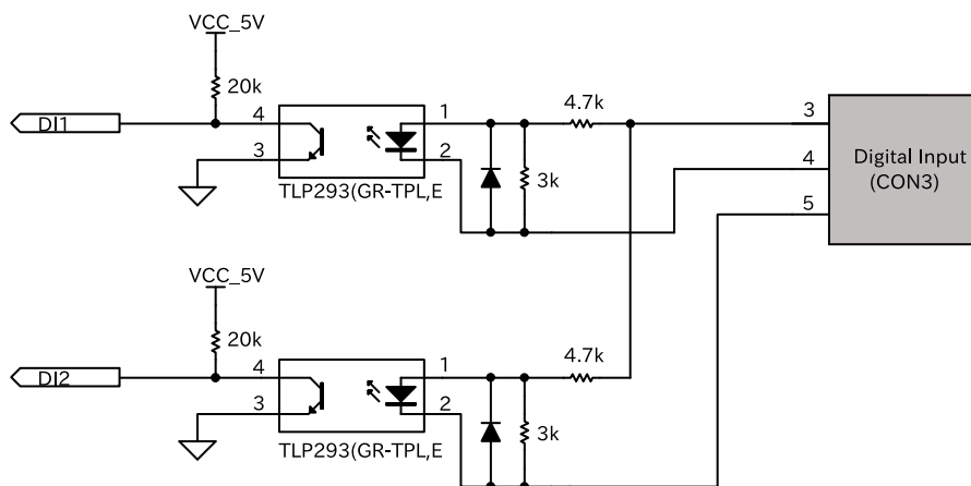
図 14.13 CON6 接点入力周辺回路
