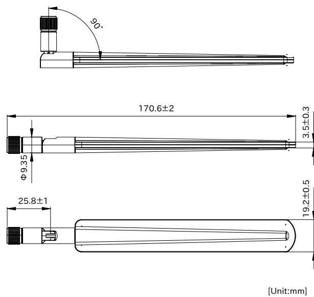
図 14.29 LTE アンテナ形状図
