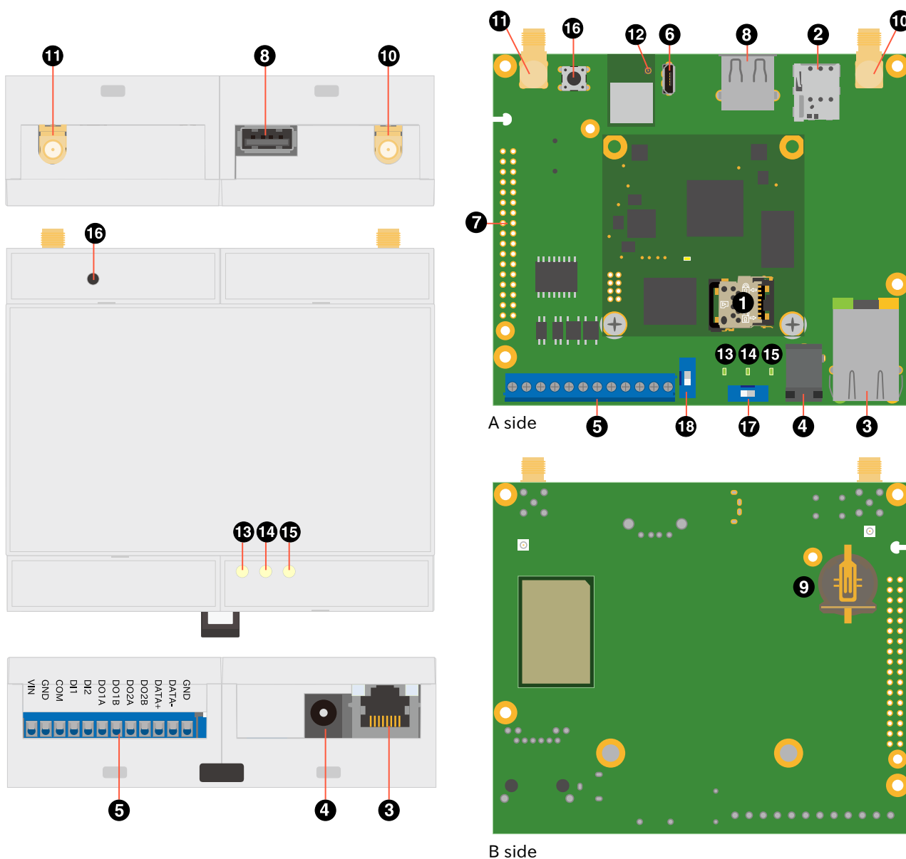
図 3.10 Armadillo-IoT ゲートウェイ A6E の外観
