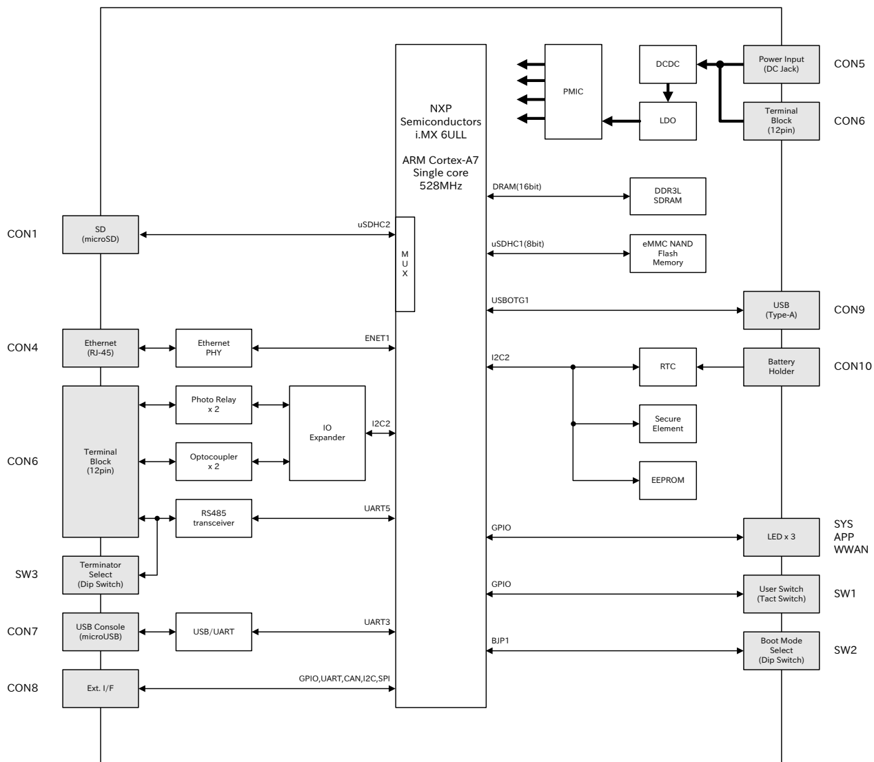
図 3.15 ブロック図(AG6201-C00Z,AG6201-U00Z)
