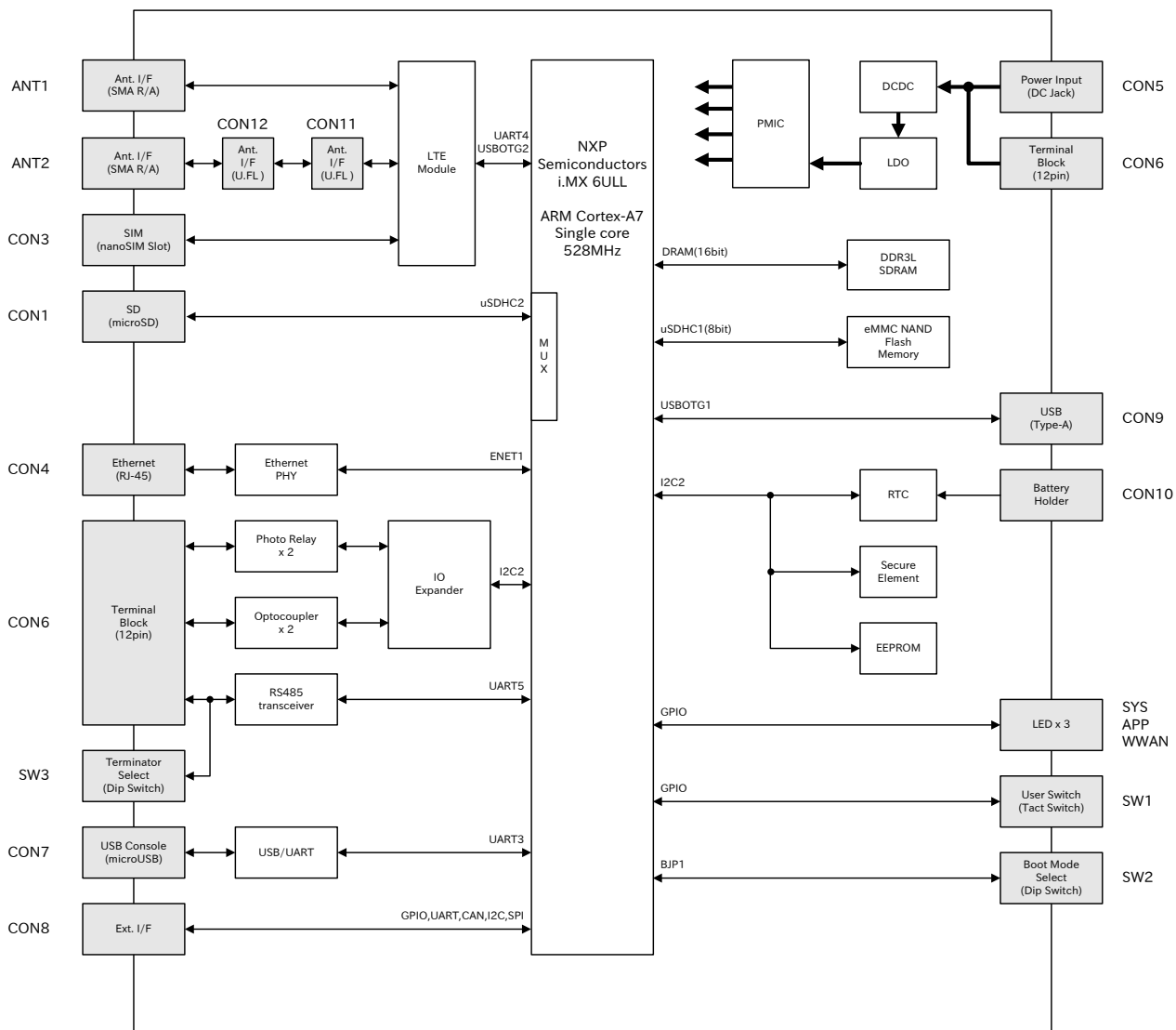
図 3.12 ブロック図(AG6261-C01Z,AG6261-U01Z,AG6261-U00Z)
