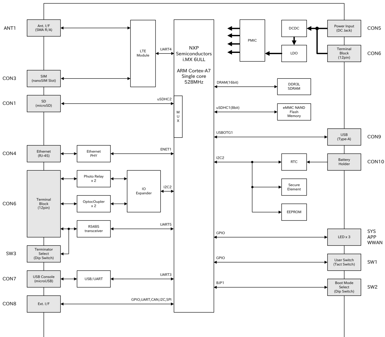
図 3.13 ブロック図(AG6221-C01D0,AG6221-C01Z,AG6221-U01Z,AG6221-U00Z)
