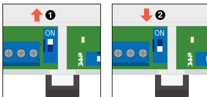
図 14.24 スイッチの状態と終端抵抗の ON/OFF
