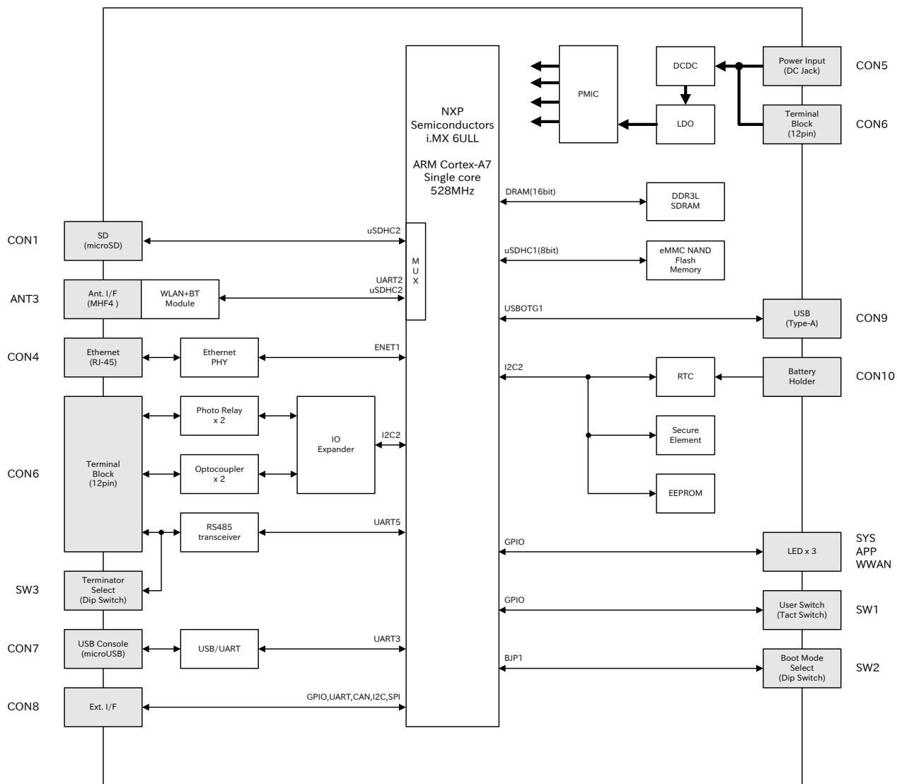
図 3.14 ブロック図(AG6211-C02D0,AG6211-C02Z,AG6211C00Z,AG6211-U02Z,AG6211-U00Z)
