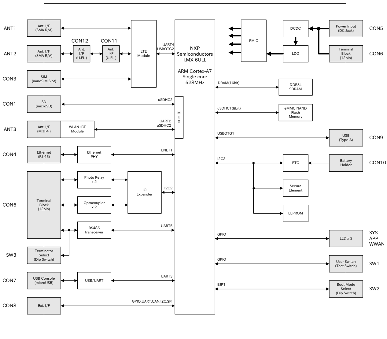
図 3.11 ブロック図(AG6271-C03D0,AG6271-C03Z,AG6271-U03Z,AG6271-U00Z)
