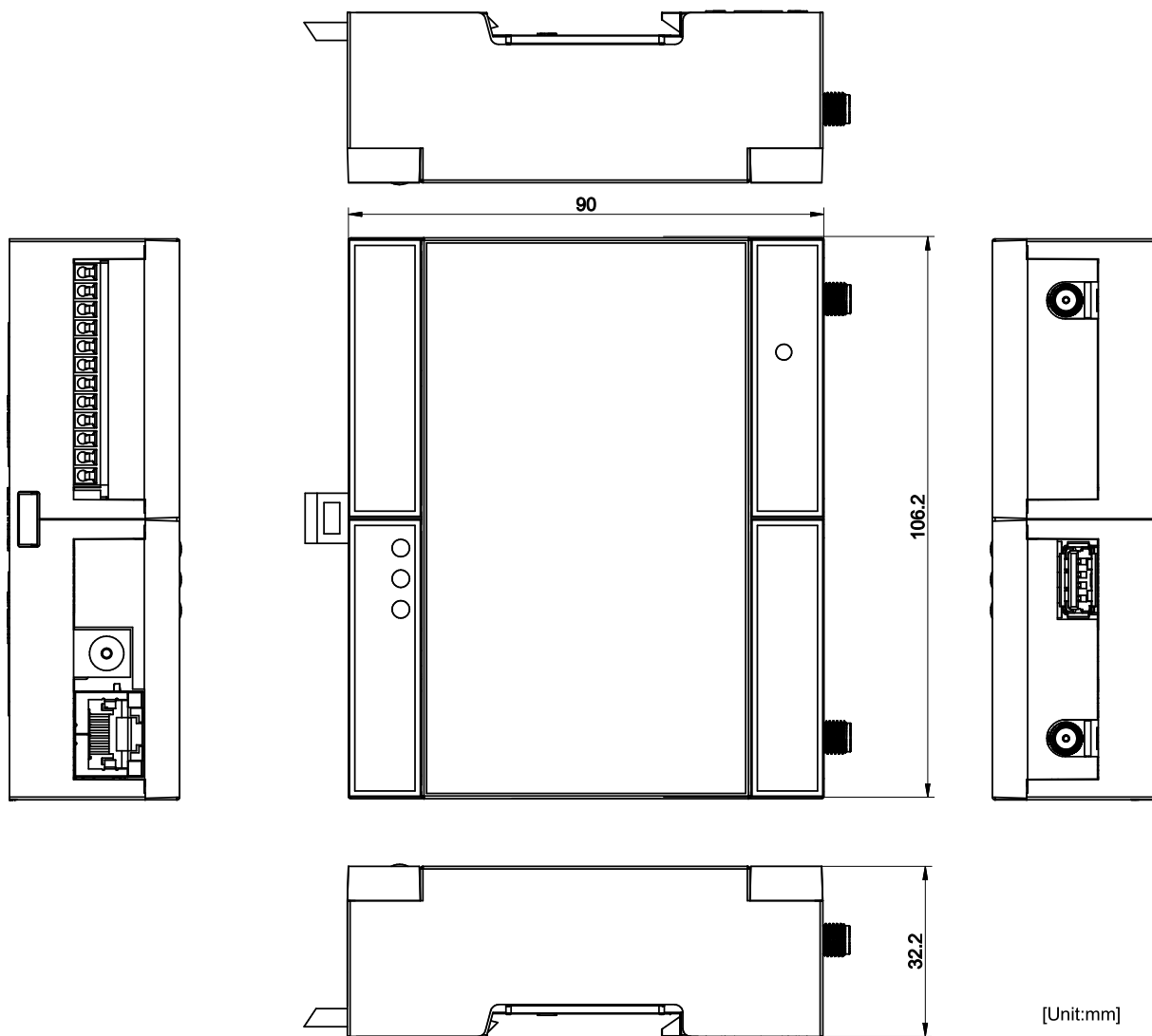
図 14.25 筐体形状
