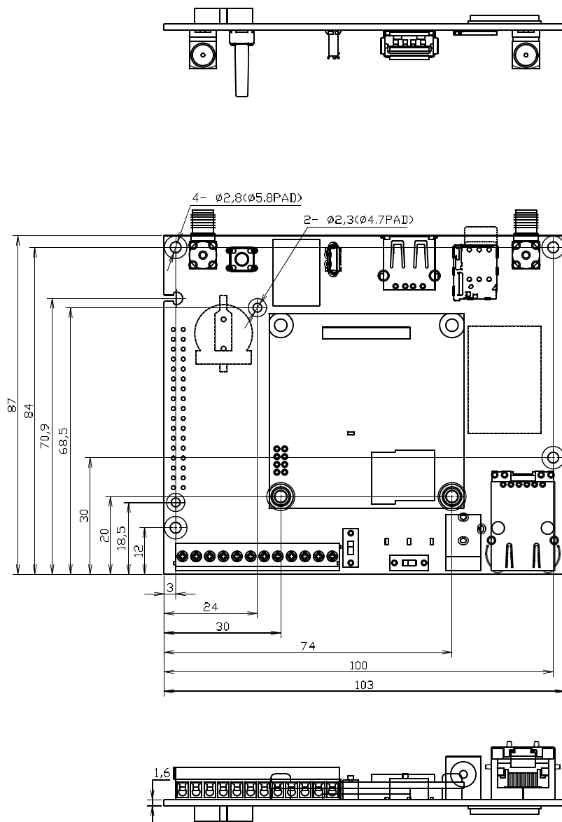
図 15.26 基板形状および固定穴寸法
