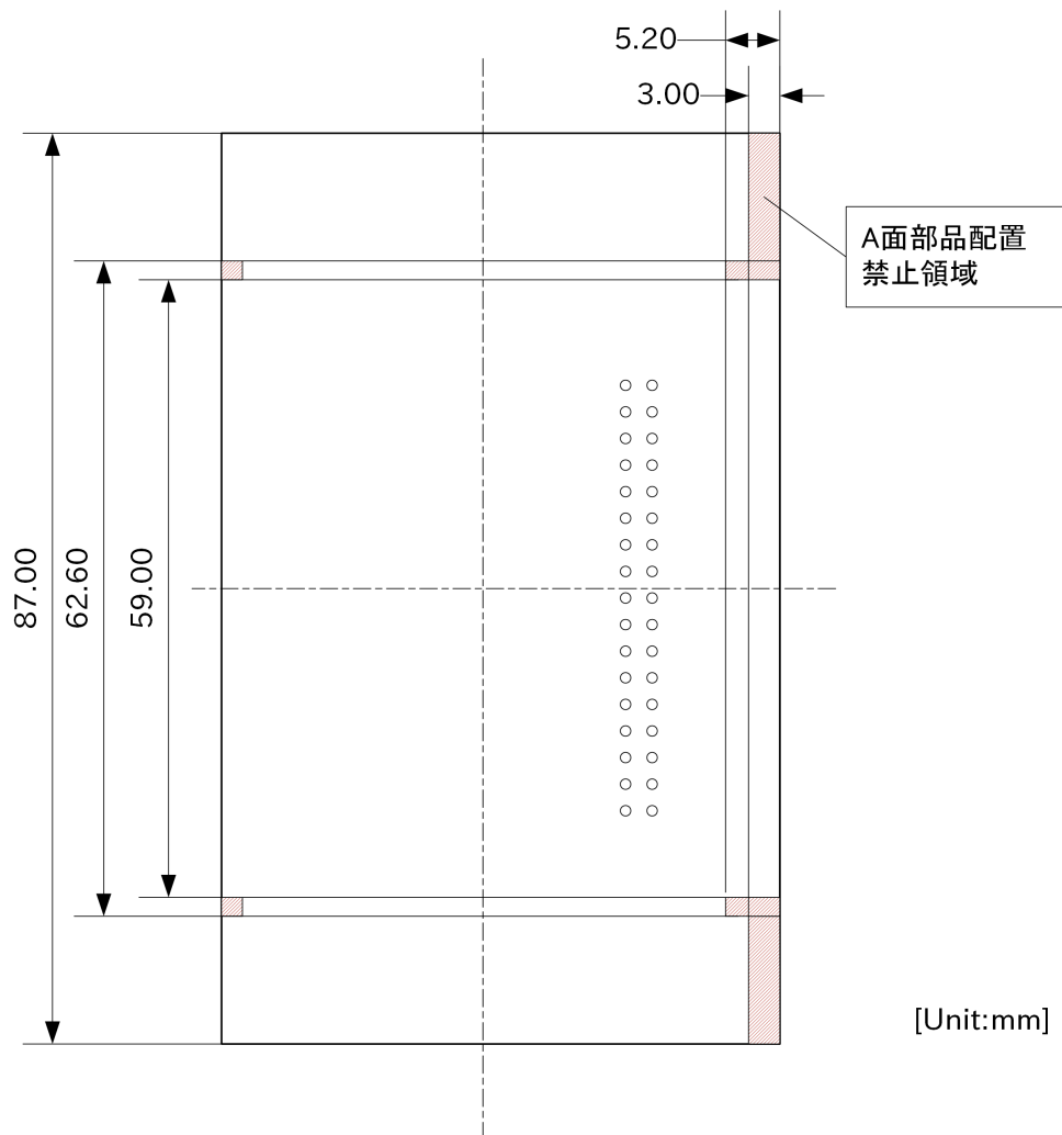
図 15.40 水平方向に拡張する場合の部品搭載制限(A 面側)
