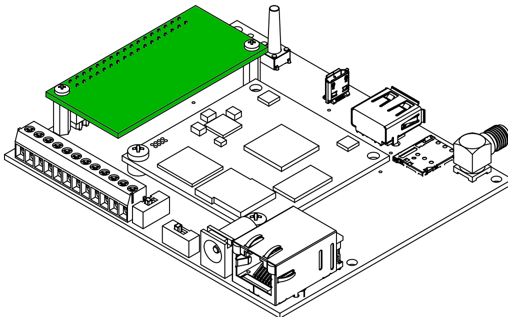
図 15.36 垂直方向に拡張基板を配置した場合の接続例
