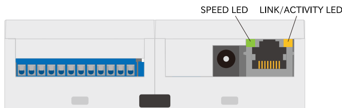
図 15.11 CON4 LAN LED
