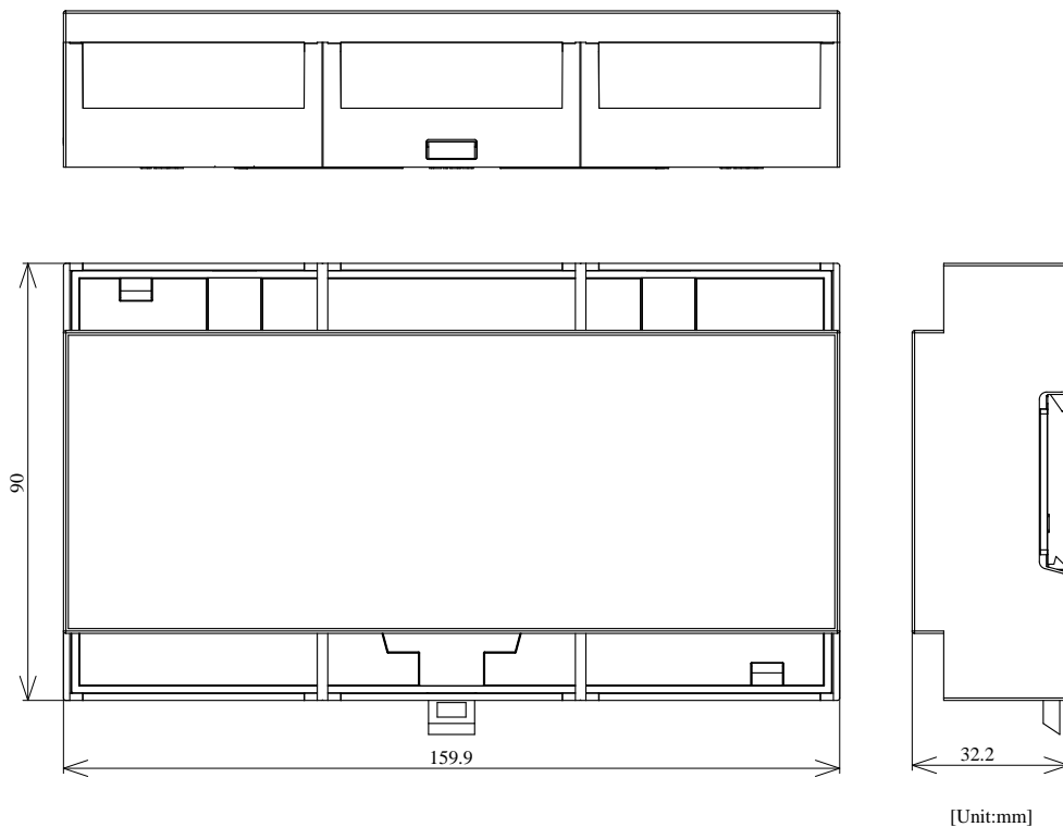
図 15.42 拡張ケース外形
