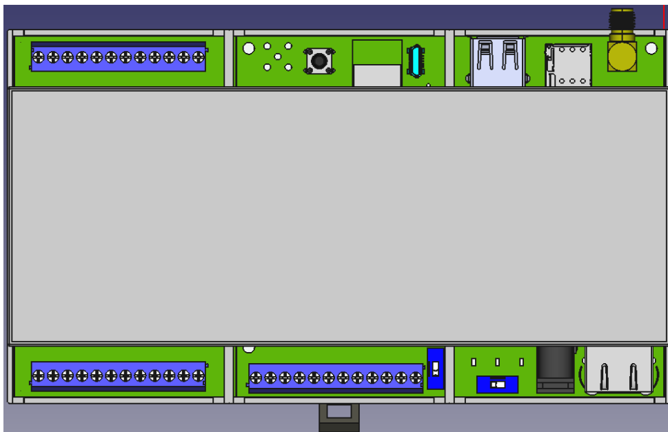
図 15.38 拡張ケース搭載例
