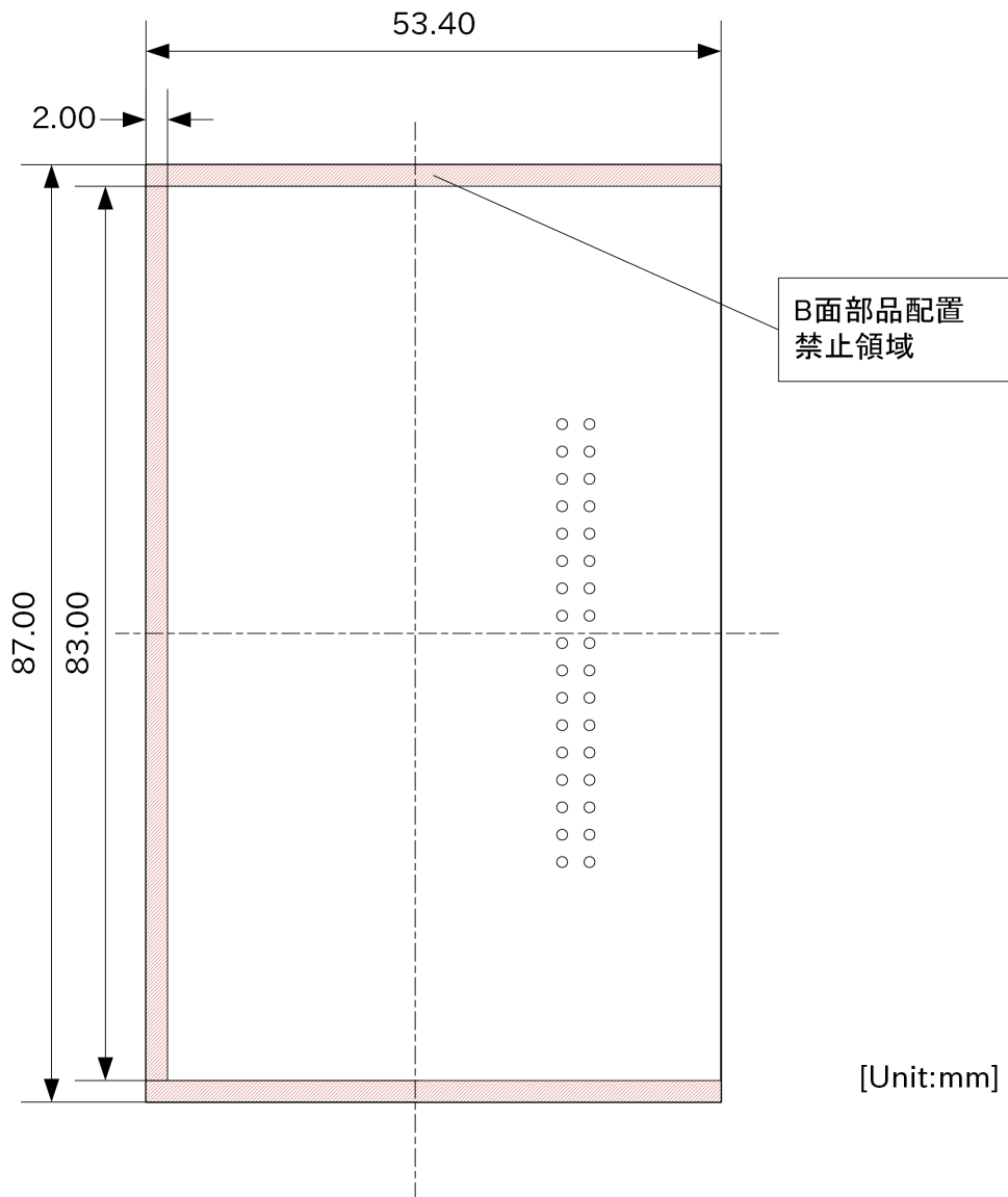
図 15.41 水平方向に拡張する場合の部品搭載制限(B 面側)
