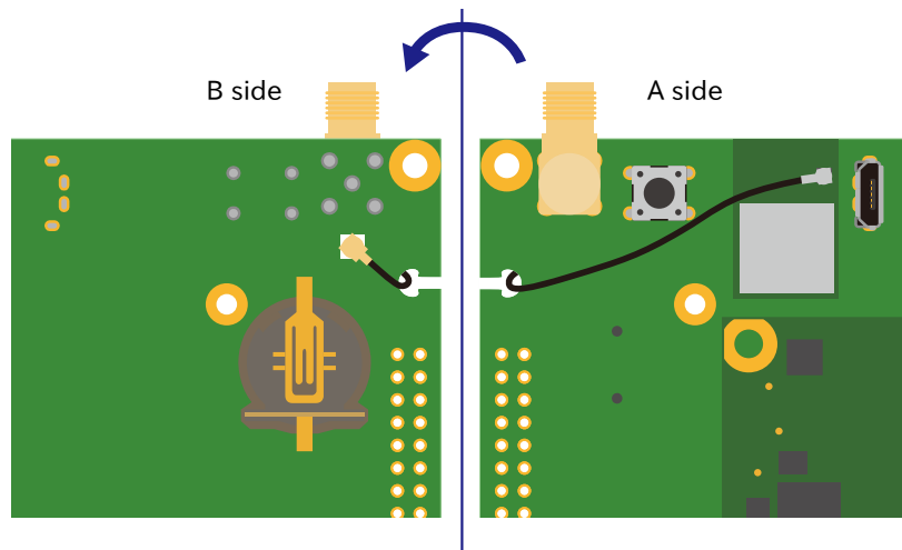
図 15.19 ANT2 カスタマイズ例：同軸ケーブル接続図
