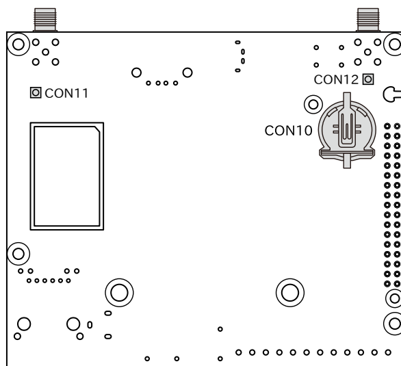
図 15.4 Armadillo-IoT ゲートウェイ A6E のインターフェース 裏面
