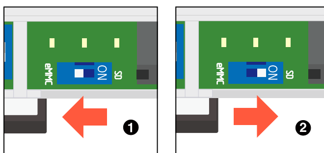
図 15.23 スイッチの状態と起動デバイス
