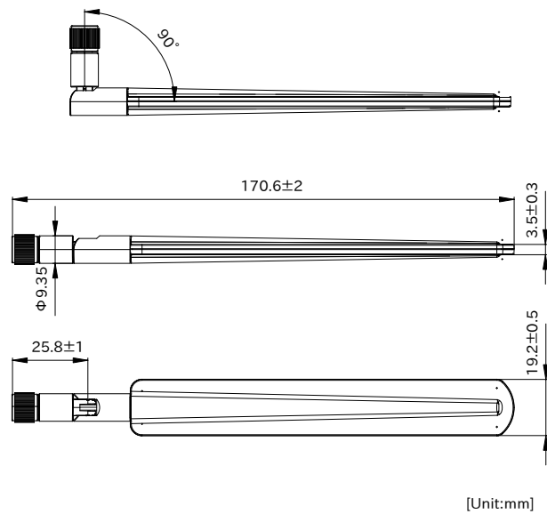
図 15.29 LTE アンテナ形状図
