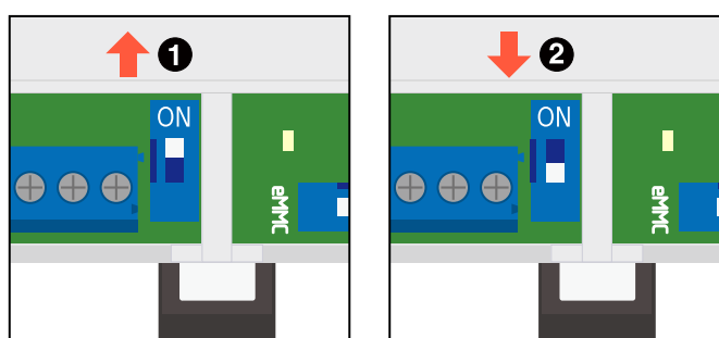
図 15.24 スイッチの状態と終端抵抗の ON/OFF
