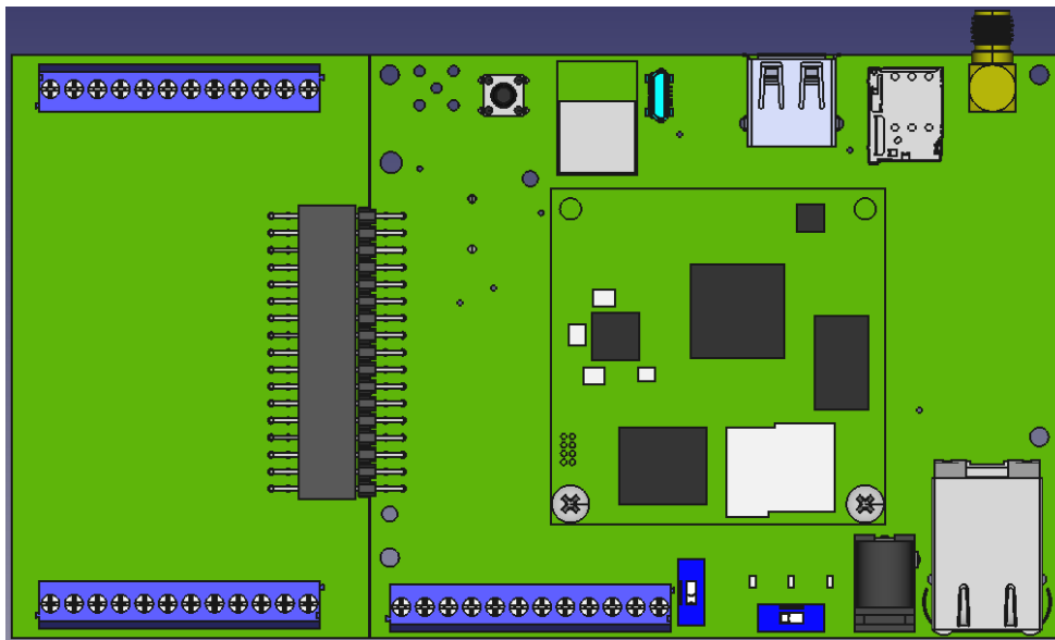
図 15.37 水平方向に拡張基板を配置した場合の接続例
