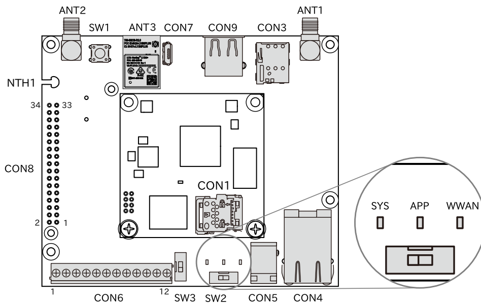
図 15.3 Armadillo-IoT ゲートウェイ A6E のインターフェース 表面
