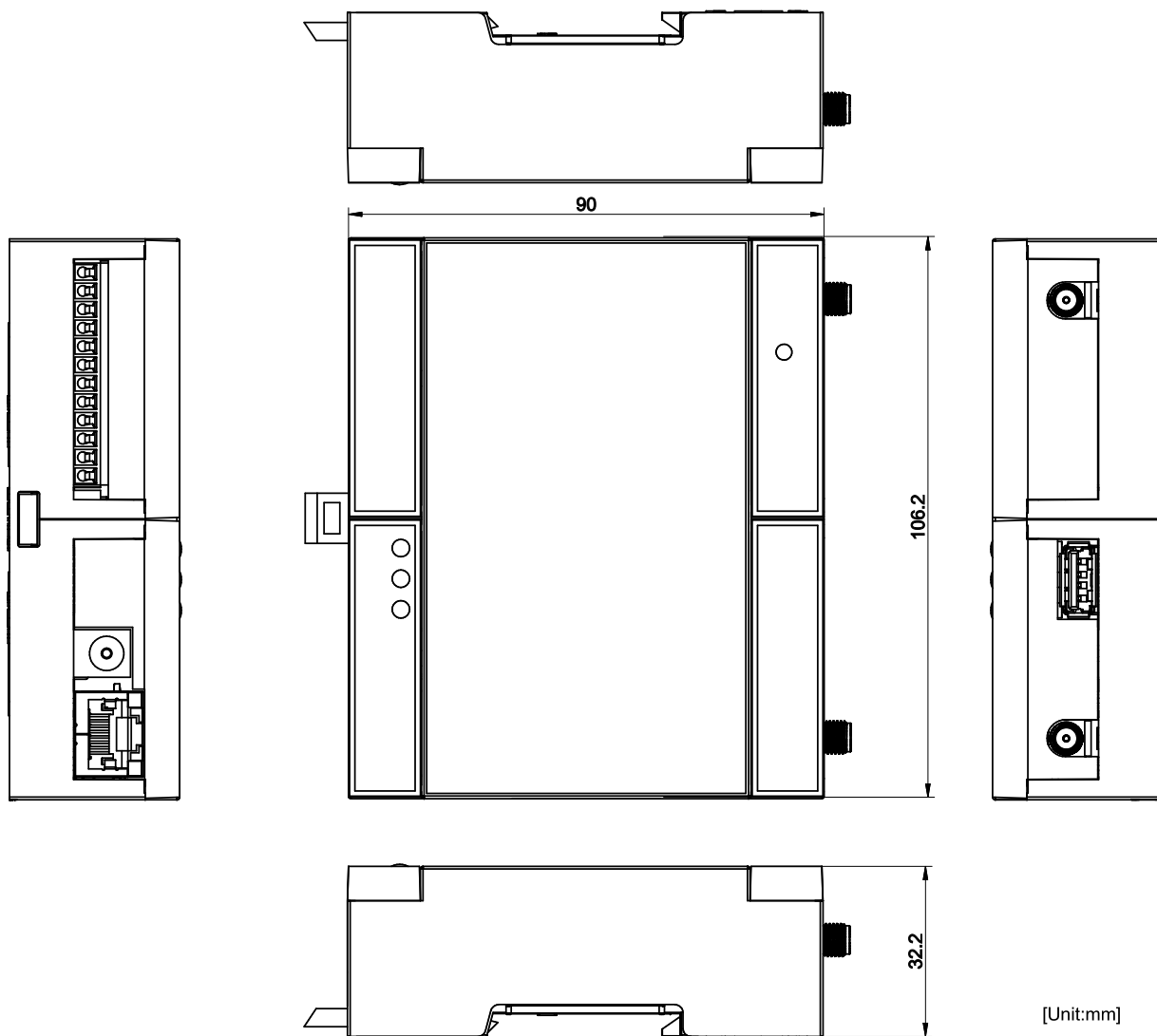
図 15.25 筐体形状
