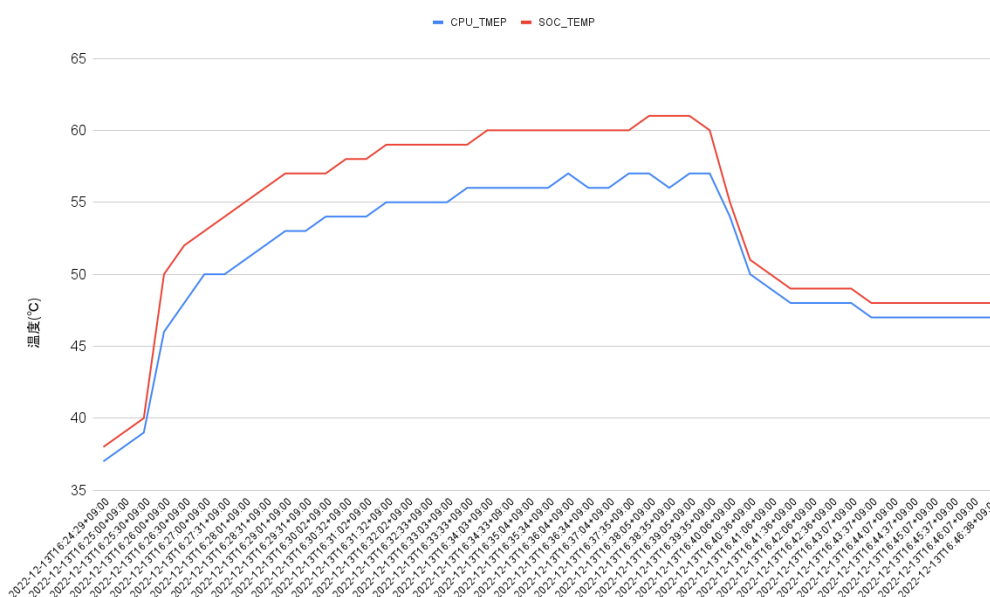
図 11.189 Armadillo-IoT ゲートウェイ G4 で取得した温度のグラフ
