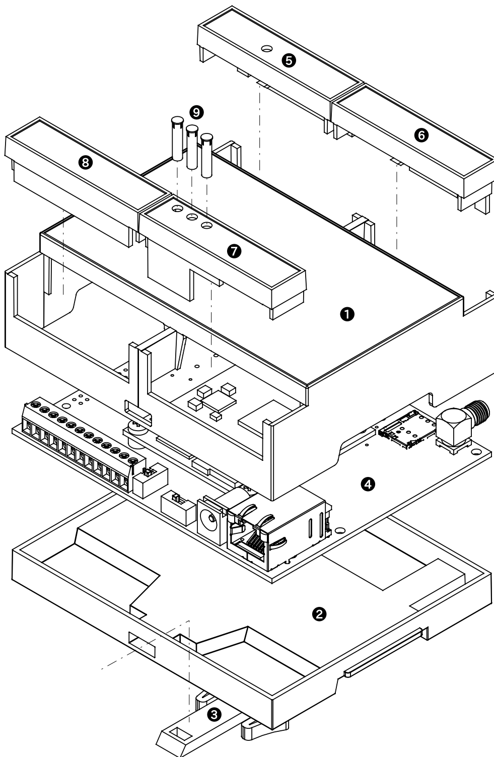
図 15.30 ケースモデル展開図
