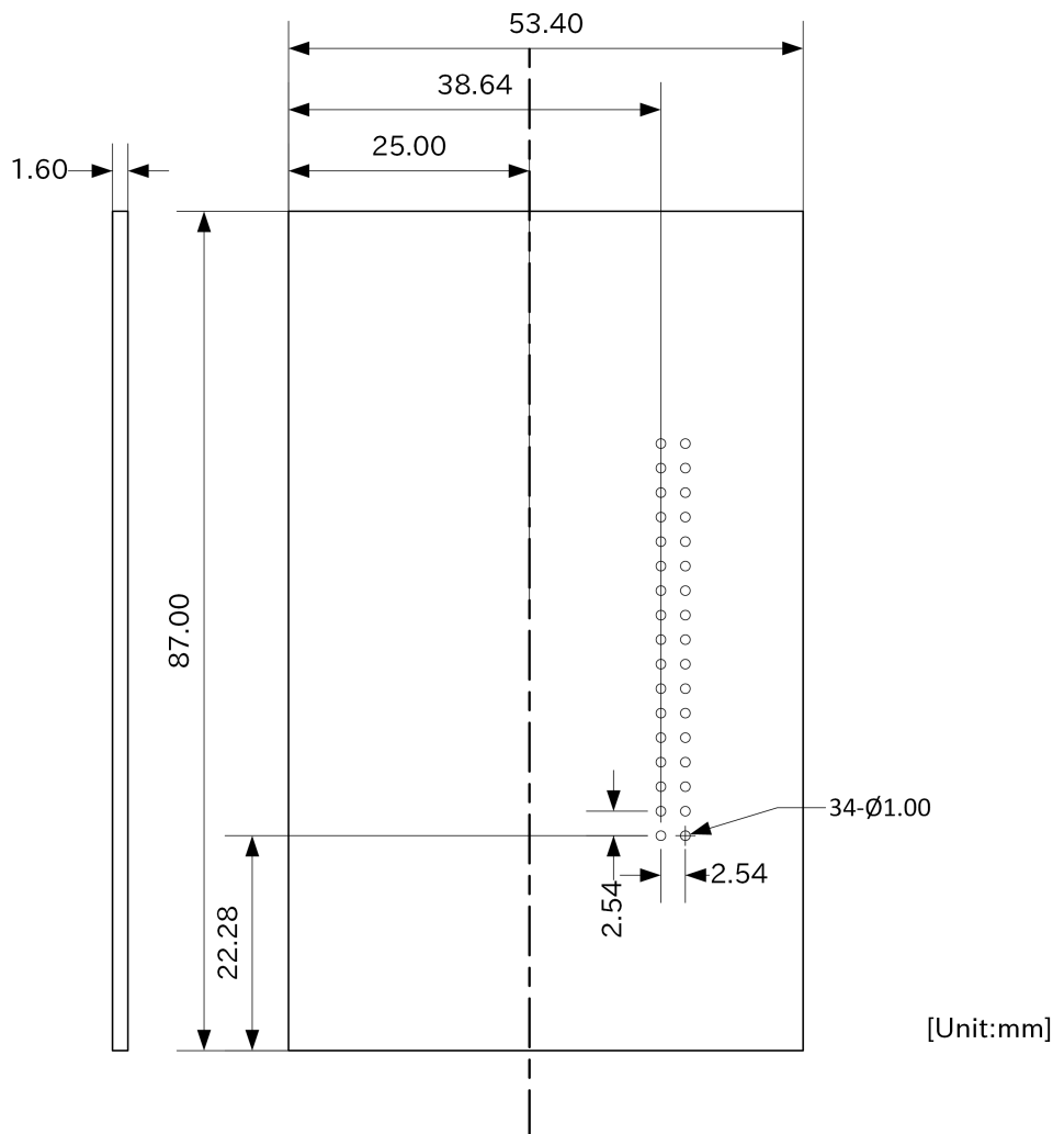
図 15.39 水平方向に拡張する場合の基板形状図
