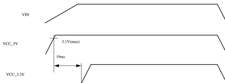
図 6.202 電源シーケンス
