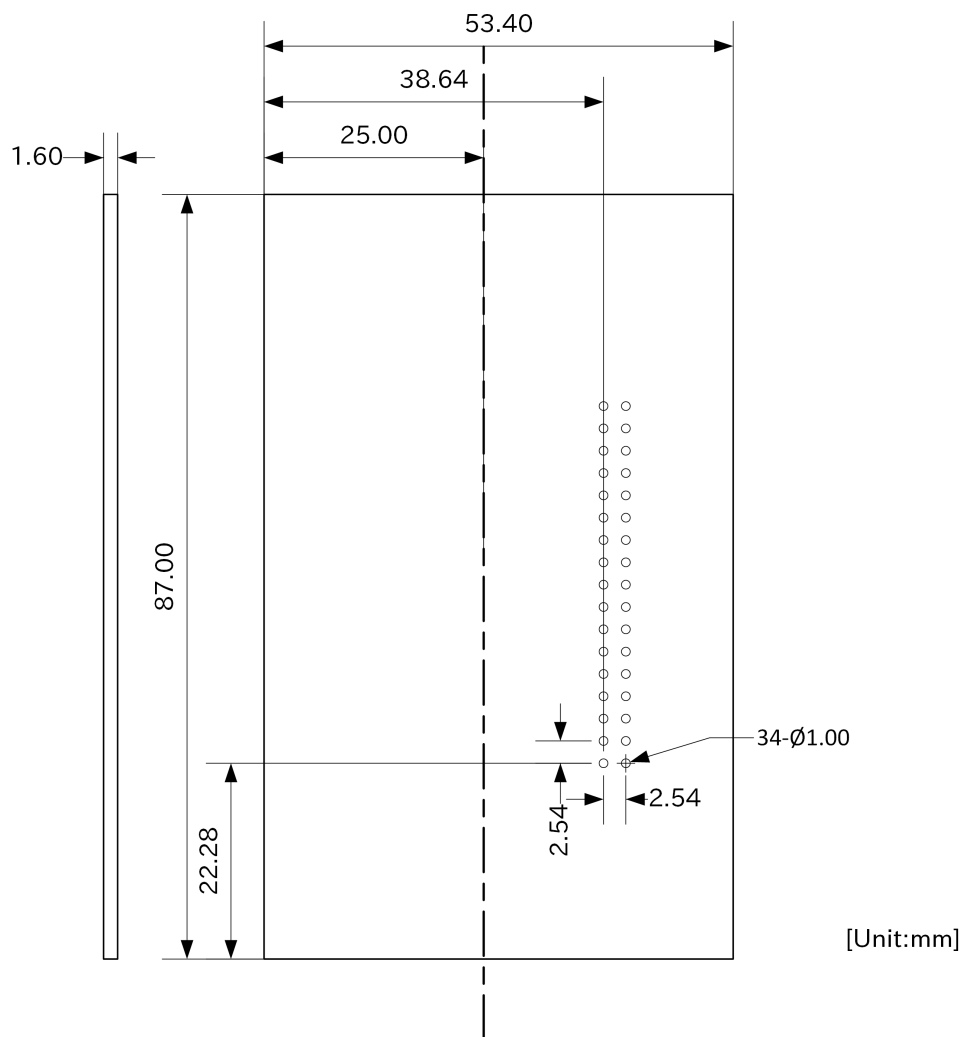
図 3.27 水平方向に拡張する場合の基板形状図
