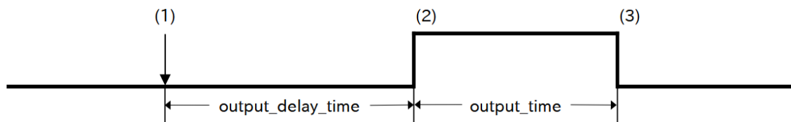
図 3.130 DO の出力タイミング
