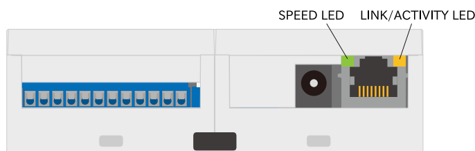
図 3.46 CON4 LAN LED
