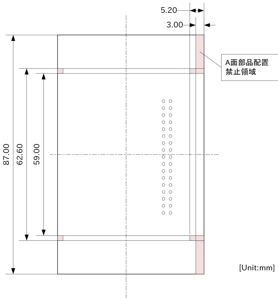
図 3.28 水平方向に拡張する場合の部品搭載制限(A 面側)
