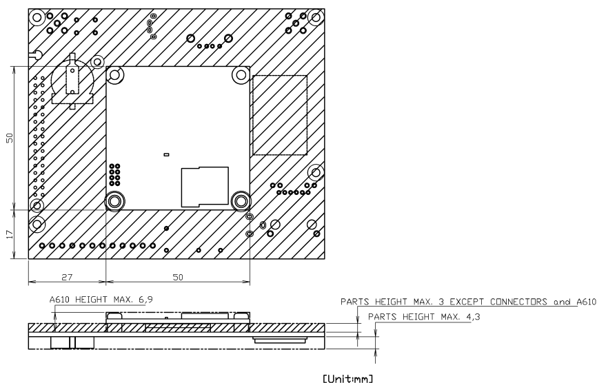
図 6.206 部品高さ
