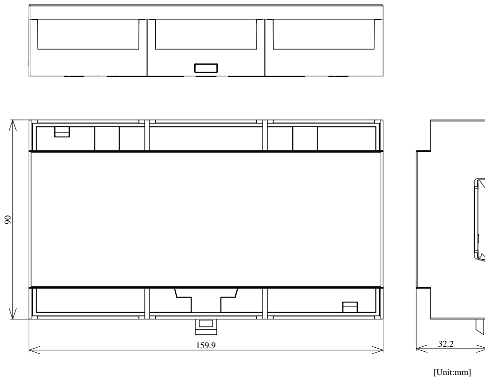
図 3.30 拡張ケース外形
