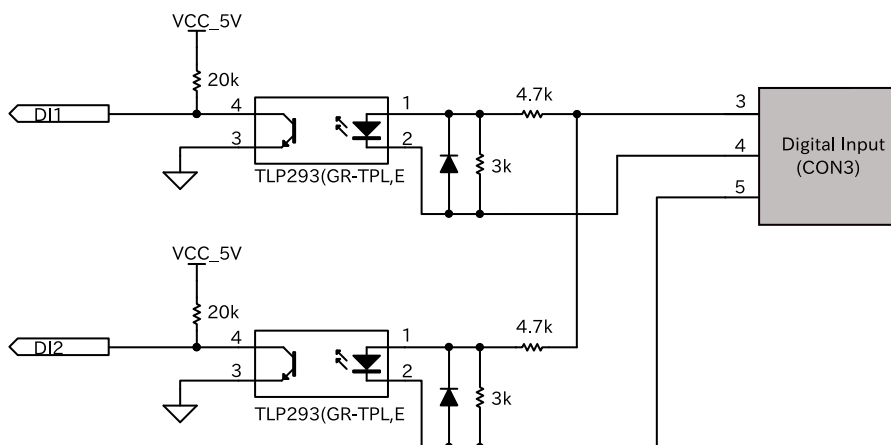
図 3.67 CON6 接点入力周辺回路
