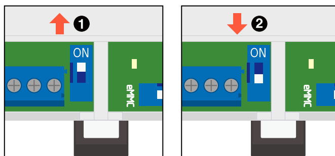
図 3.77 スwitchの状態と終端抵抗の ON/OFF
