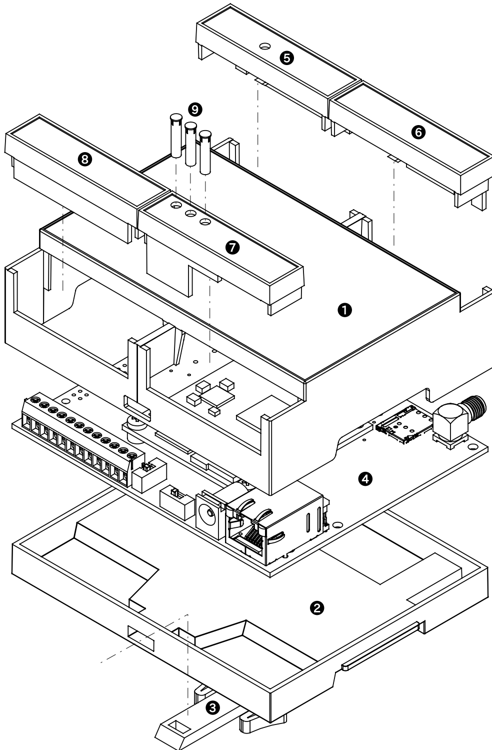
図 3.32 ケースモデル展開図
