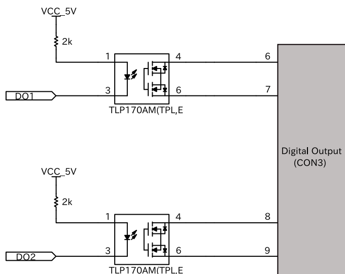
図 3.71 CON6 接点出力周辺回路
