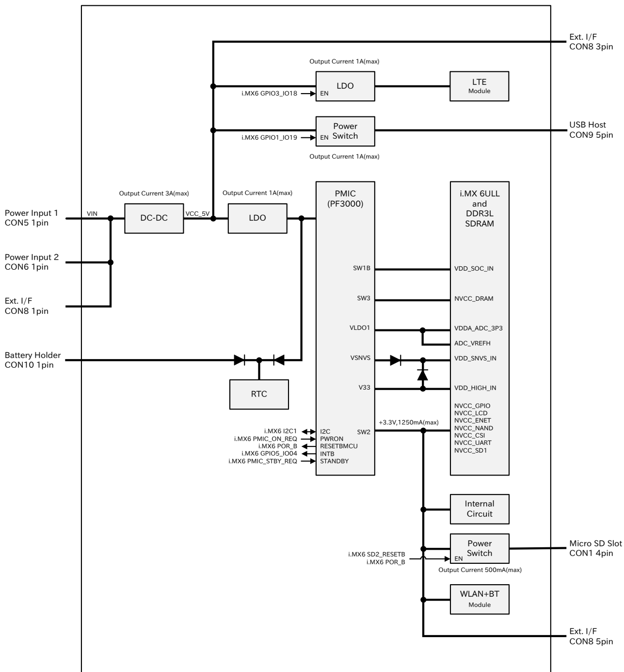
図 6.201 電源回路の構成
