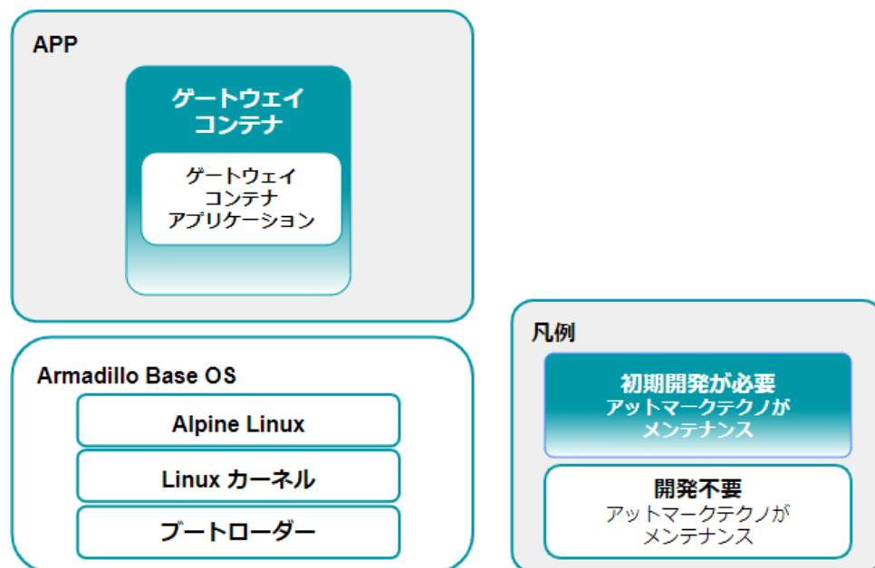
図 3.104 ゲートウェイコンテナ使用時、開発者が開発するもの、開発しなくていいもの
