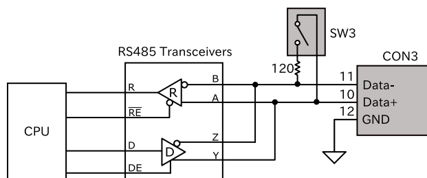
図 3.76 CON6 RS485 トランシーバ周辺回路
