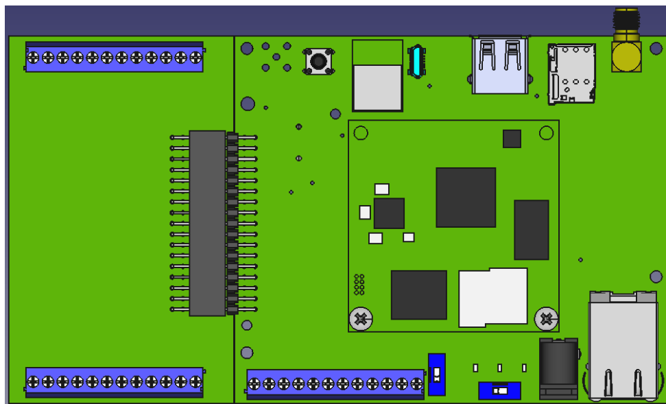
図 3.25 水平方向に拡張基板を配置した場合の接続例
