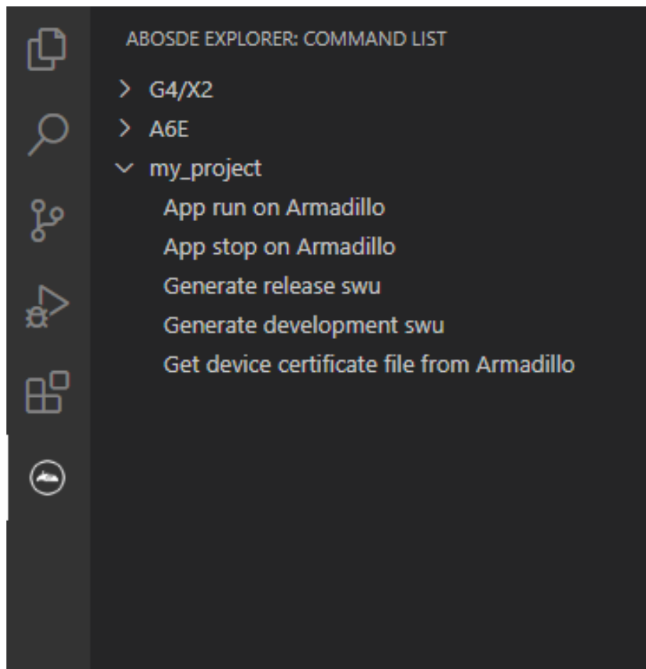
図 3.127 タスク一覧
