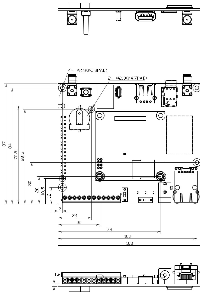
図 6.199 基板形状および固定穴寸法
