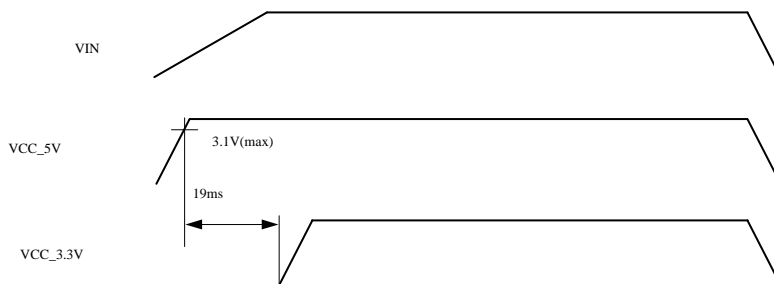
図 6.197 電源シーケンス
