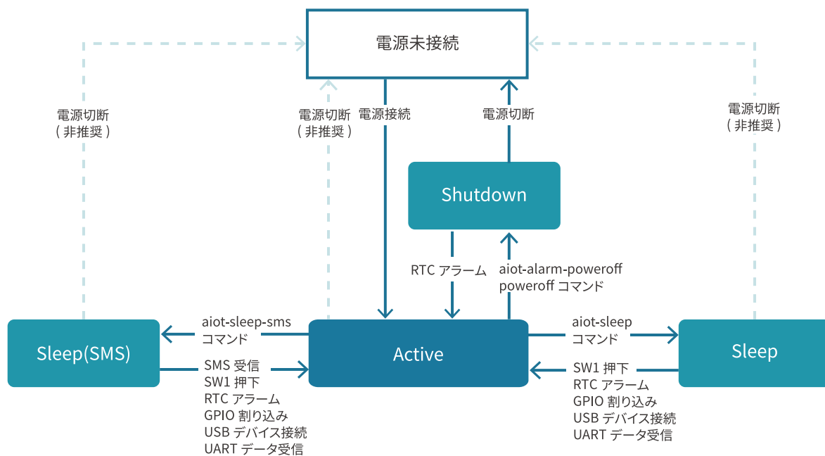
図 3.105 状態遷移図
