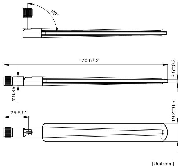
図 6.202 LTE アンテナ形状図
