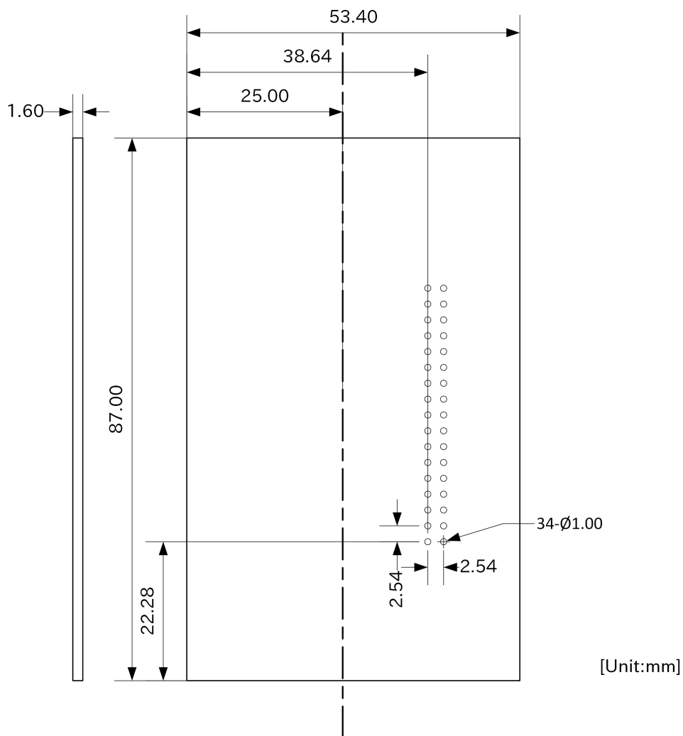
図 3.27 水平方向に拡張する場合の基板形状図
