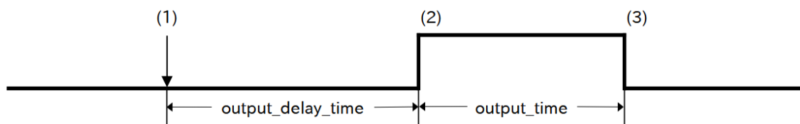
図 3.130 DO の出力タイミング
