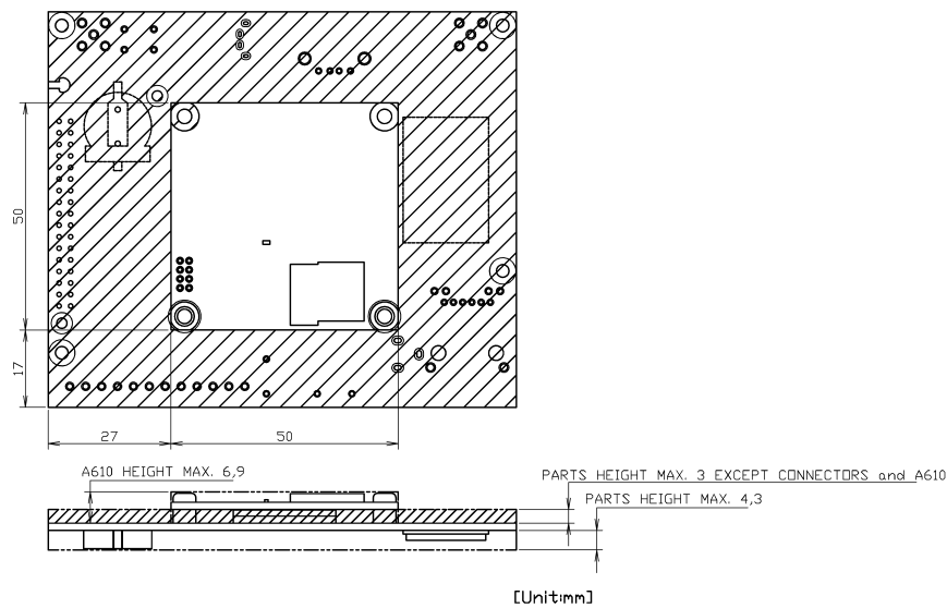
図 6.201 部品高さ
