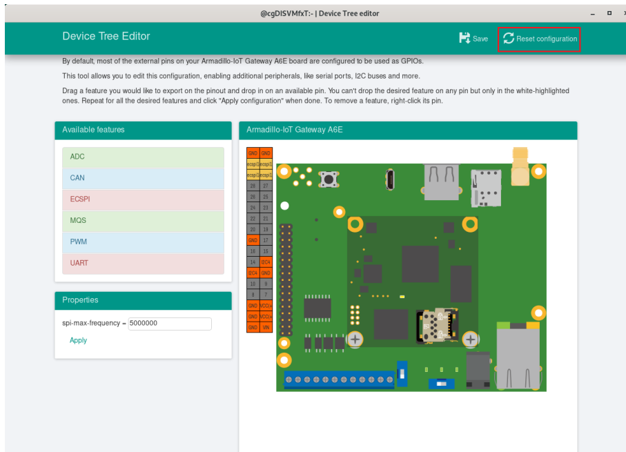
図 6.199 全ての機能の削除
