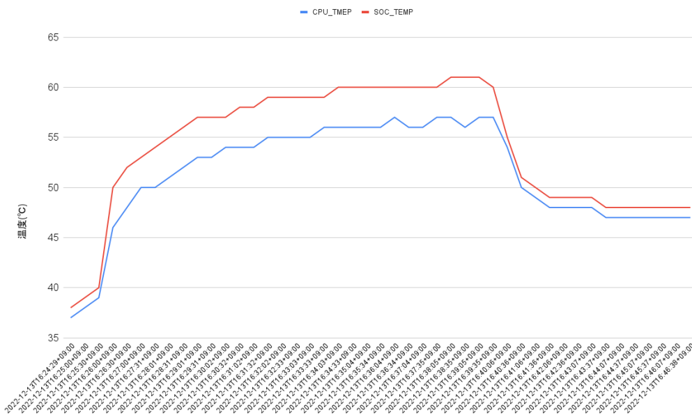
図 6.180 Armadillo-IoT ゲートウェイ G4 で取得した温度のグラフ
