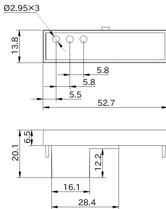
図 6.231 形状図 カバーパーツ C
