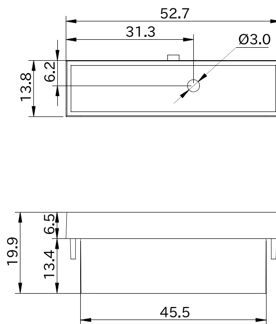
図 6.228 形状図 カバーパーツ A (アンテナ穴無し)
