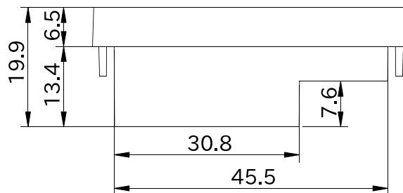
図 6.230 形状図 カバーパーツ B (アンテナ穴無し)
