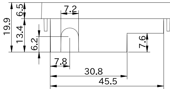
図 6.229 形状図 カバーパーツ B (アンテナ穴有り)
