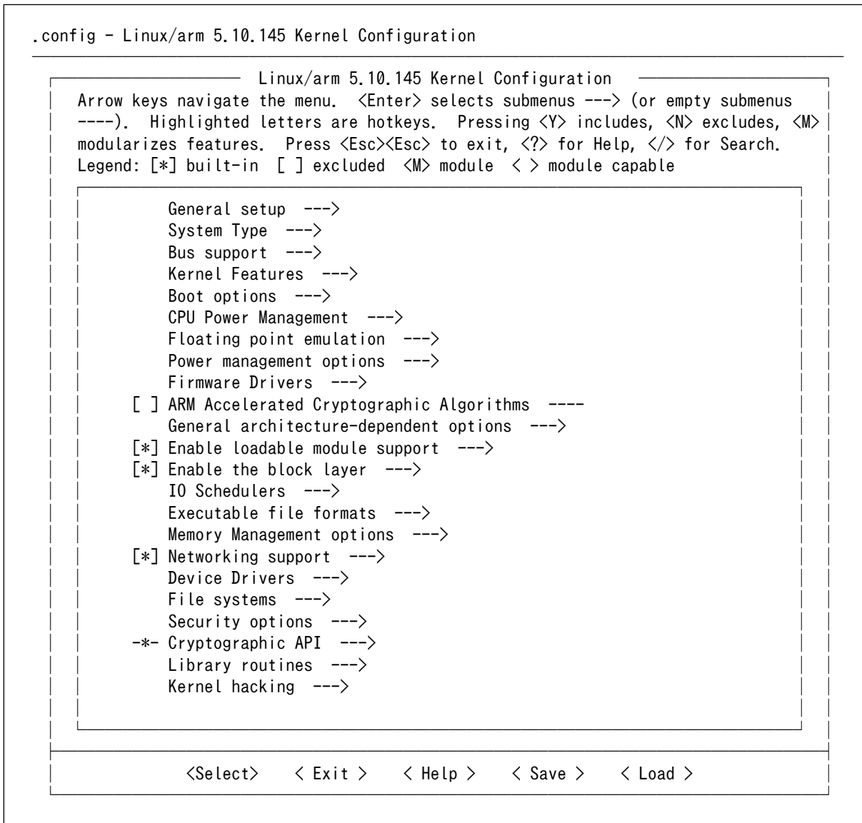
図 6.216 Linux カーネルコンフィギュレーション設定画面
