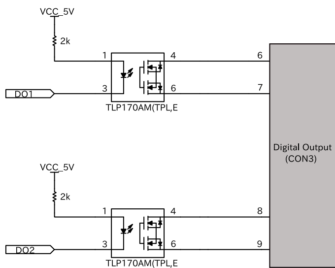
図 3.73 CON6 接点出力周辺回路
