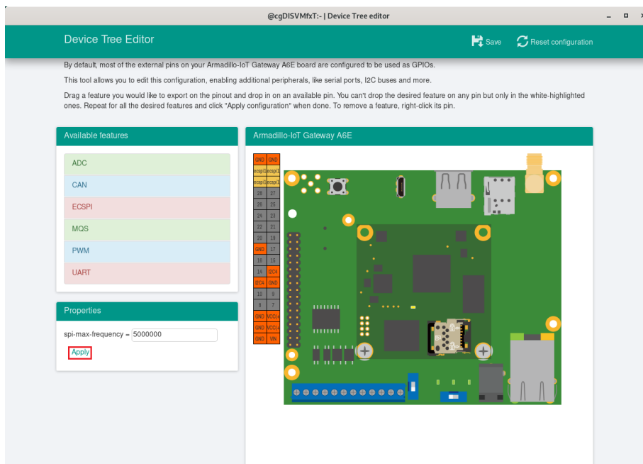
図 6.198 プロパティの保存
