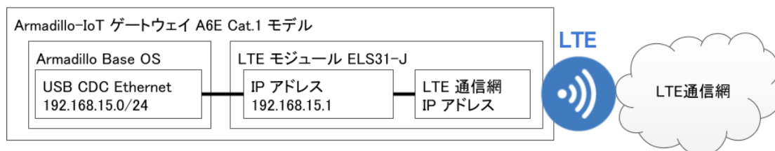
図 6.124 Cat.1 モデル (ELS31-J) LTE ネットワーク構成
