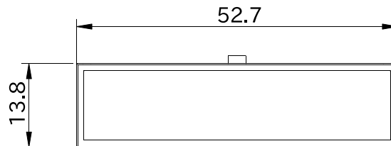
図 6.229 形状図 カバーパーツ B (アンテナ穴有り)
