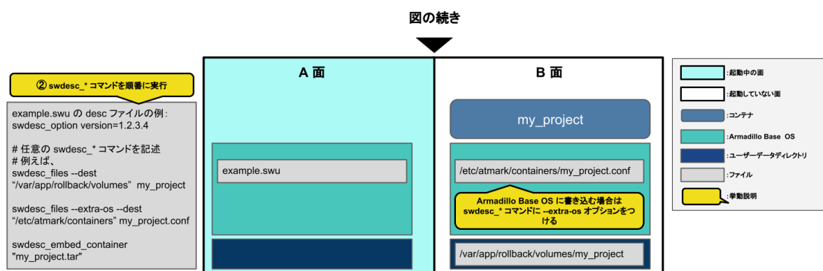
図 6.12 desc ファイルに記述した swudesc_* コマンドを実行
