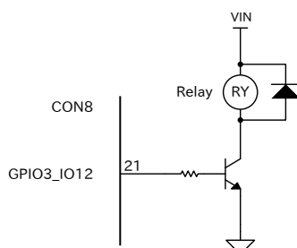
図 3.104 ピンを出力専用で使用した回路例
