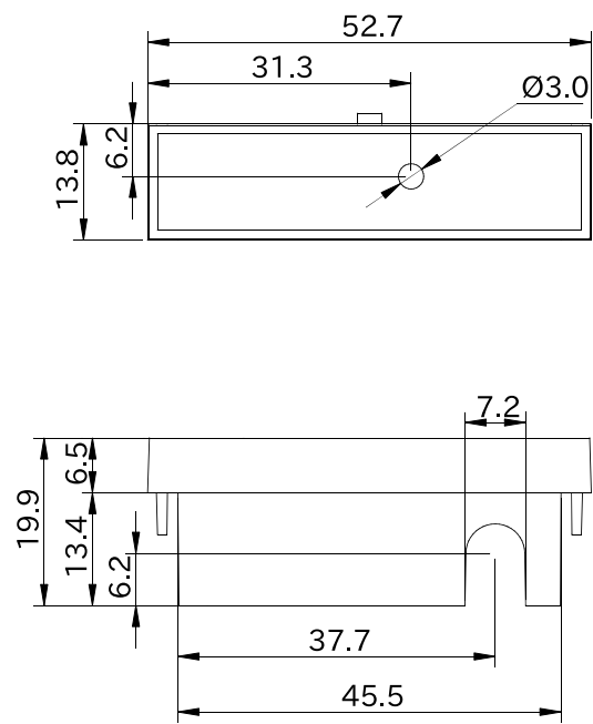
図 6.227 形状図 カバーパーツ A (アンテナ穴有り)
