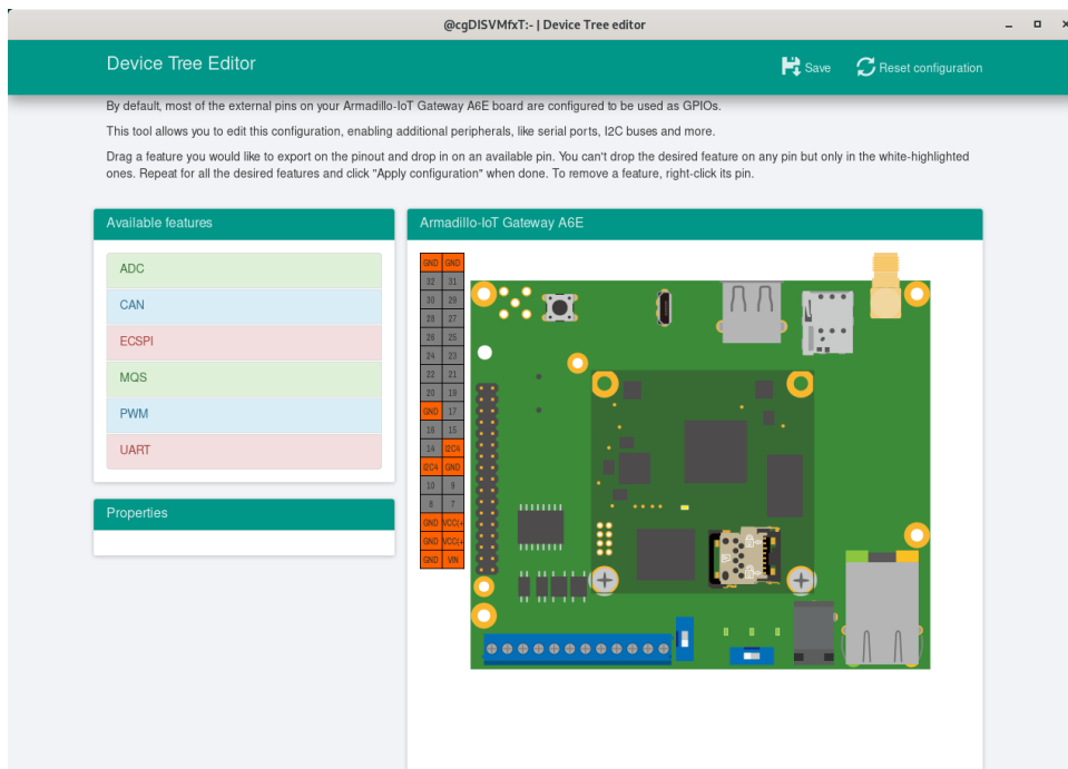
図 6.193 at-dtweb 起動画面
