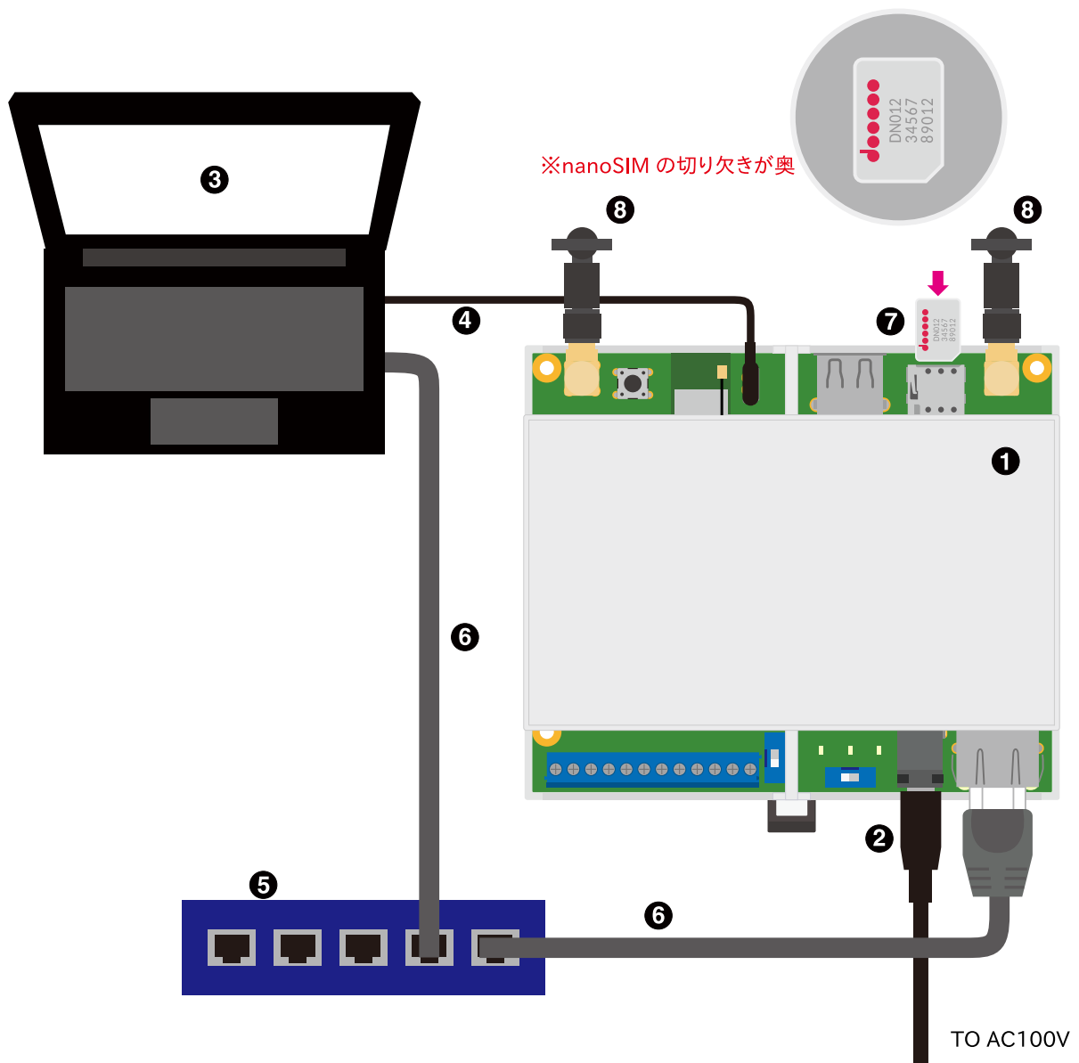
図 3.46 Armadillo-IoT ゲートウェイ A6E の接続例
