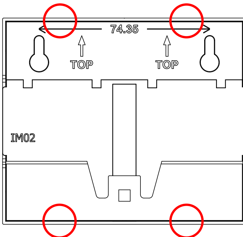
図 3.65 ケースボトムのツメ
