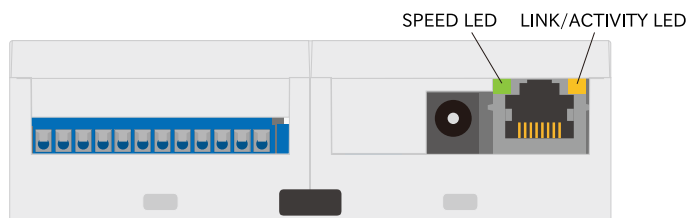
図 3.75 CON4 LAN LED
