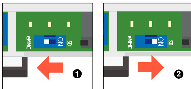
図 3.119 スwitchの状態と起動デバイス
