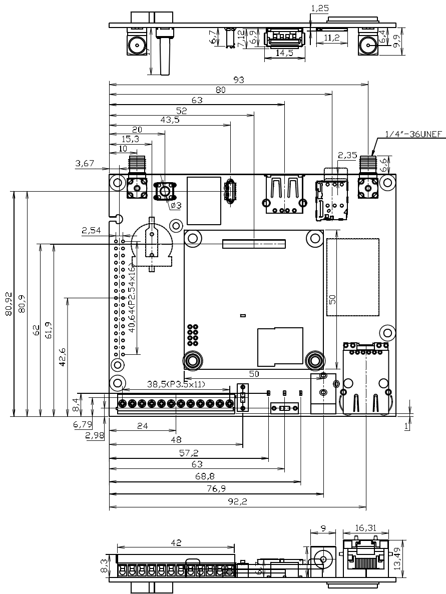
図 3.57 コネクタ、スイッチ、LED 位置
