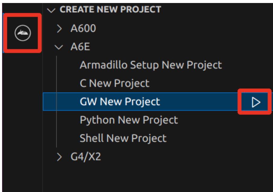
図 3.163 プロジェクトを作成する
