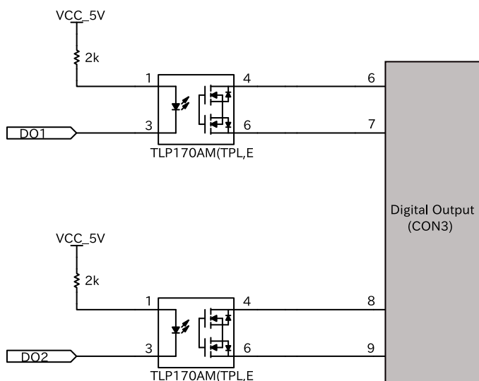
図 3.100 CON6 接点出力周辺回路
