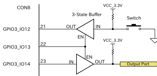
図 3.129 3-State バッファを使用した回路例
