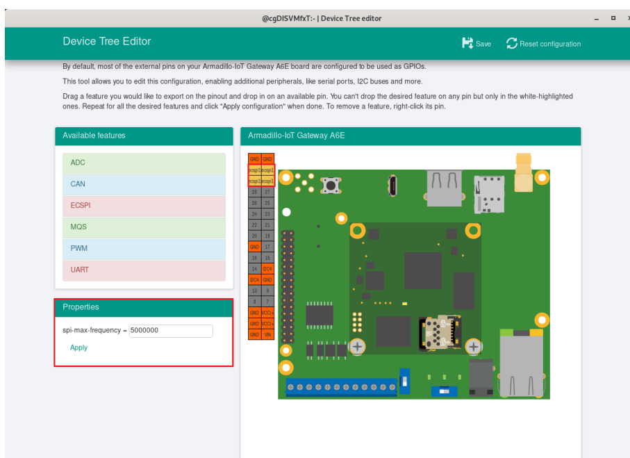
図 6.199 プロパティの設定
