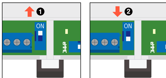
図 3.106 スイッチの状態と終端抵抗の ON/OFF
