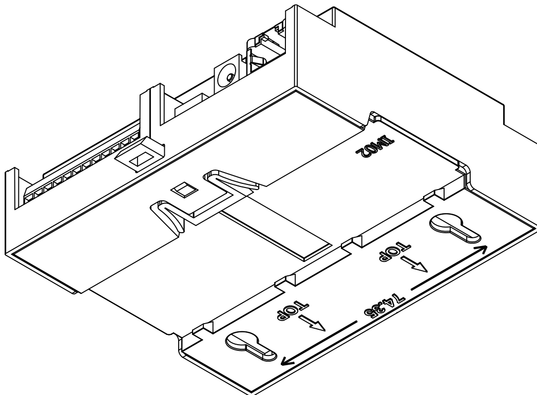
図 3.62 フック取り付け 2
