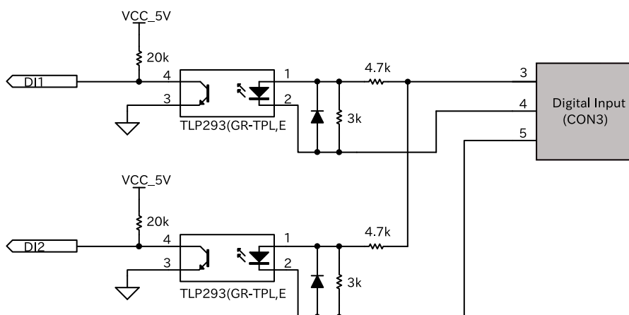
図 3.96 CON6 接点入力周辺回路
