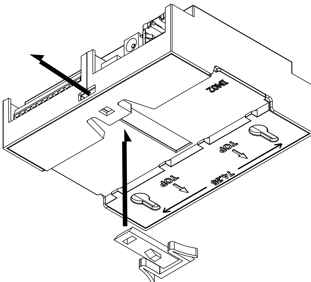
図 3.61 フック取り付け 1
