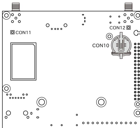
図 3.68 Armadillo-IoT ゲートウェイ A6E のインターフェース 裏面
