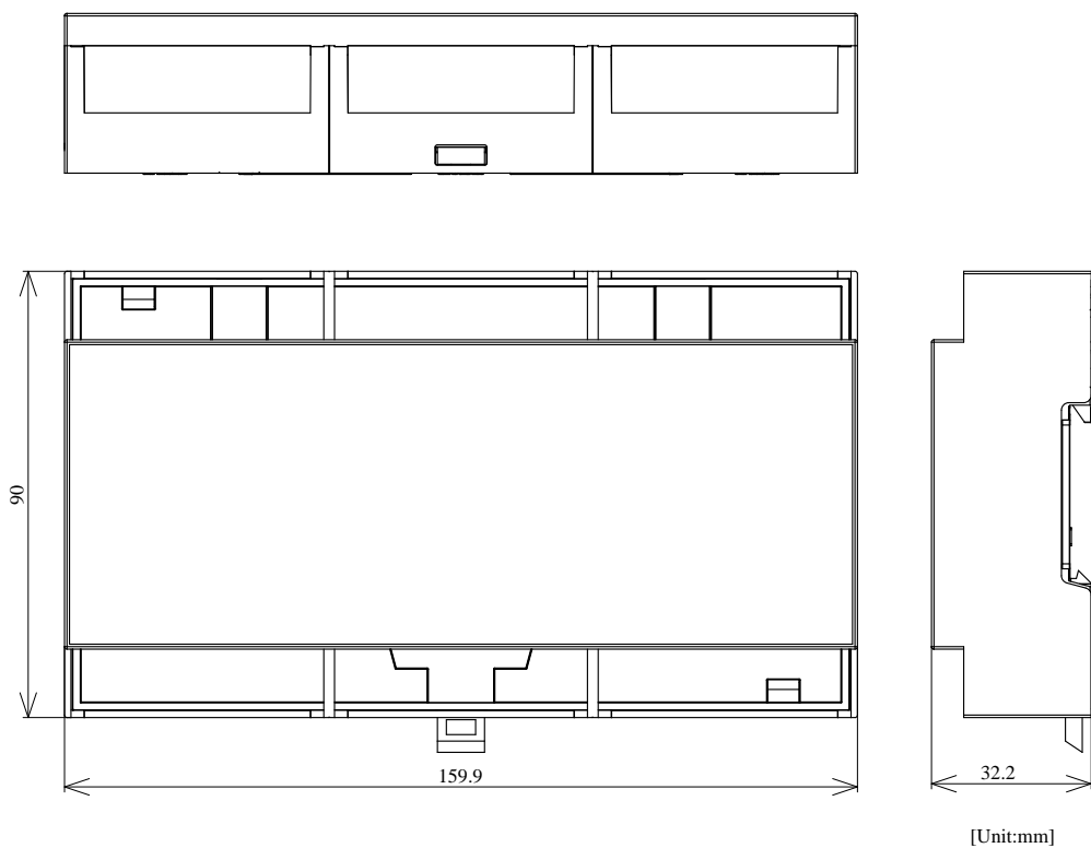
図 6.228 形状図 ケース外形(トップとボトムを組み合わせた状態)
