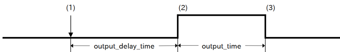
図 3.172 DO の出力タイミング
