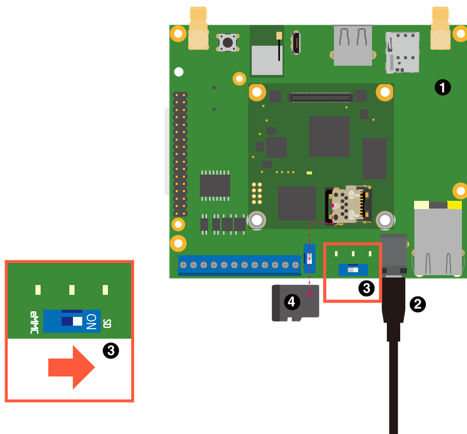
図 3.6 Armadillo-IoT ゲートウェイ A6E を初期化する接続
