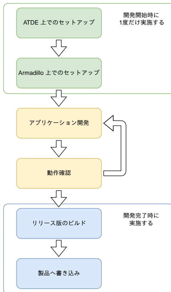
図 3.162 ゲートウェイコンテナアプリケーション開発の流れ
