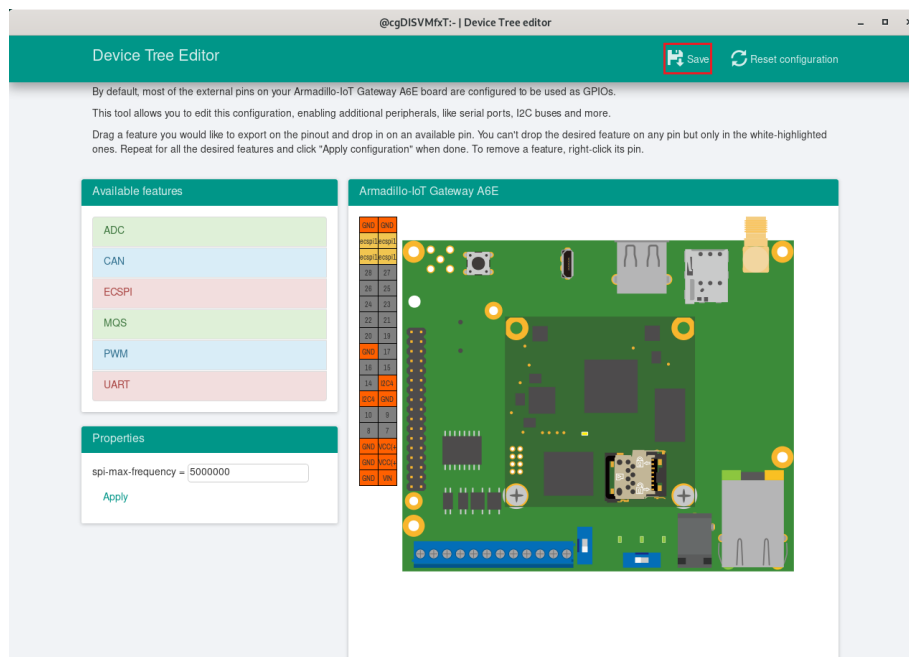
図 6.203 dtbo/desc ファイルの生成
