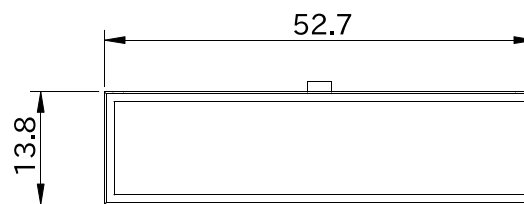
図 6.231 形状図 カバーパーツ A (アンテナ穴無し)
