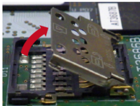
図 3.70 カバーを開ける
