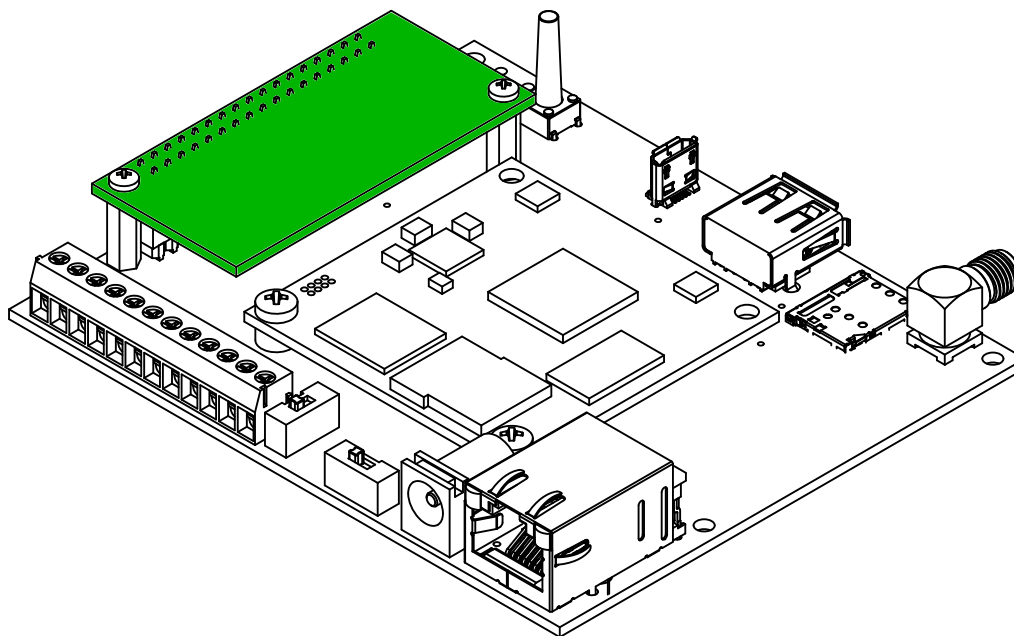
図 3.47 垂直方向に拡張基板を配置した場合の接続例
