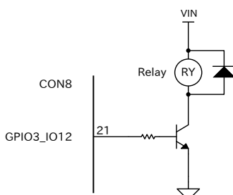
図 3.131 ピンを出力専用で使用した回路例
