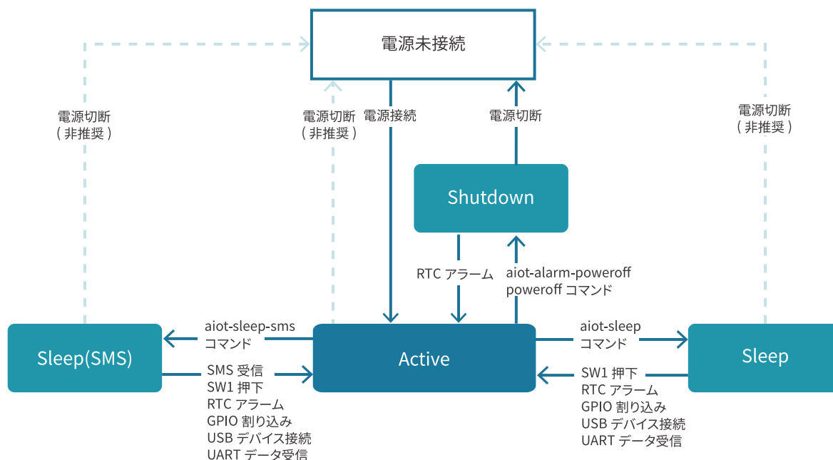
図 3.137 状態遷移図
