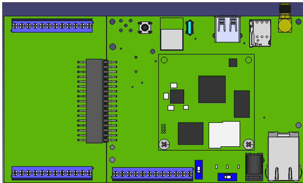
図 3.48 水平方向に拡張基板を配置した場合の接続例
