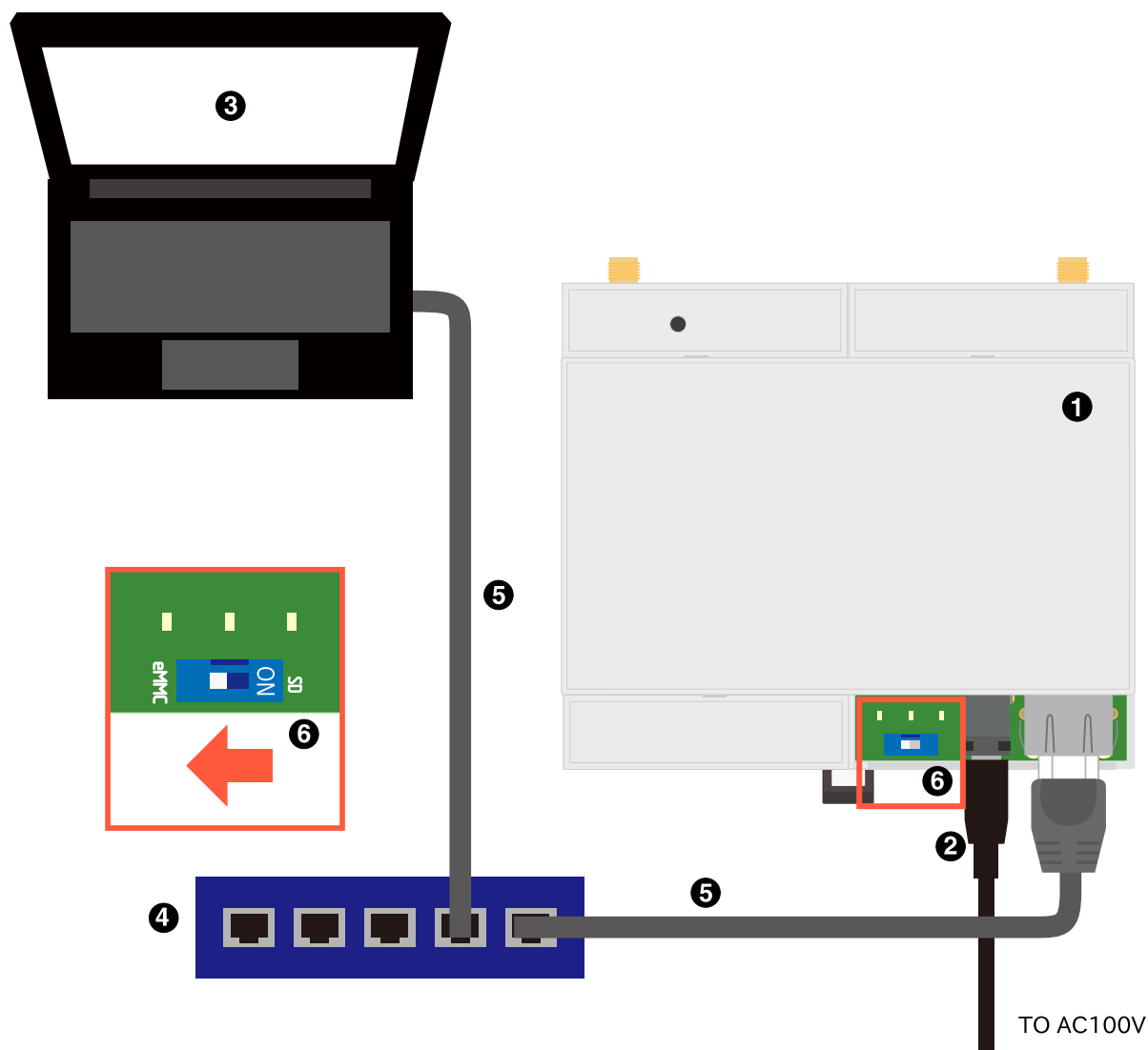
図 3.10 ABOS にアクセスするための接続
