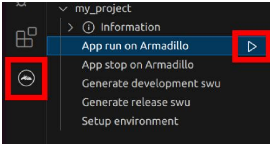
図 3.213 Armadillo 上でアプリケーションを実行する
