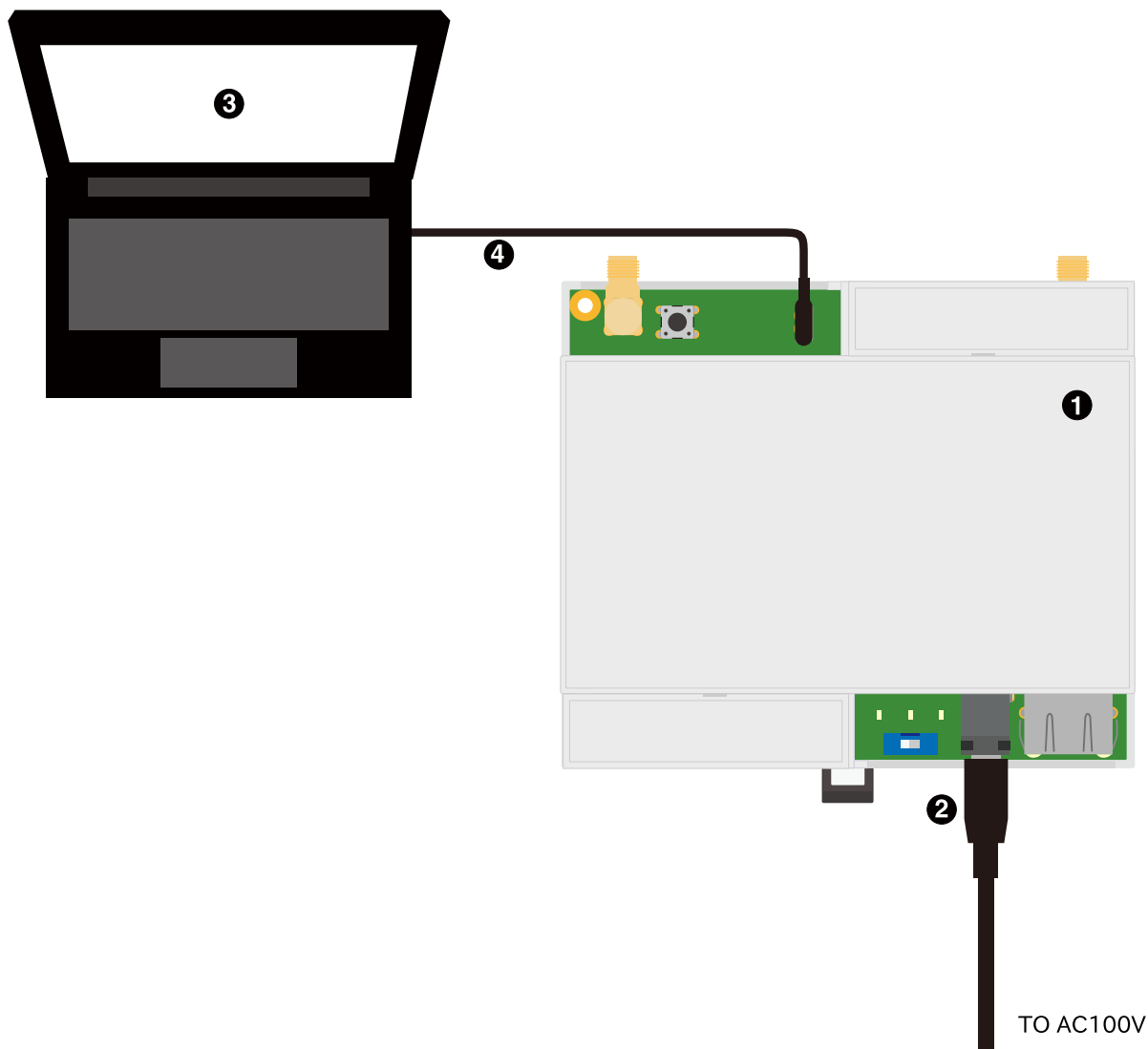
図 3.40 シリアルコンソールを使用する配線例
