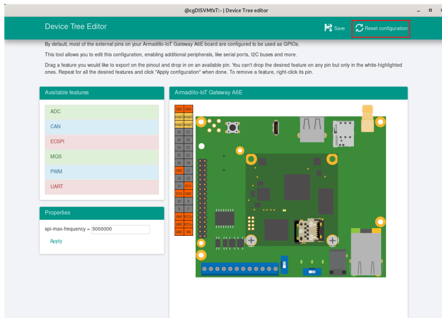
図 6.201 全ての機能の削除
