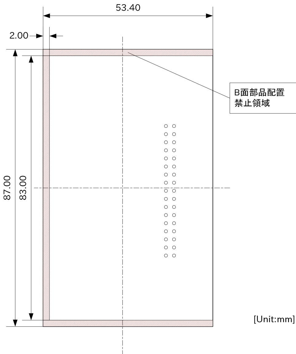
図 3.52 水平方向に拡張する場合の部品搭載制限(B 面側)
