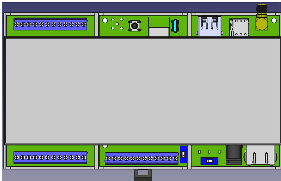
図 3.49 Armadillo-IoT ゲートウェイ A6E 標準ケースセットロング(9M) (OP-CASEA6E-PLA-20) 搭載例
