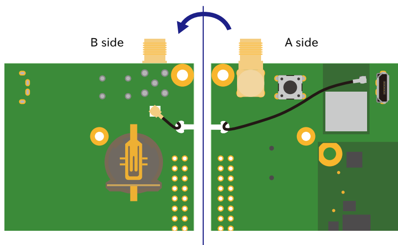
図 3.83 ANT2 カスタマイズ例：同軸ケーブル接続図
