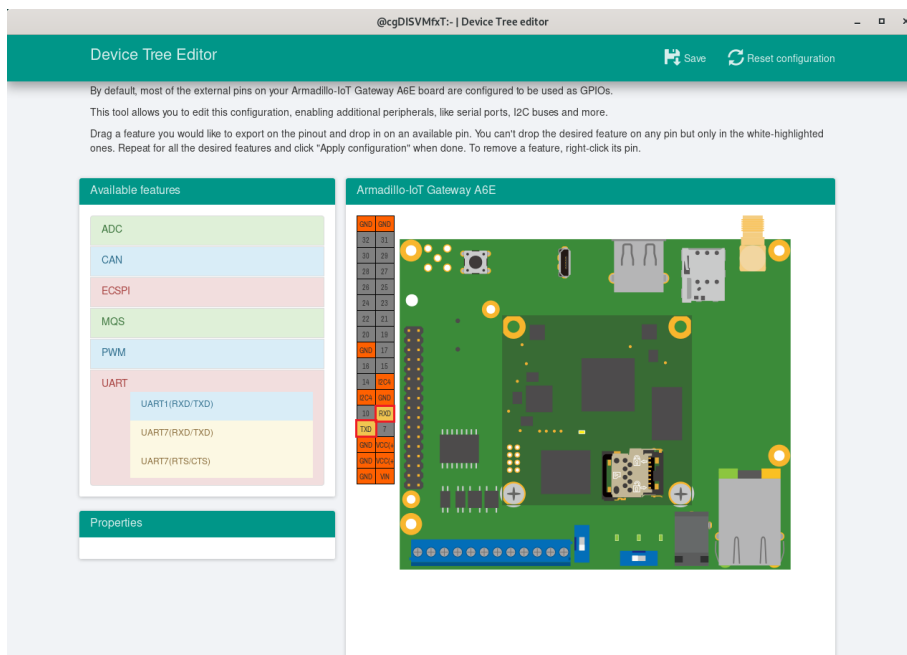
図 6.198 信号名の確認
