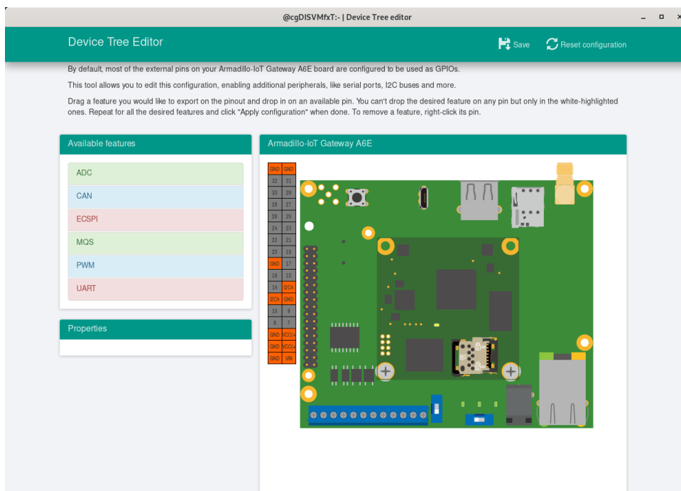
図 6.195 at-dtweb 起動画面
