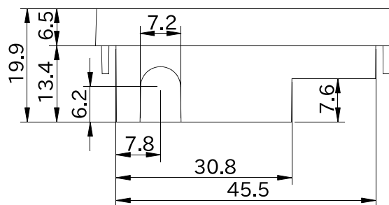
図 6.232 形状図 カバーパーツ B (アンテナ穴有り)
