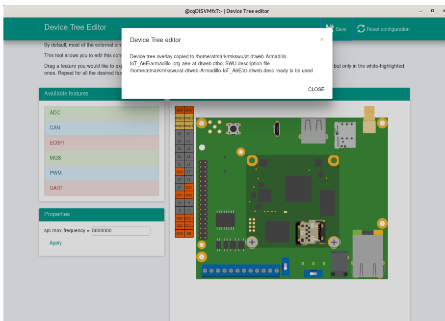
図 6.204 dtbo/desc の生成完了
