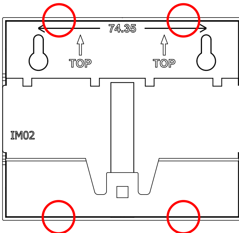
図 3.40 ケースボトムの実
