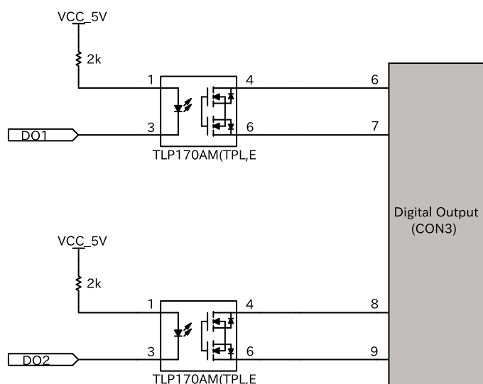
図 3.75 CON6 接点出力周辺回路
