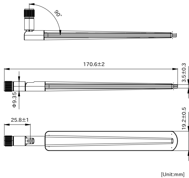
図 3.35 LTE アンテナ形状図
