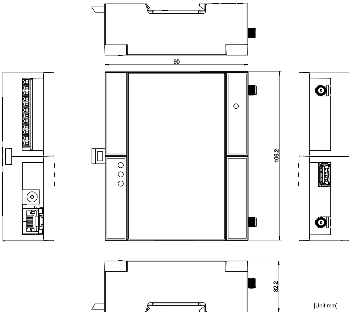
図 3.31 筐体形状
