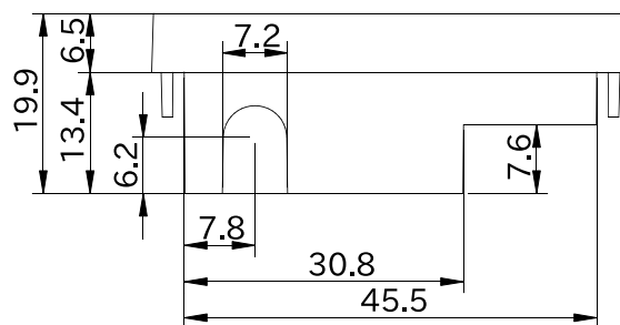
図 6.200 形状図 カバーパーツ B (アンテナ穴有り)
