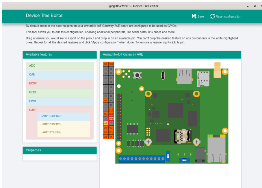
図 6.171 CON8 8/9 ピンへのドロップ
