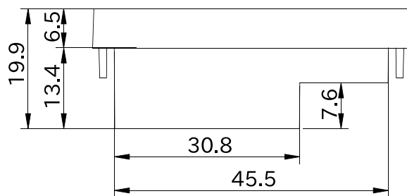
図 6.201 形状図 カバーパーツ B (アンテナ穴無し)
