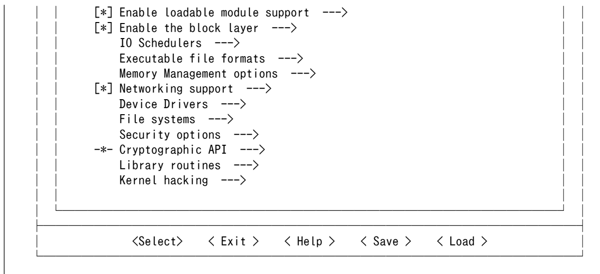
図 6.187 Linux カーネルコンフィギュレーション設定画面
