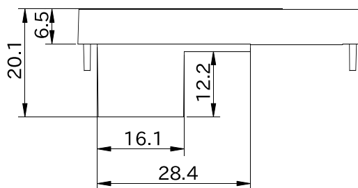
図 6.202 形状図 カバーパーツ C
