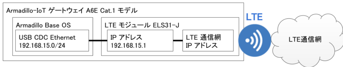
図 6.102 Cat.1 モデル (ELS31-J) LTE ネットワーク構成
