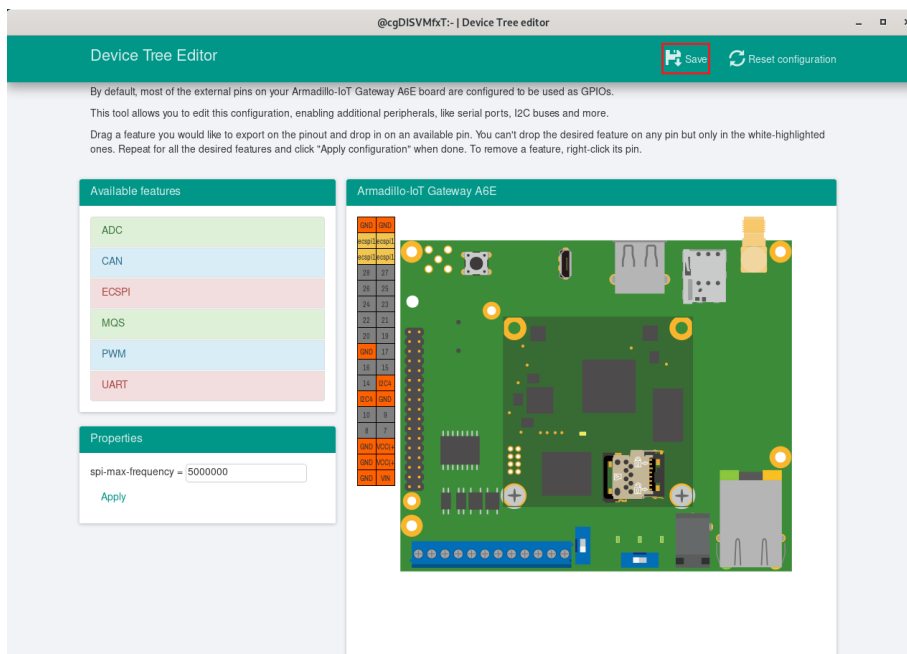
図 6.177 dtbo/desc ファイルの生成
