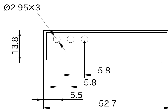
図 6.201 形状図 カバーパーツ B (アンテナ穴無し)
