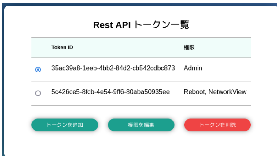
図 6.85 設定管理の Rest API トークン一覧表示
