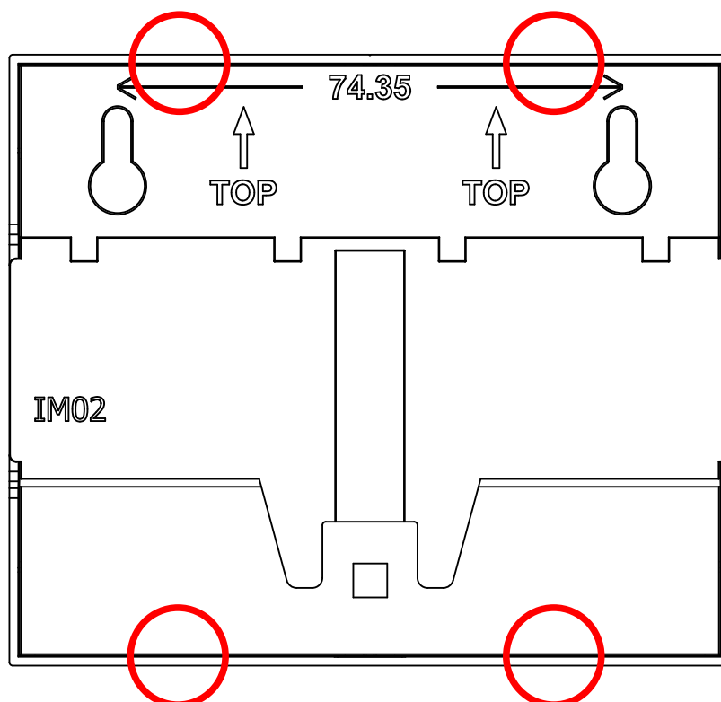
図 3.38 ケースボトムของツメ
