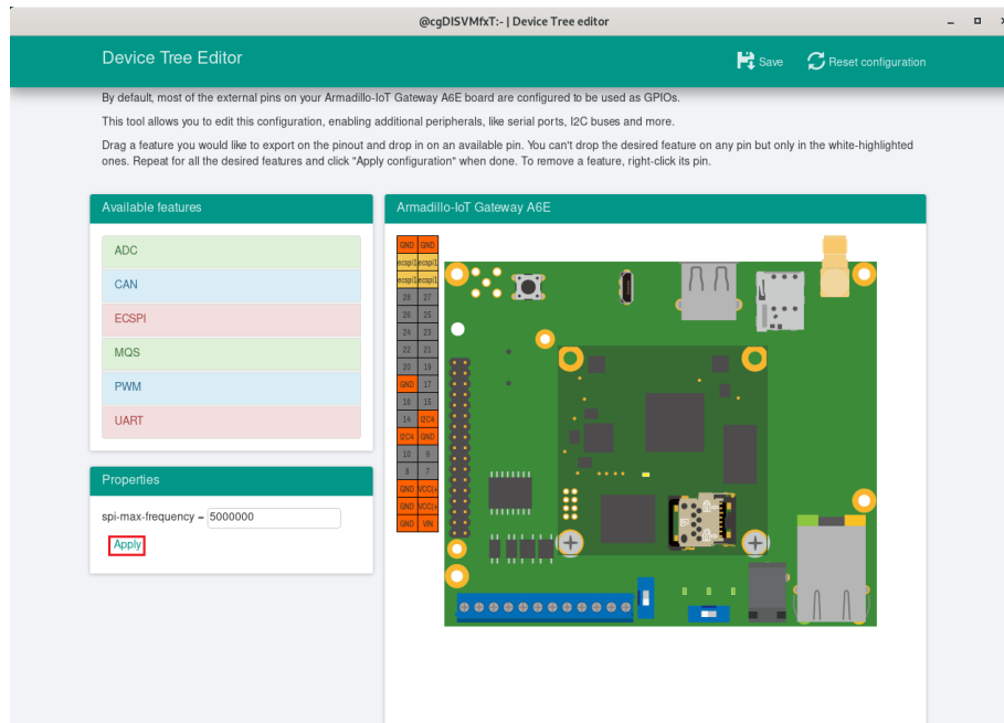
図 6.174 プロパティの保存
