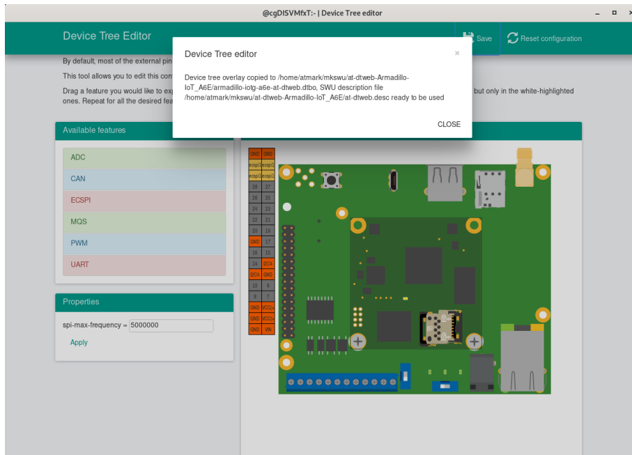
図 6.178 dtbo/desc の生成完了
