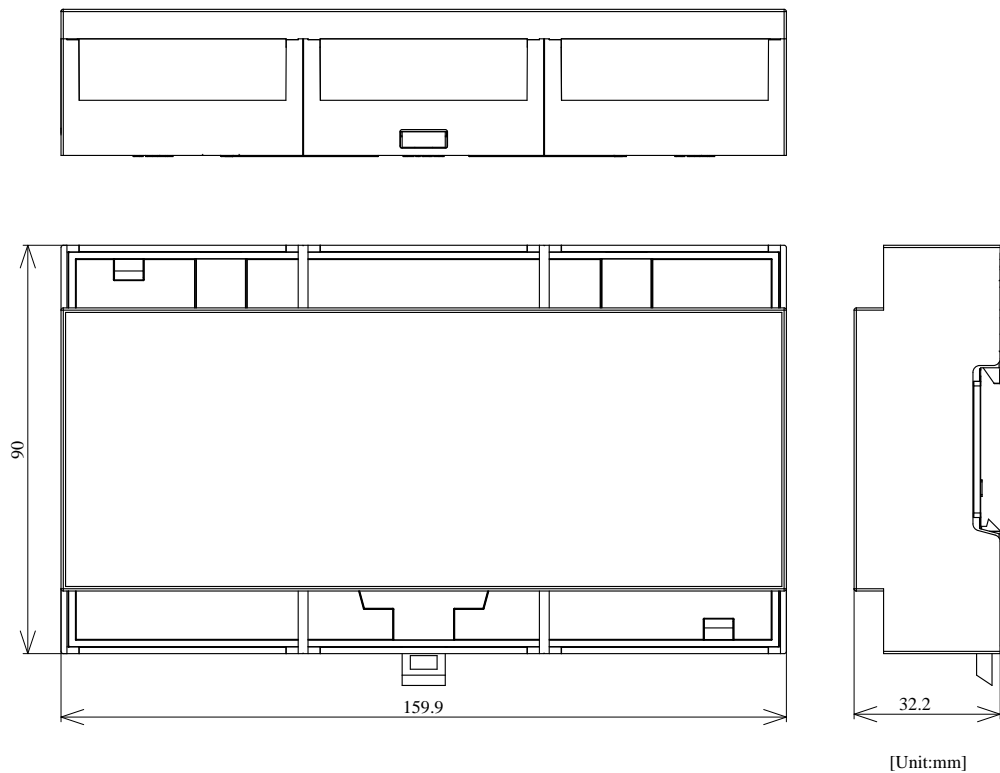
図 6.196 形状図 ケース外形(トップとボトムを組み合わせた状態)
