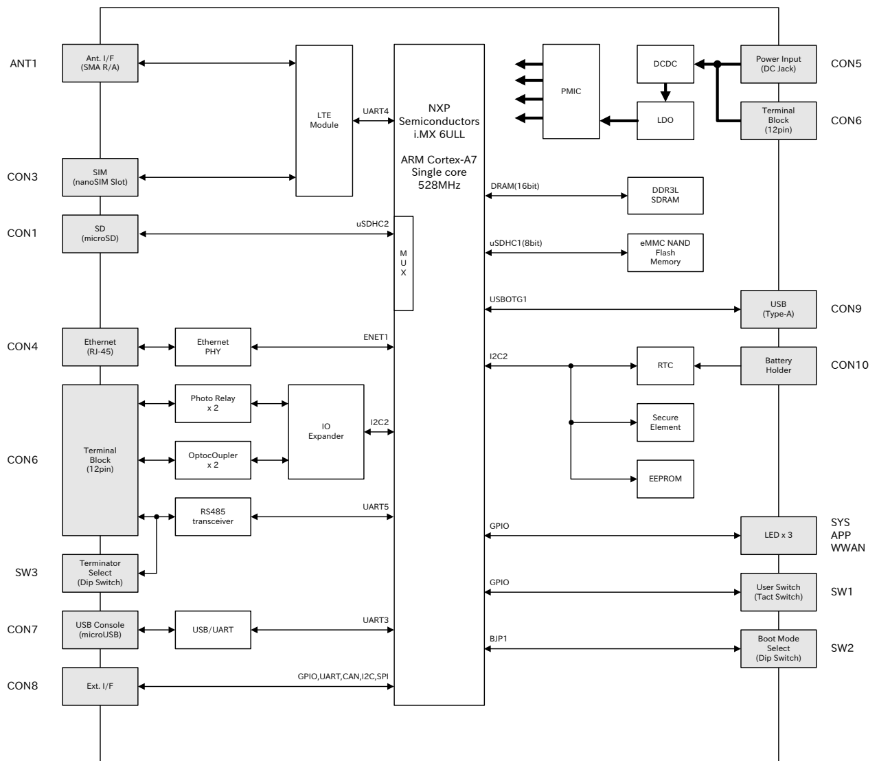
図 2.13 ブロック図(AG6221-C01D0,AG6221-C01Z,AG6221-U01Z,AG6221-U00Z)
