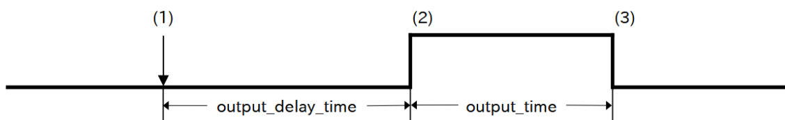
図 3.136 DO の出力タイミング
