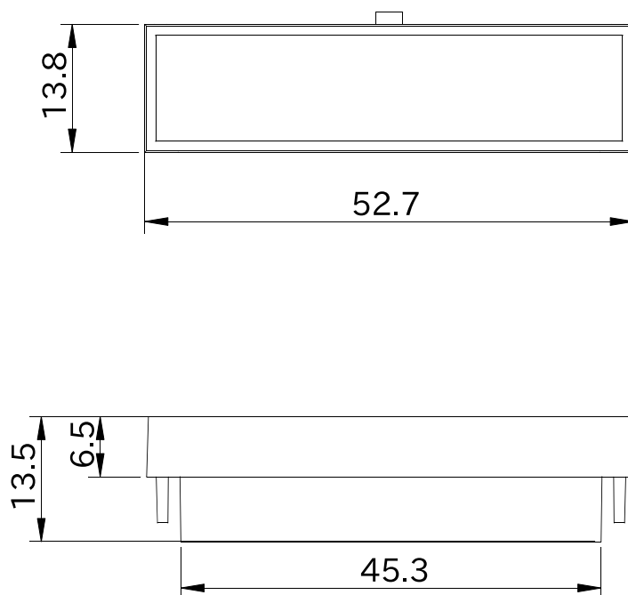
図 6.203 形状図 カバーパーツ D
