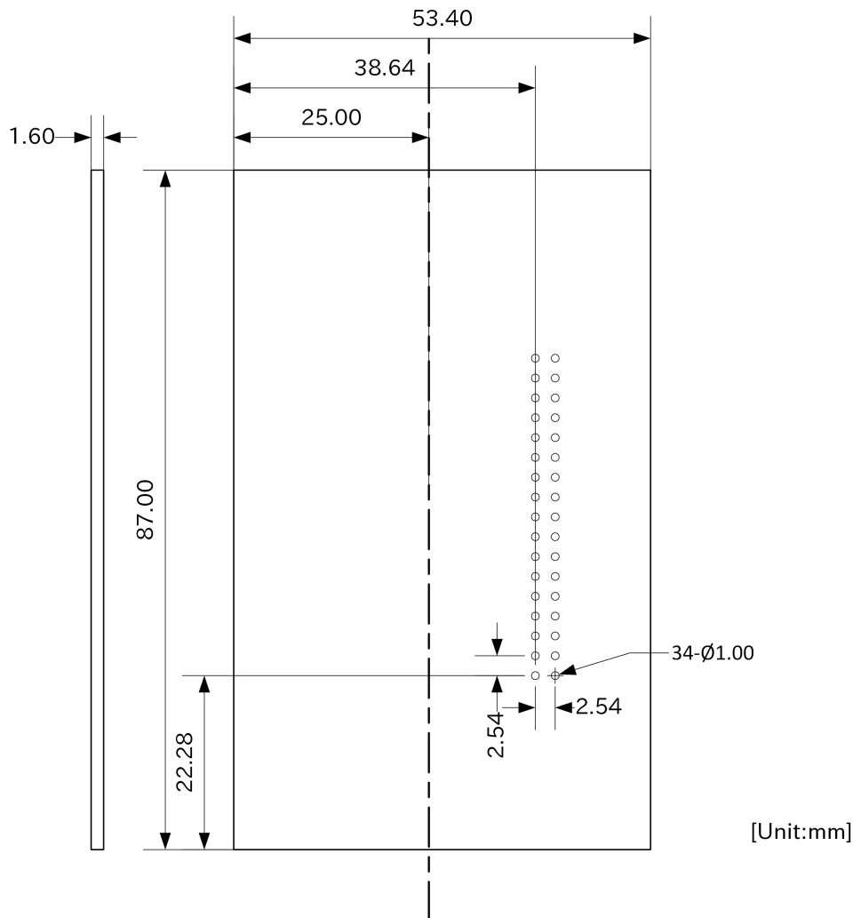
図 3.24 水平方向に拡張する場合の基板形状図
