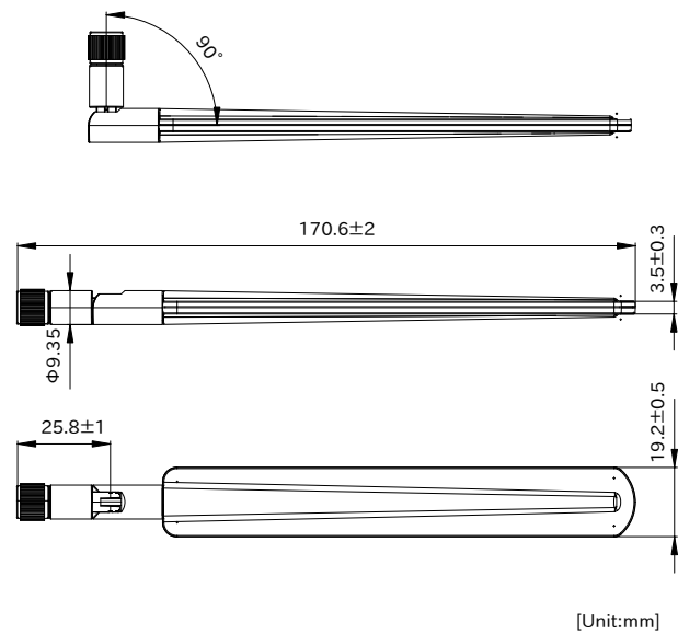
図 3.33 LTE アンテナ形状図
