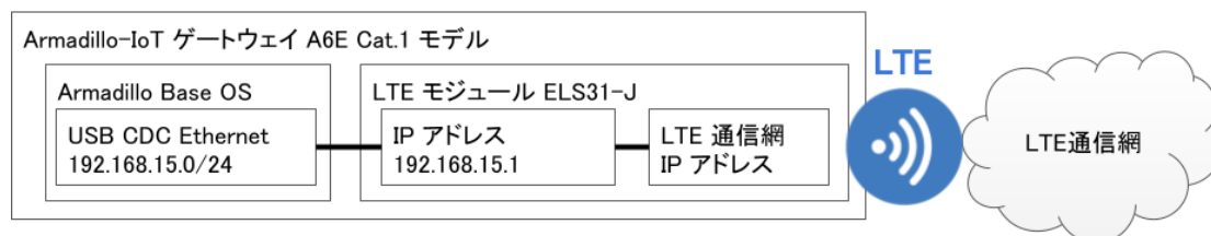
図 6.110 Cat.1 モデル (ELS31-J) LTE ネットワーク構成
