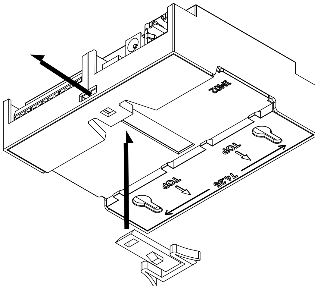
図 3.35 フック取り付け 1
