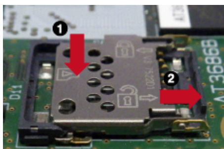
図 3.42 カバーのロックを解除する
