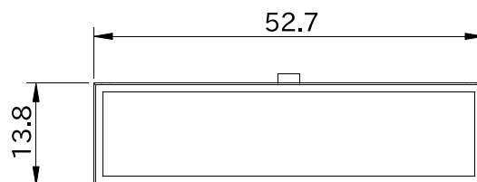
図 6.207 形状図 カバーパーツ A (アンテナ穴無し)
