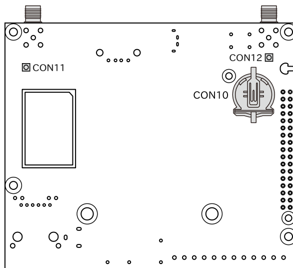
図 3.41 Armadillo-IoT ゲートウェイ A6E のインターフェース 裏面
