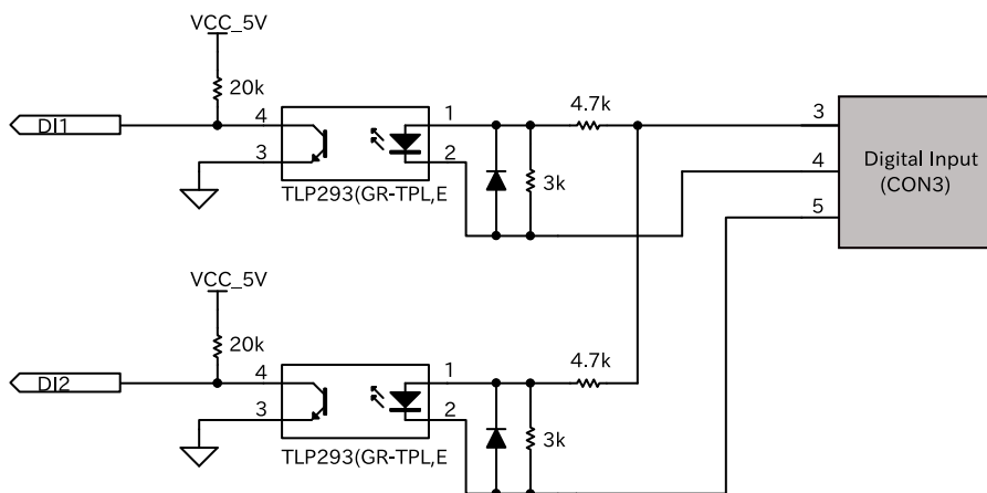
図 3.69 CON6 接点入力周辺回路
