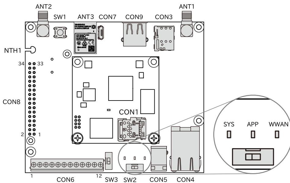
図 3.40 Armadillo-IoT ゲートウェイ A6E のインターフェース 表面
