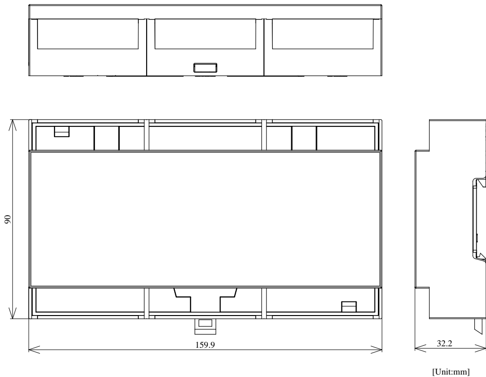
図 6.204 形状図 ケース外形(トップとボトムを組み合わせた状態)
