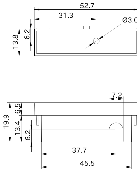
図 6.206 形状図 カバーパーツ A (アンテナ穴有り)
