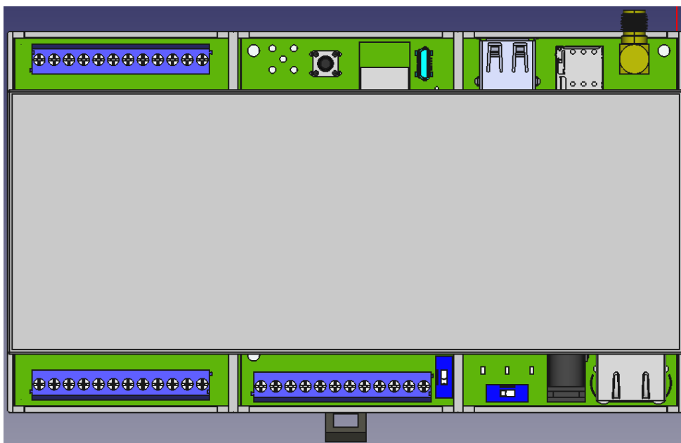
図 3.23 Armadillo-IoT ゲートウェイ A6E 標準ケースセットロング(9M) (OP-CASEA6E-PLA-20) 搭載例
