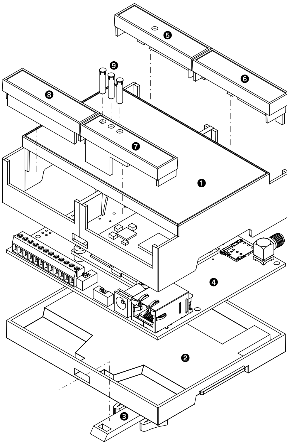
図 3.34 ケースモデル展開図
