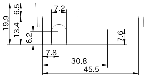
図 6.208 形状図 カバーパーツ B (アンテナ穴有り)
