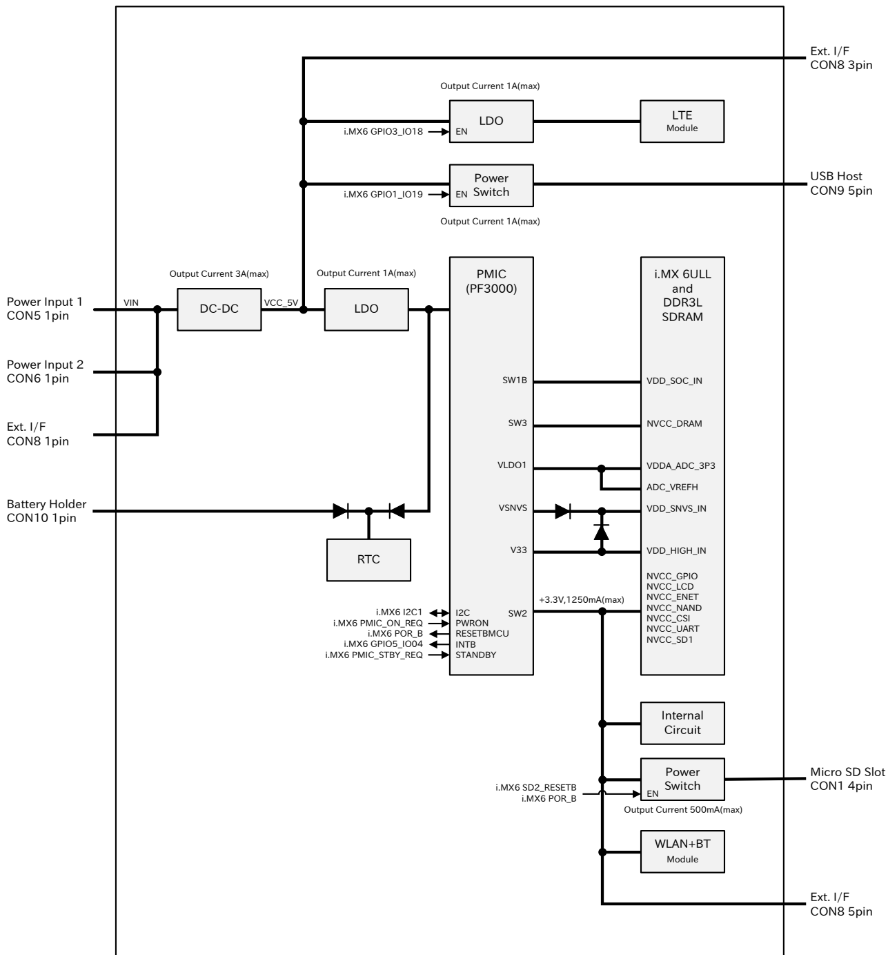
図 3.27 電源回路の構成
