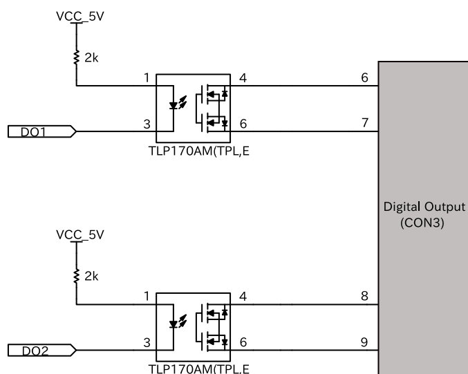
図 3.73 CON6 接点出力周辺回路
