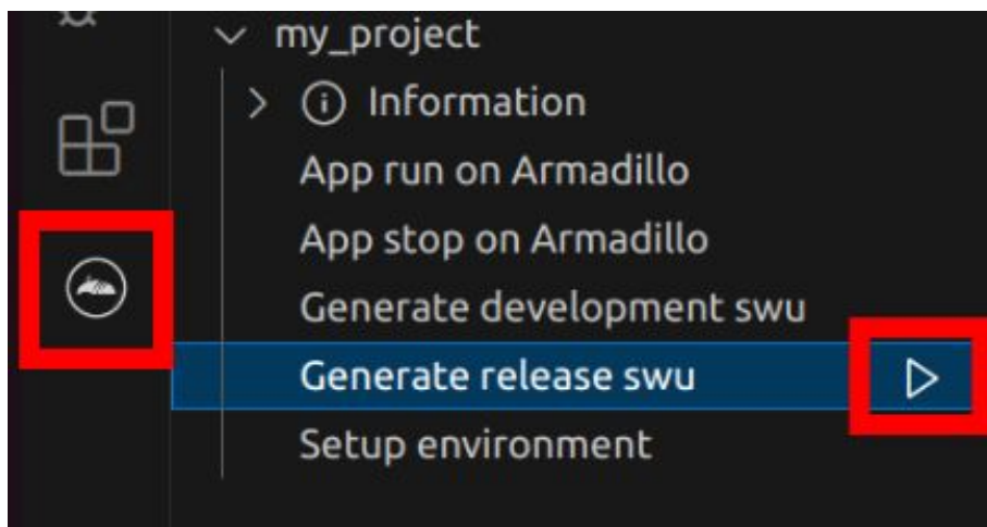
図 3.187 リリース版をビルドする
