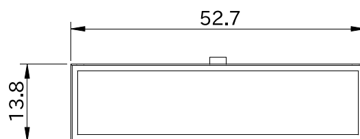
図 6.211 形状図 カバーパーツ A (アンテナ穴無し)
