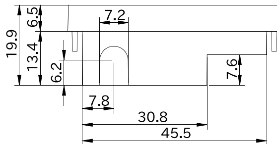
図 6.212 形状図 カバーパーツ B (アンテナ穴有り)
