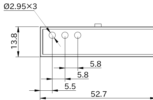
図 6.213 形状図 カバーパーツ B (アンテナ穴無し)
