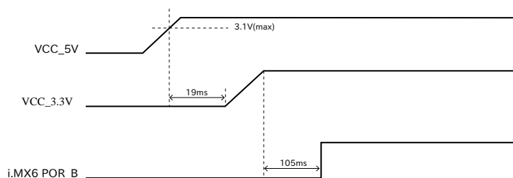
図 3.28 電源シーケンス
