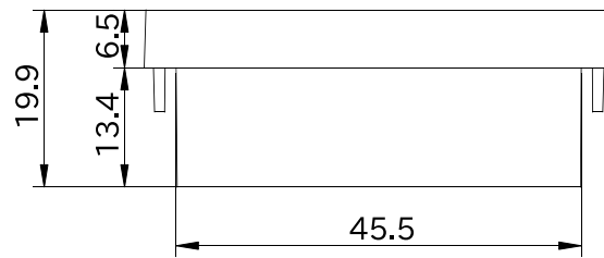
図 6.211 形状図 カバーパーツ A (アンテナ穴無し)
