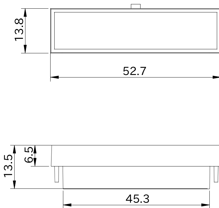
図 6.215 形状図 カバーパーツ D
