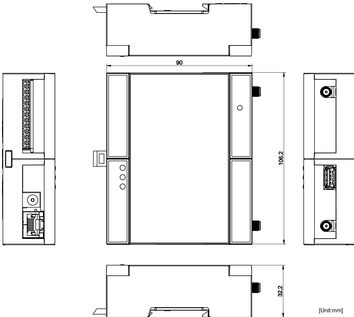
図 3.29 筐体形状
