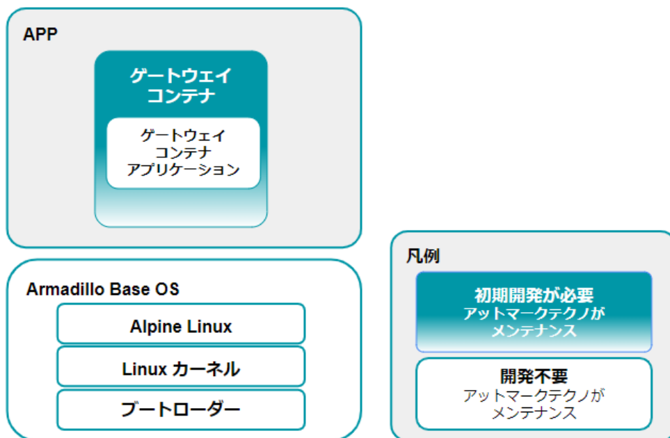
図 3.106 ゲートウェイコンテナ使用時、開発者が開発するもの、開発しなくていいもの
