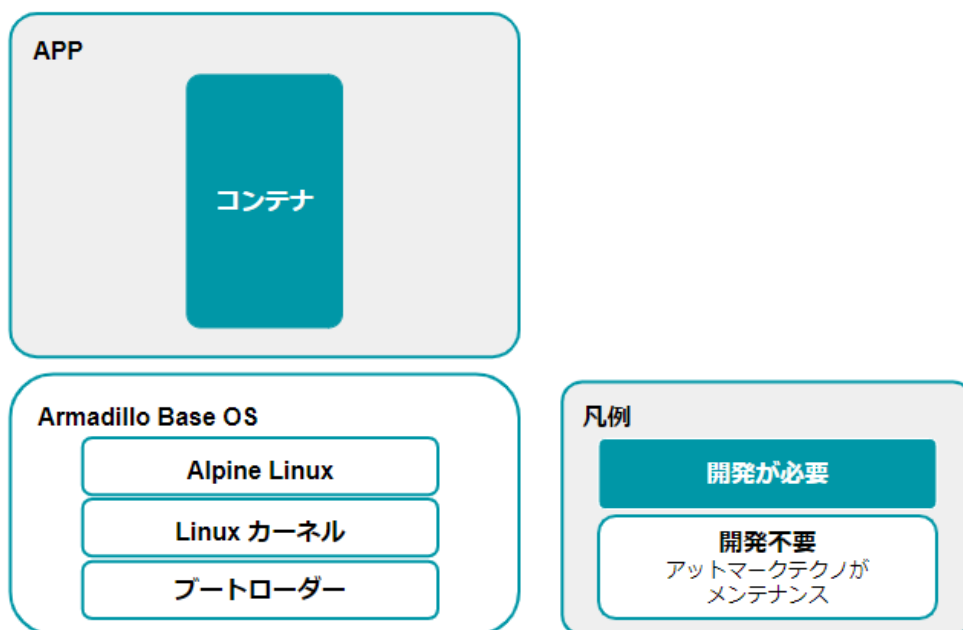
図 3.105 開発者が開発するもの、開発しなくていいもの
