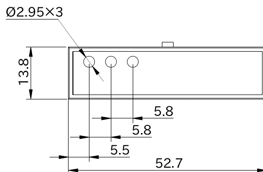
図 6.213 形状図 カバーパーツ B (アンテナ穴無し)
