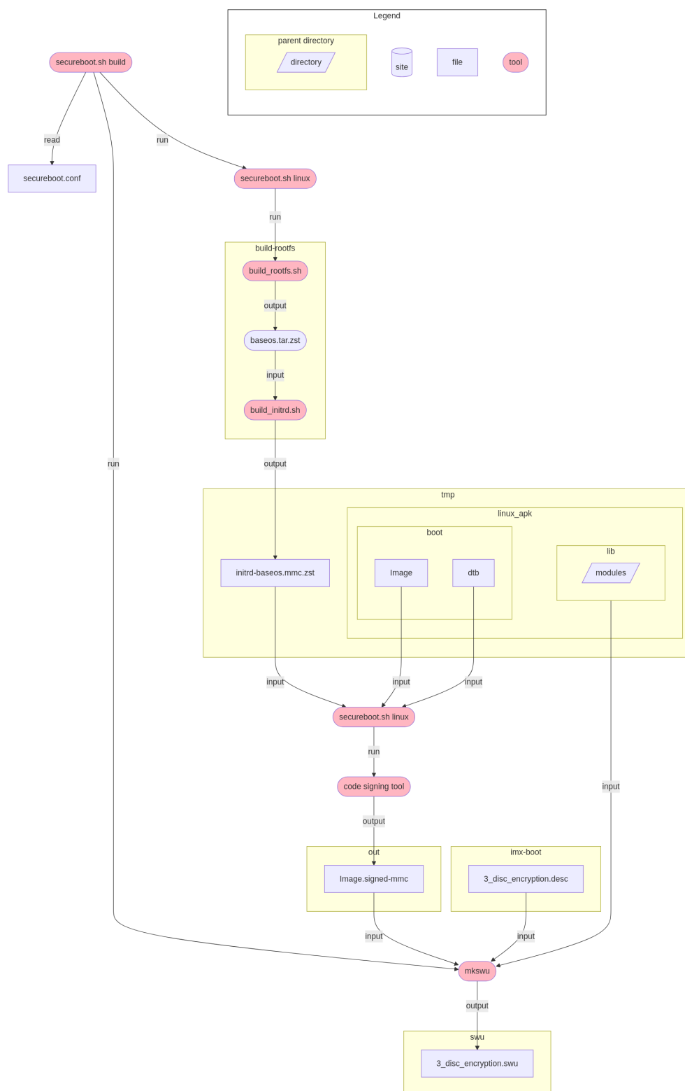
図 3.10 3_disk_encryption.swu を生成するまでの流れ
