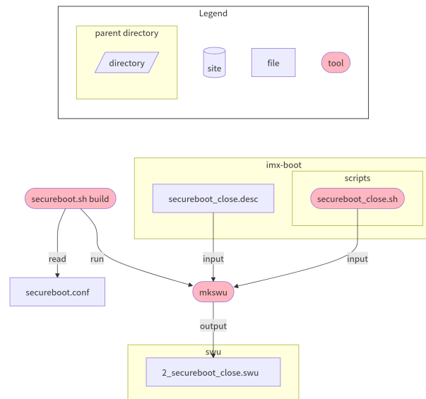
図 3.9 2_secureboot_close.swu を生成するまでの流れ
