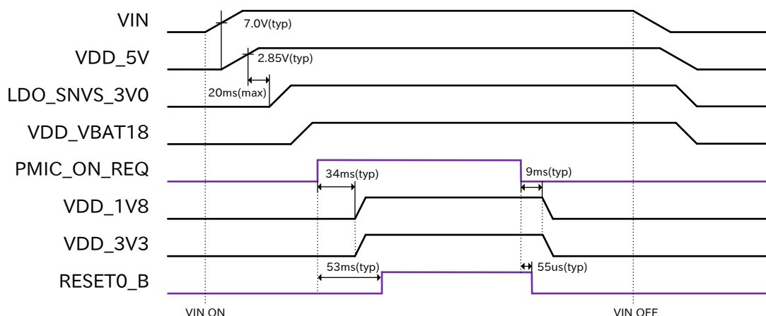
図 3.64 電源シーケンス
