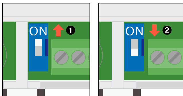
図 3.111 スwitchの状態と終端抵抗の ON/OFF
