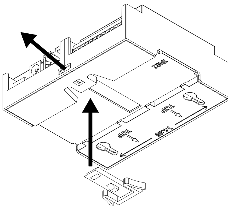
図 3.72 フック取り付け 1
