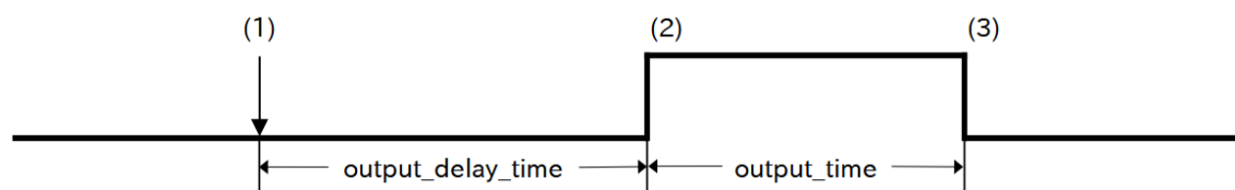
図 3.195 DO の出力タイミング
