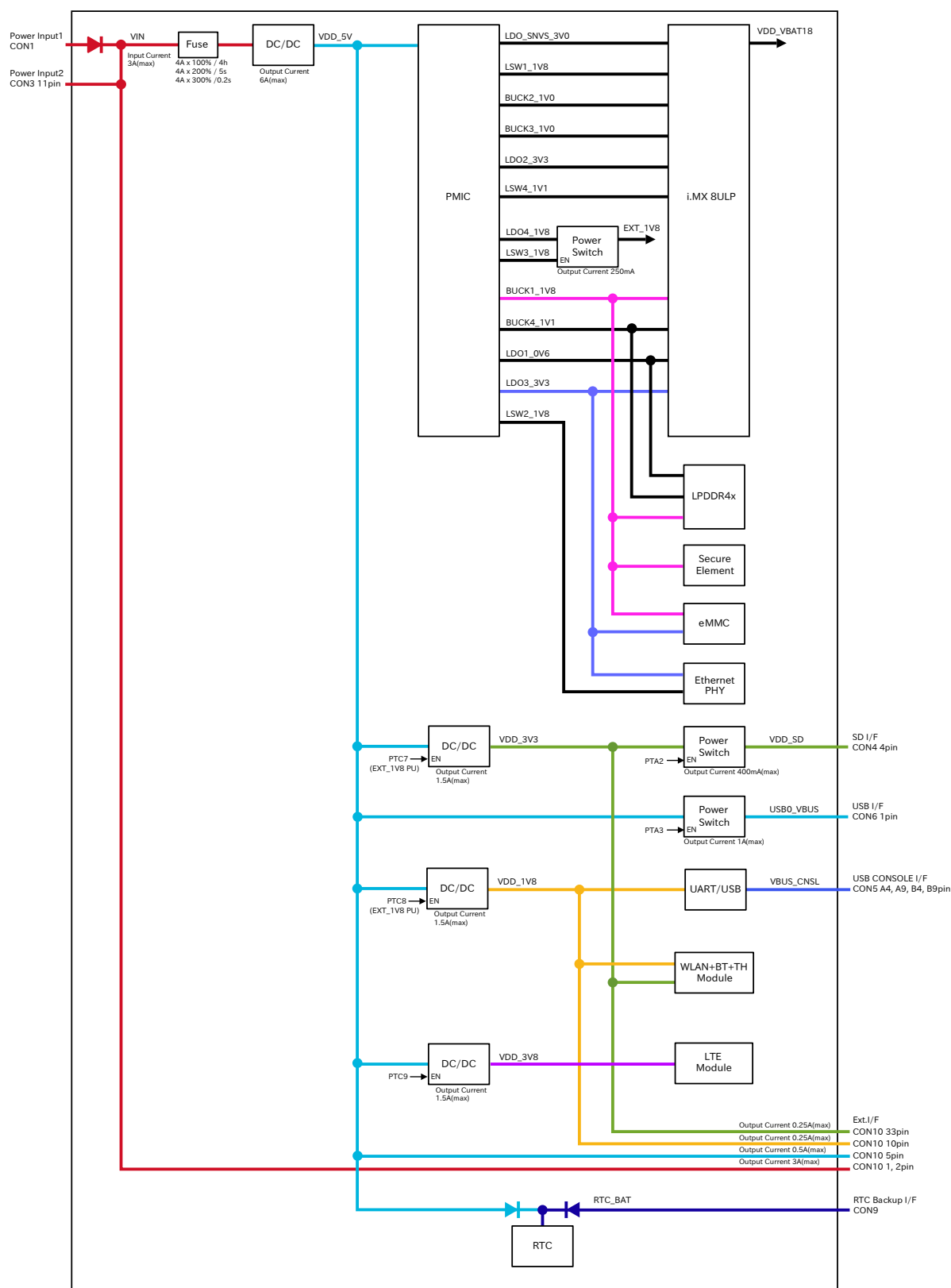
図 3.63 電源回路の構成
