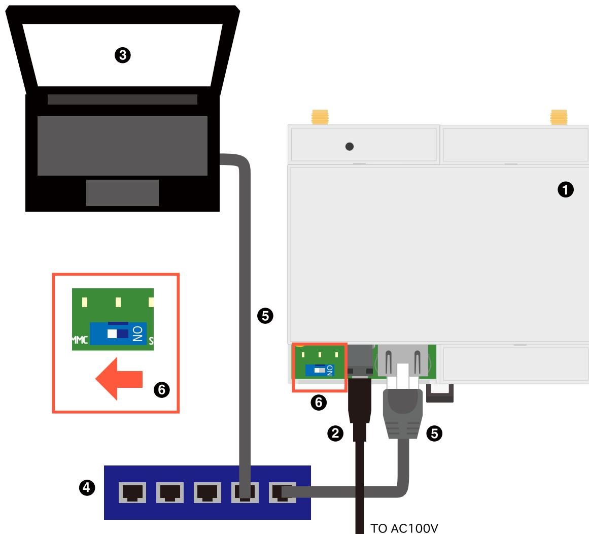
図 3.23 ABOS にアクセスするための接続
