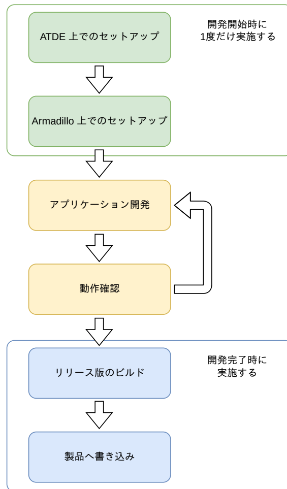
図 3.207 CUI アプリケーション開発の流れ
