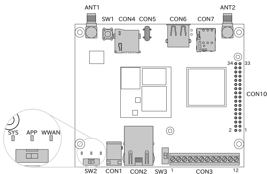
図 3.77 Armadillo-IoT ゲートウェイ A9E のインターフェース 表面
