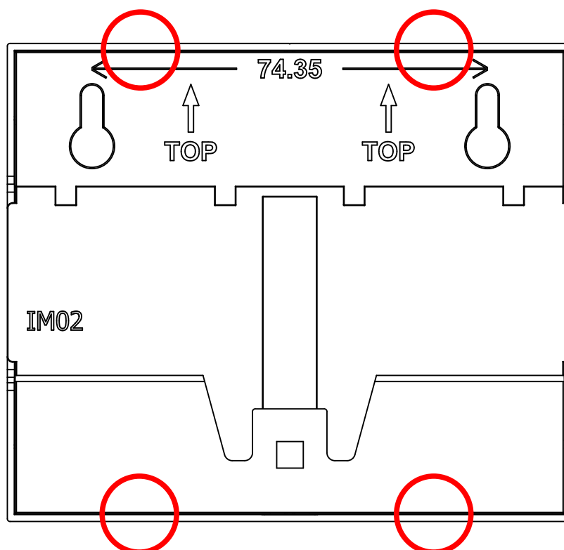
図 3.75 ケースボトムのツメ
