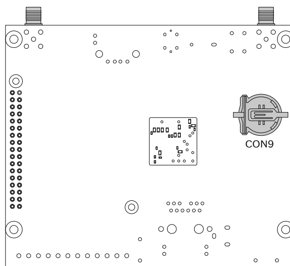
図 3.78 Armadillo-IoT ゲートウェイ A9E のインターフェース 裏面
