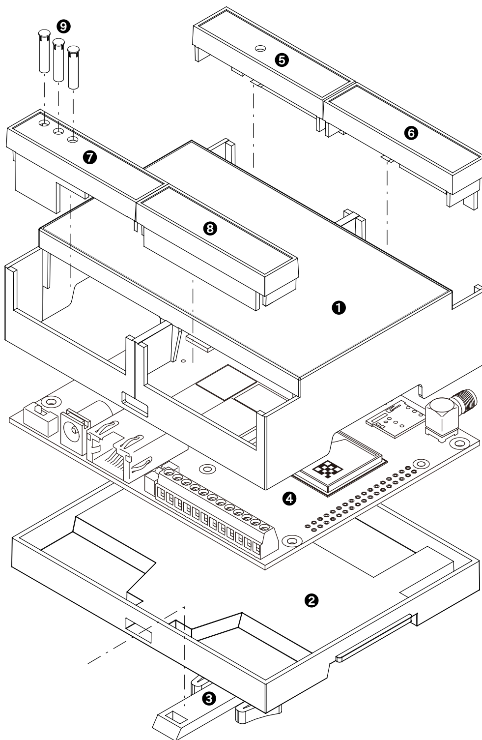
図 3.71 ケースモデル展開図
