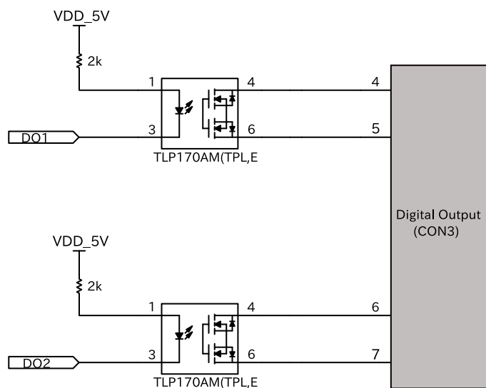
図 3.105 CON3 接点出力周辺回路
