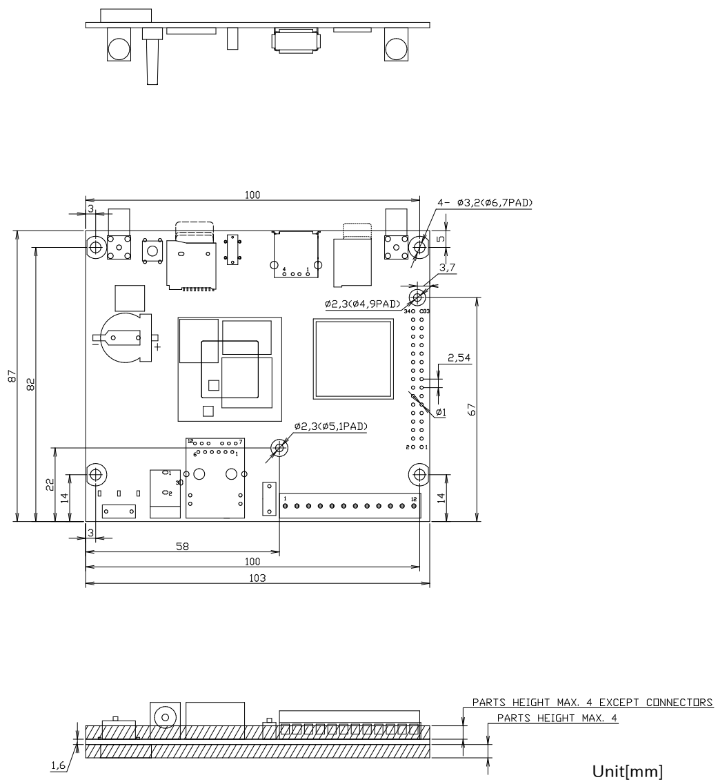
図 3.67 基板形状図（外形、固定穴、部品高さ）
