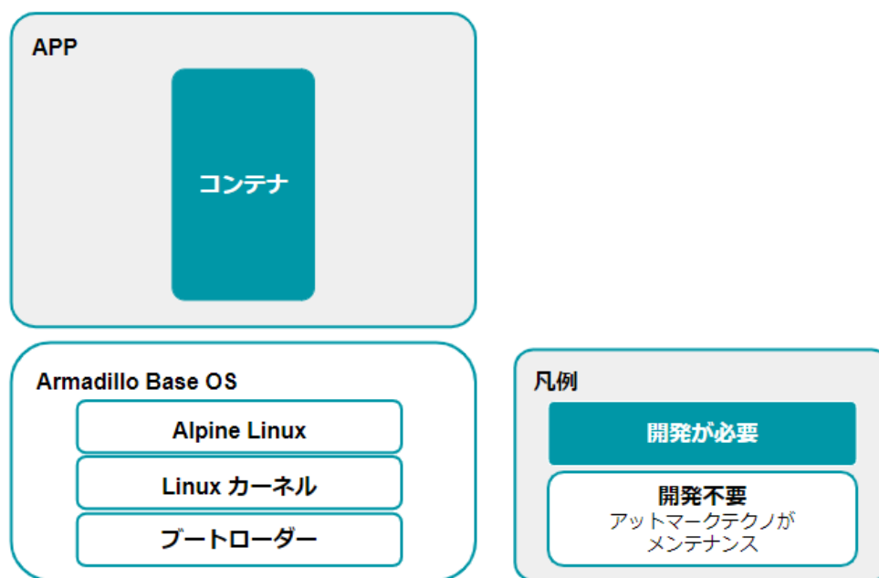
図 3.144 開発者が開発するもの、開発しなくていいもの
