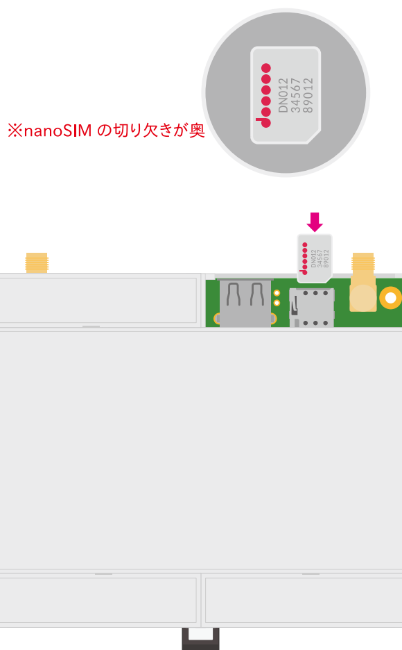
図 3.88 nanoSIM カードの接続例
