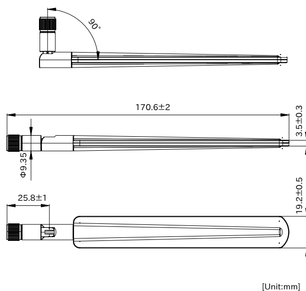
図 3.70 LTE 外付けアンテナ形状図
