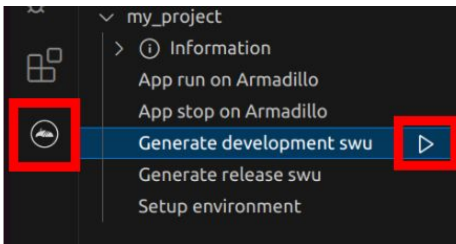
図 3.215 VS Code でコンテナイメージの作成を行う
