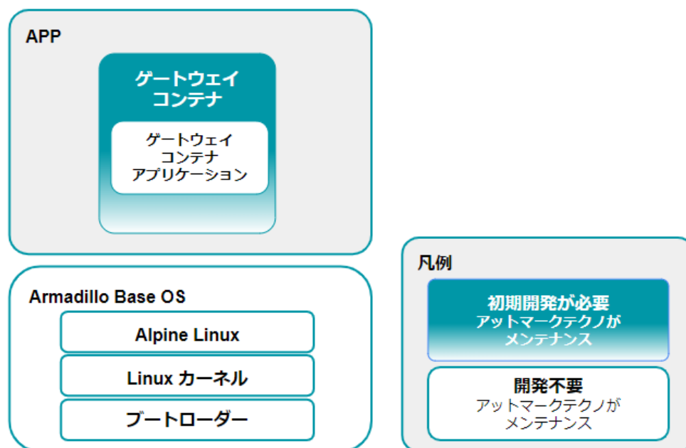
図 3.145 ゲートウェイコンテナ使用時、開発者が開発するもの、開発しなくていいもの
