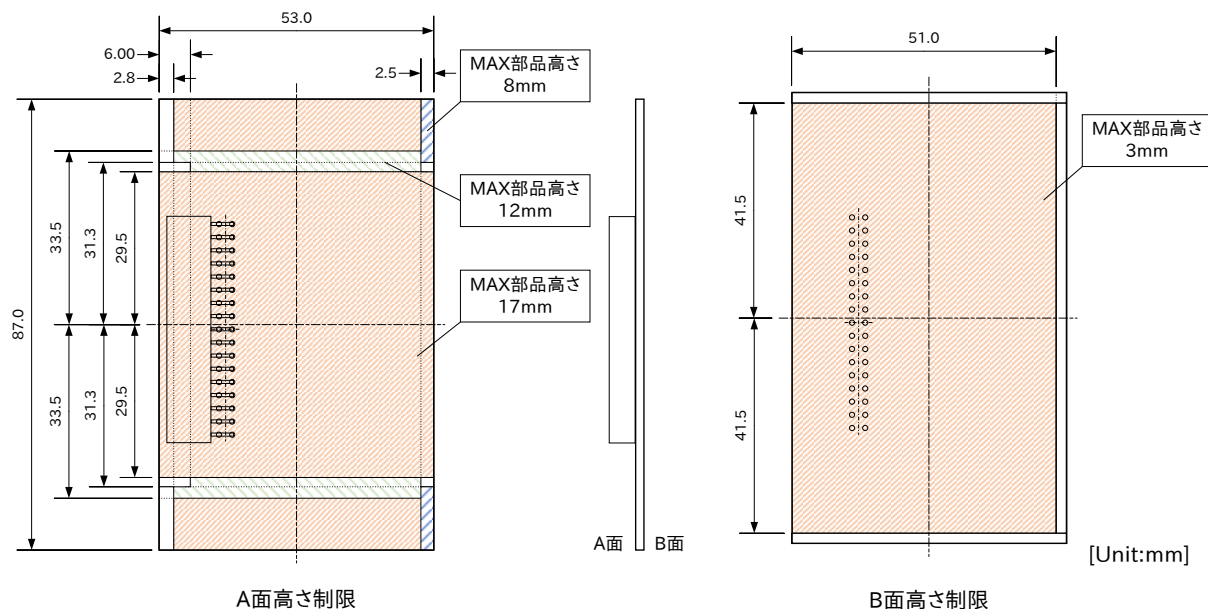
図 3.59 水平方向に拡張する場合の部品高さ制限
