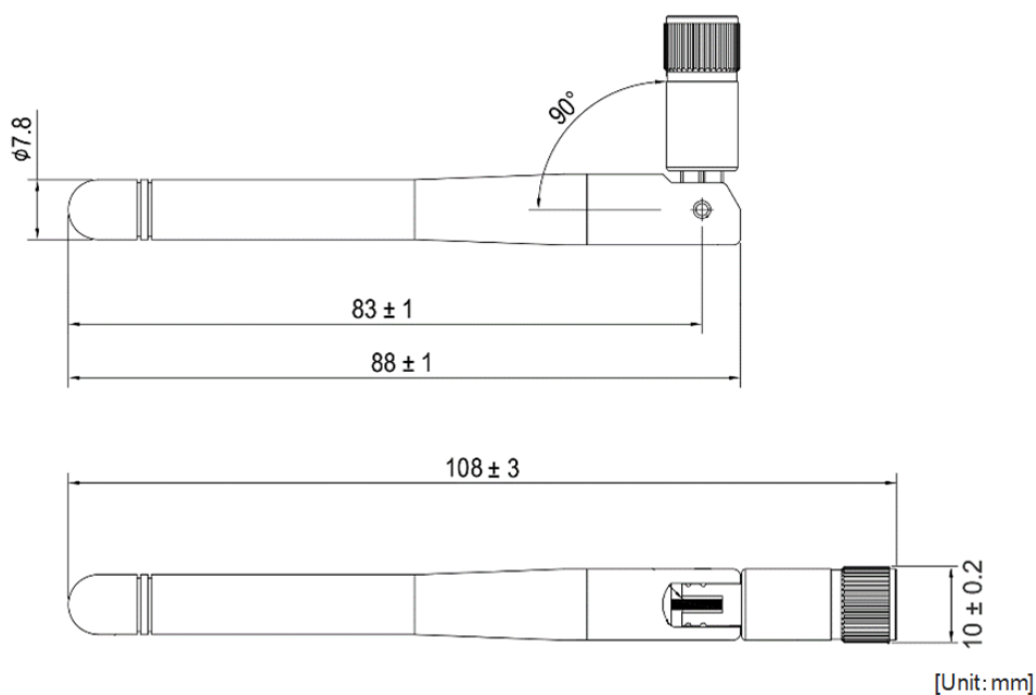
図 3.69 WLAN/BT/TH 外付けアンテナ形状図
