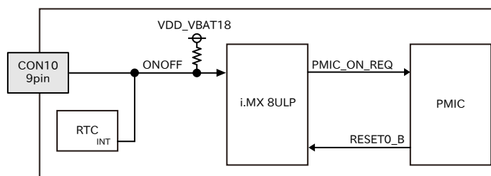
図 3.65 ONOFF 回路の構成
