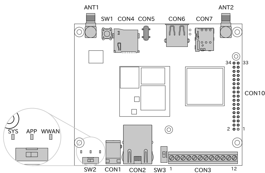
図 3.71 Armadillo-IoT ゲートウェイ A9E のインターフェース 表面
