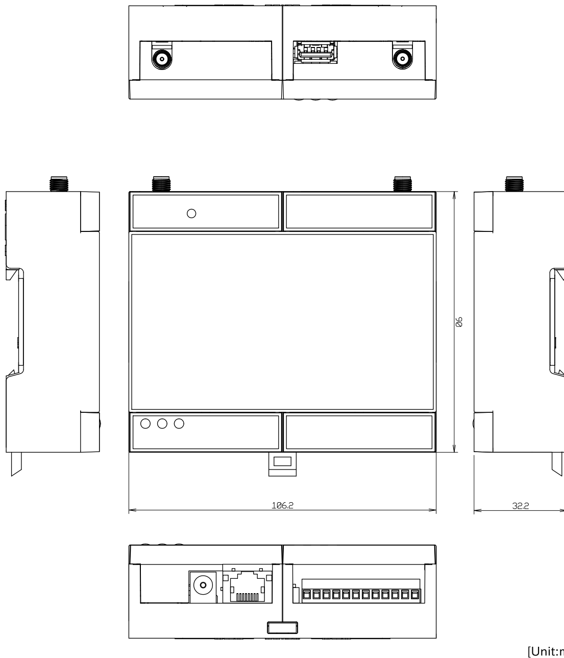
図 3.60 筐体形状
