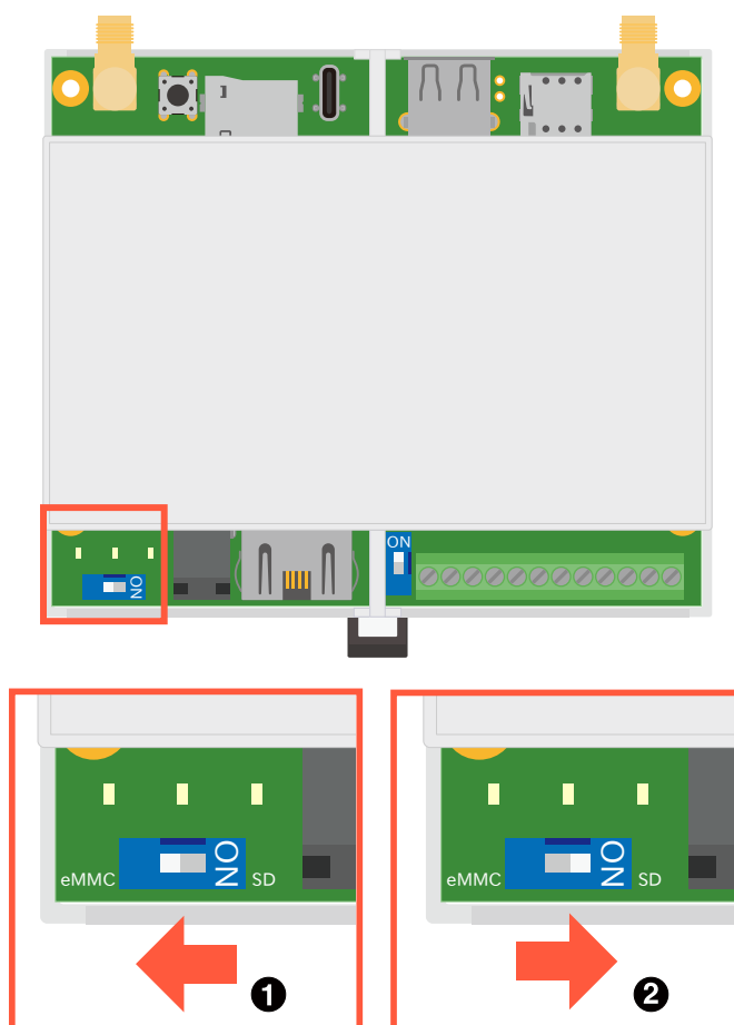
図 3.14 起動デバイス設定スイッチの操作
