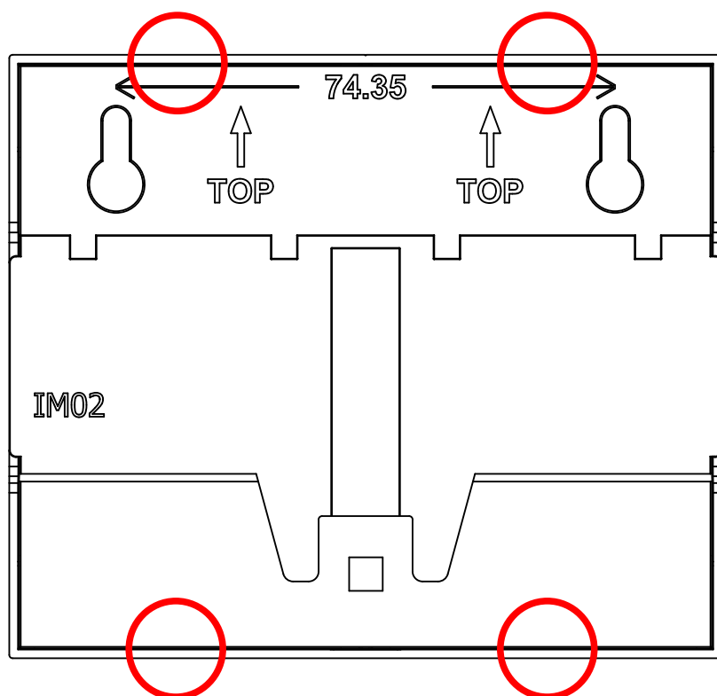
図 3.69 ケースボトムのツメ
