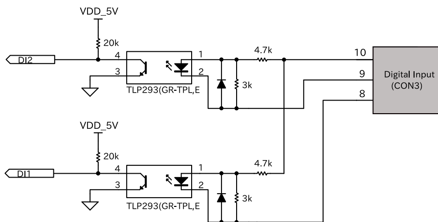
図 3.95 CON3 接点入力内部回路
