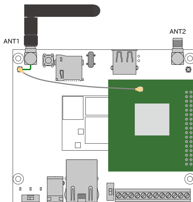
図 3.54 拡張基板に搭載した無線モジュールで外付けアンテナを使用する場合のイメージ(ANT1 使用)
