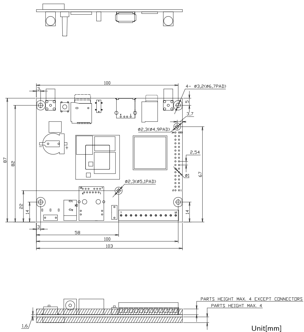
図 3.61 基板形状図（外形、固定穴、部品高さ）
