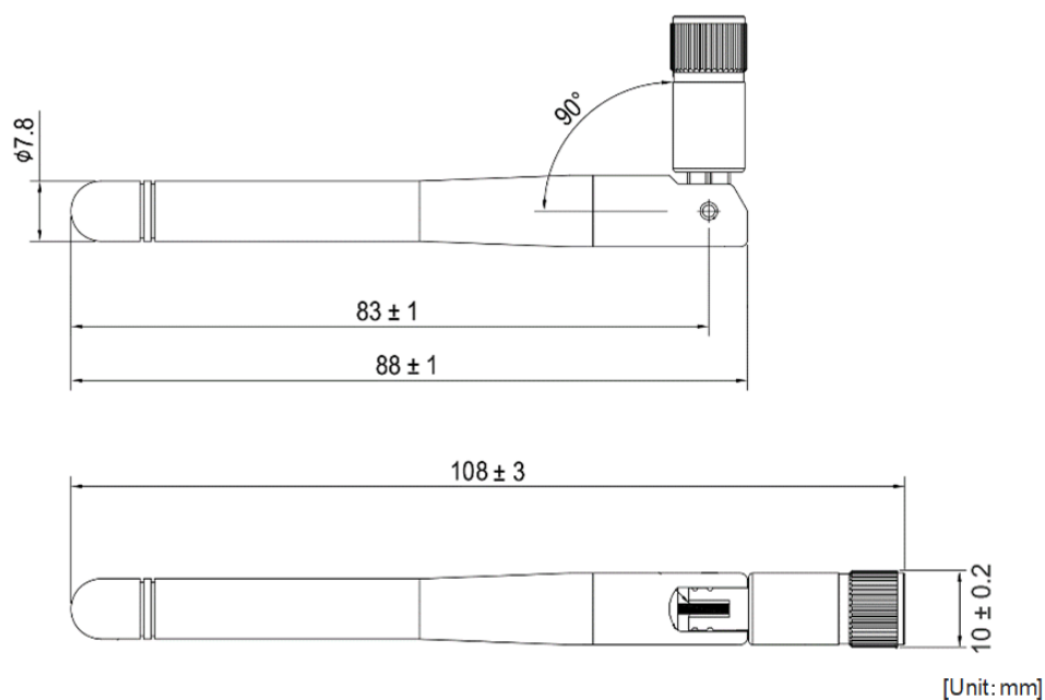
図 3.63 WLAN/BT/TH 外付けアンテナ形状図
