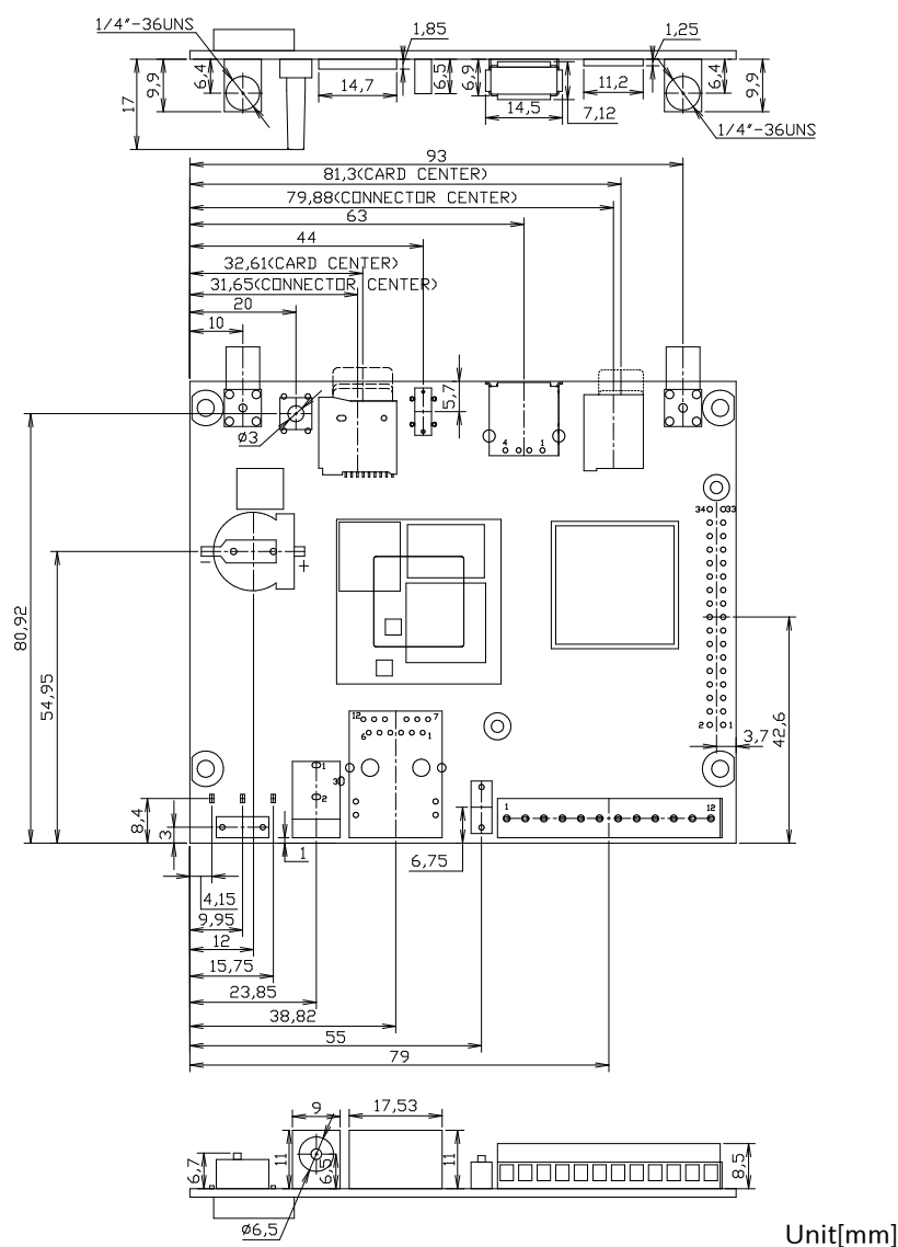
図 3.62 基板形状図（コネクタ、スイッチ、LED 位置）
