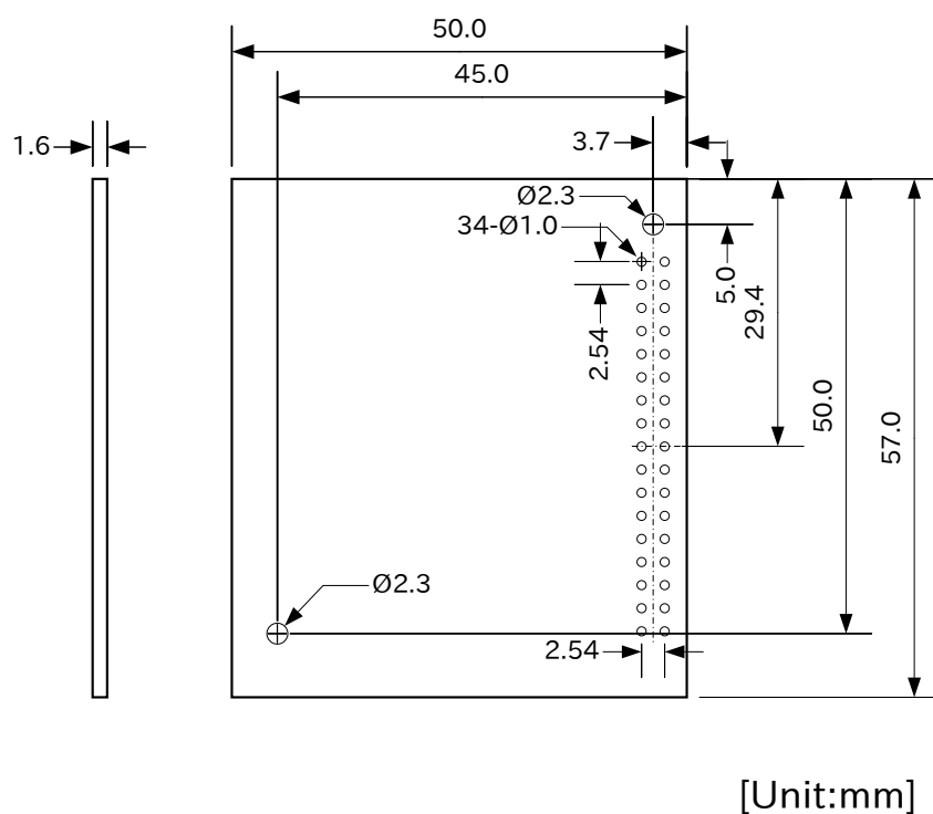
図 3.48 垂直方向に拡張する場合の基板形状図
