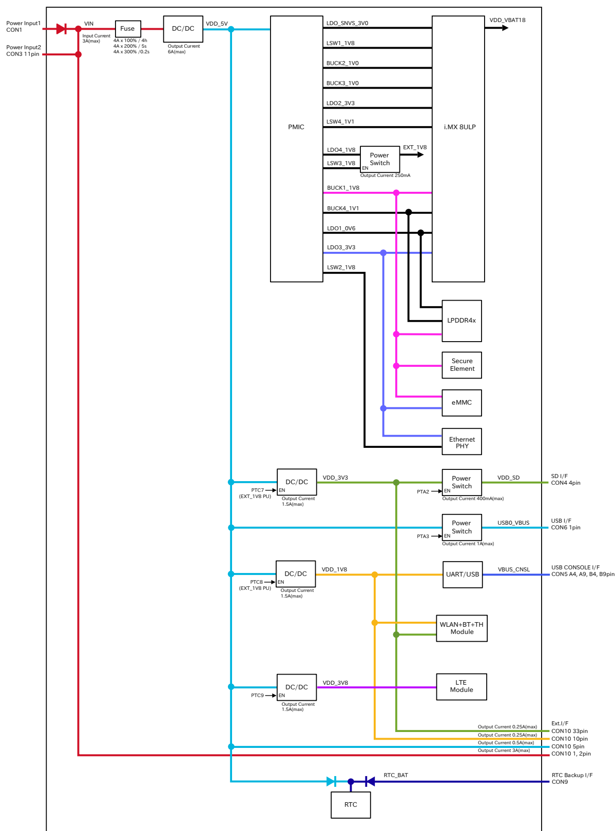
図 3.57 電源回路の構成
