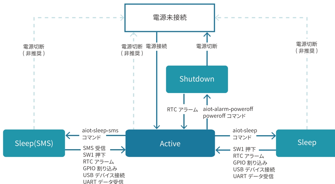
図 3.140 状態遷移図
