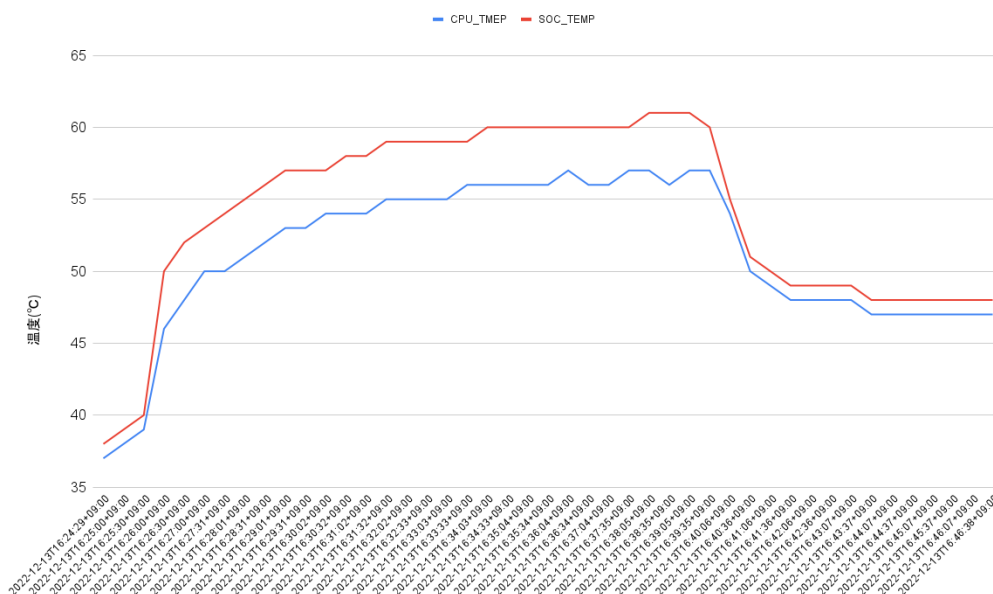
図 6.198 Armadillo-IoT ゲートウェイ G4 で取得した温度のグラフ
