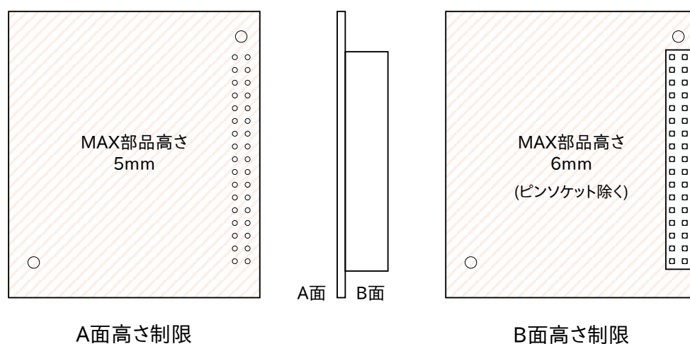
図 3.49 垂直方向に拡張する場合の搭載部品高さ制限
