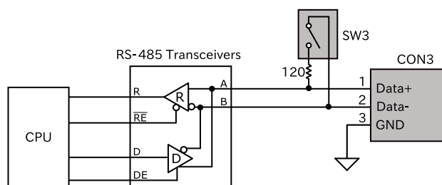
図 3.104 CON3 RS-485 内部回路
