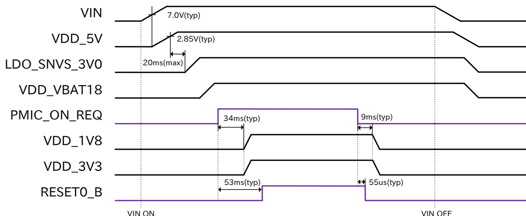
図 3.58 電源シーケンス
