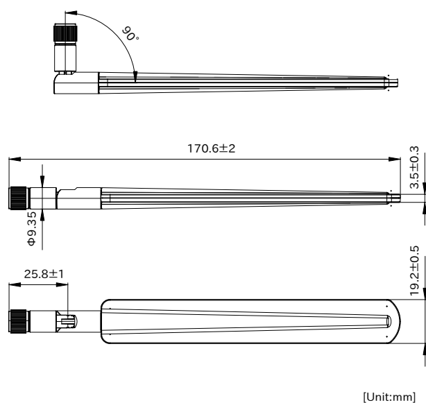
図 3.64 LTE 外付けアンテナ形状図
