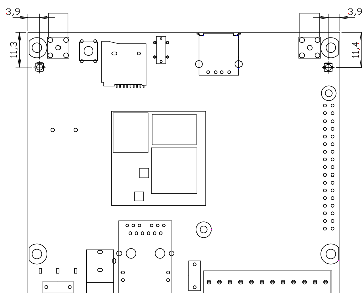
図 3.56 基板上の U.FL コネクタの位置
