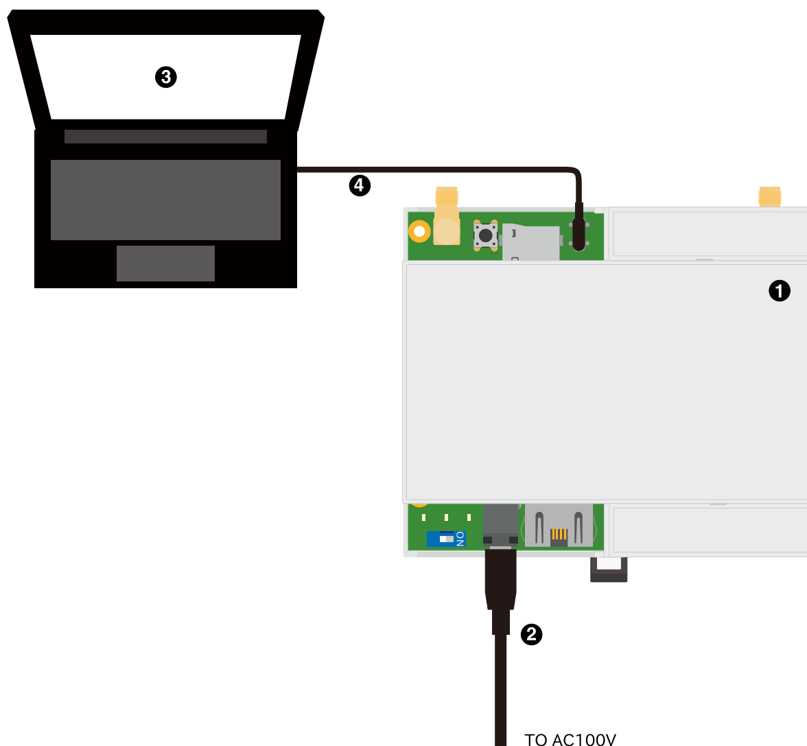
図 3.41 シリアルコンソールを使用する配線例
