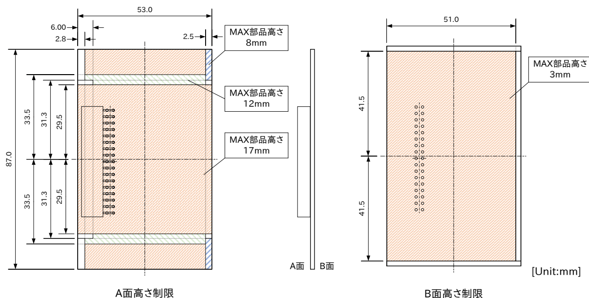
図 3.53 水平方向に拡張する場合の部品高さ制限
