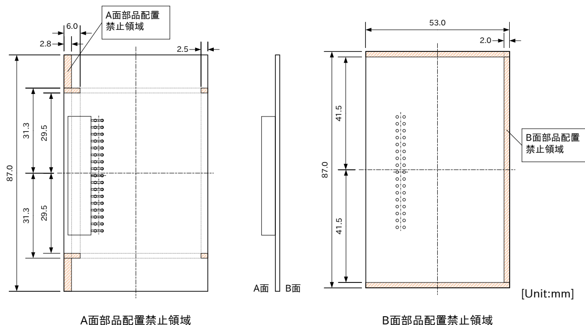
図 3.52 水平方向に拡張する場合の部品配置禁止領域
