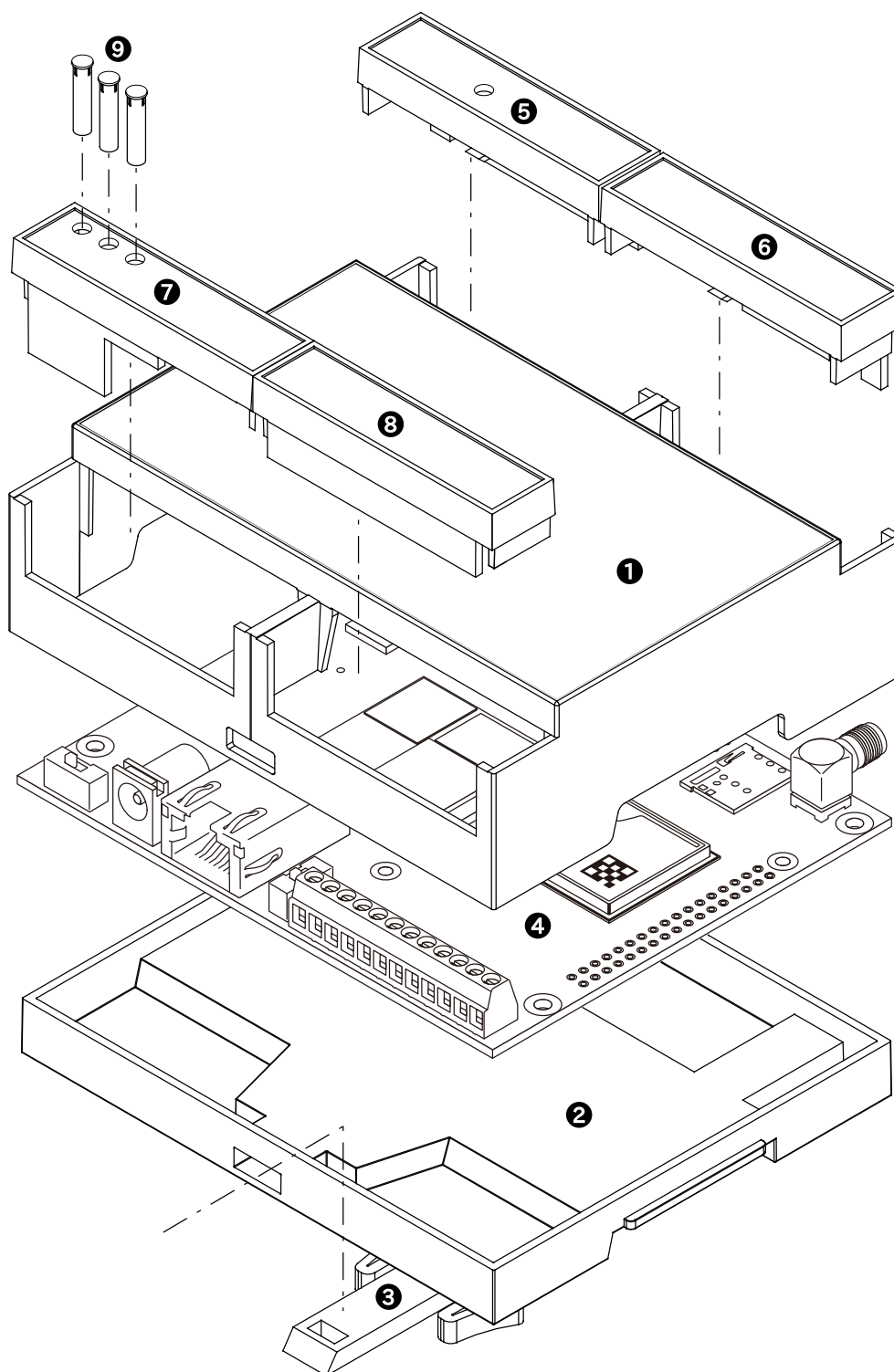
図 3.65 ケースモデル展開図
