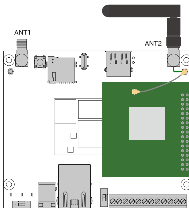
図 3.55 拡張基板に搭載した無線モジュールで外付けアンテナを使用する場合のイメージ(ANT2 使用)
