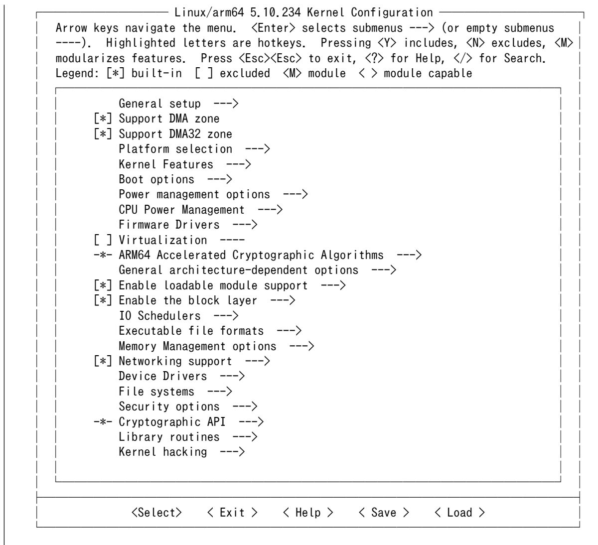
図 6.224 Linux カーネルコンフィギュレーション設定画面
