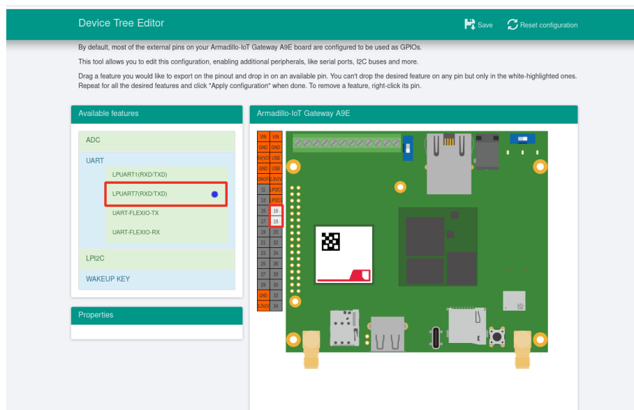
図 6.209 LPUART7(RXD/TXD) のドラッグ
