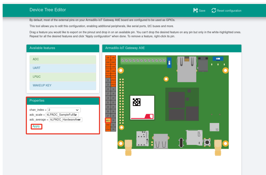
図 6.212 プロパティの設定
