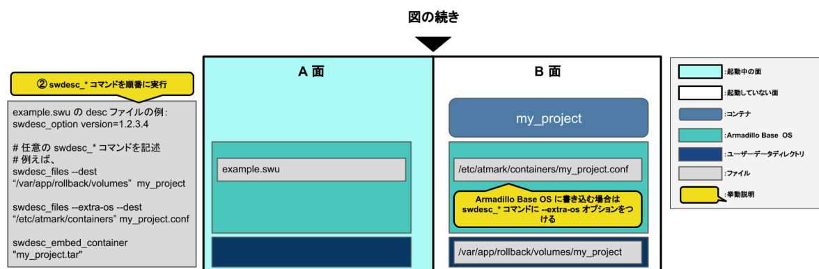
図 6.21 desc ファイルに記述した swudesc_* コマンドを実行
