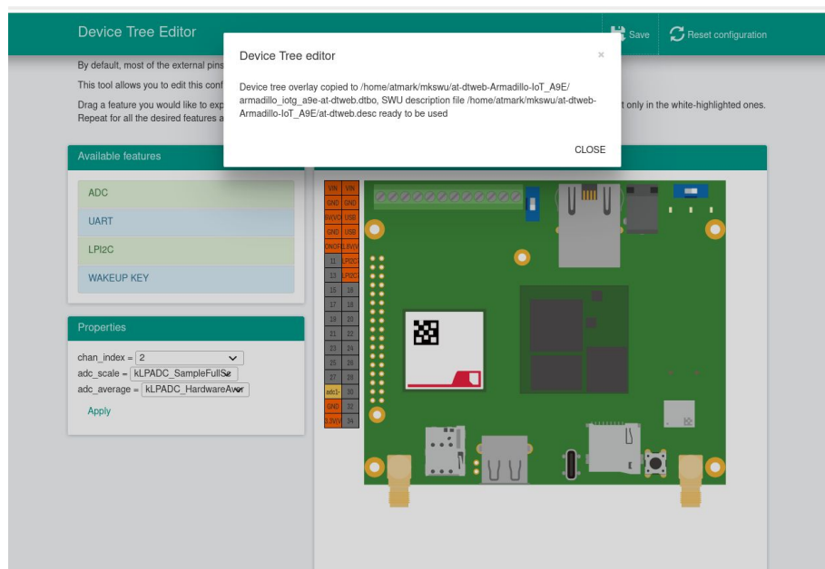
図 6.216 dtbo/desc の生成完了
