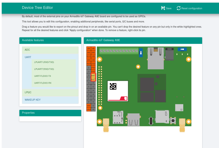
図 6.210 CON10 16/18 ピンへのドロップ
