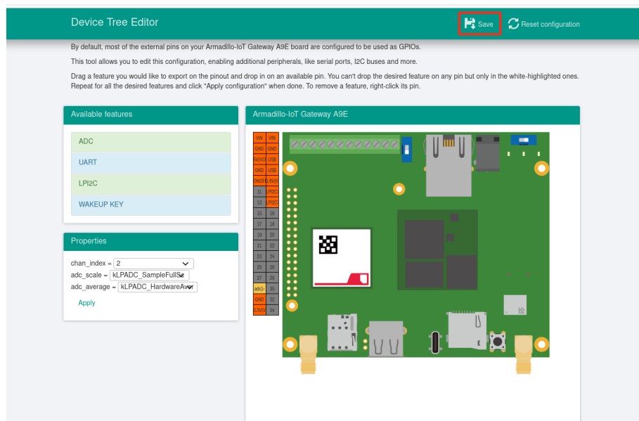
図 6.215 dtbo/desc ファイルの生成
