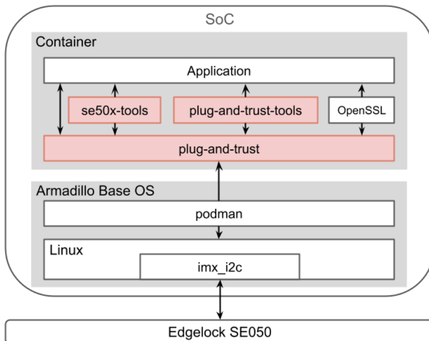
図 6.259 Plug & Trust Middleware の周辺のソフトウェアスタック
