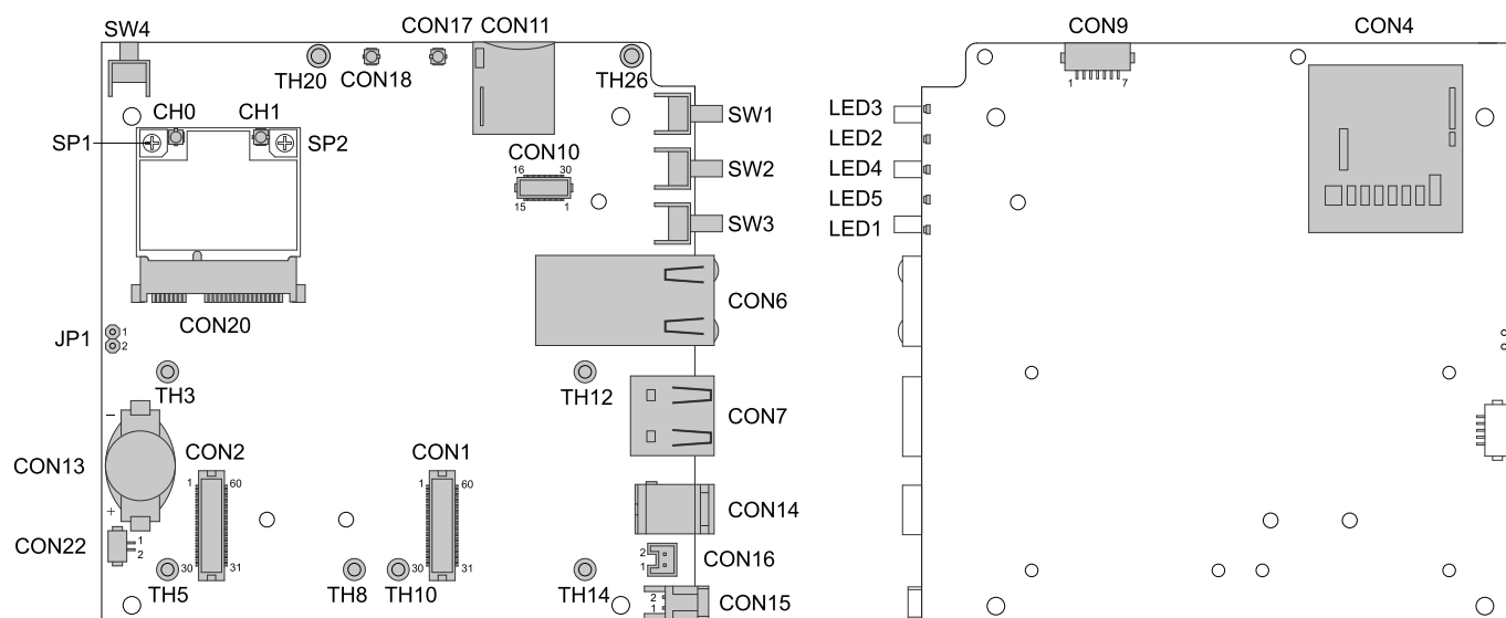
図 4.6 インターフェースレイアウト図(AGX314*、AEH-AR9462 搭載) [3]
