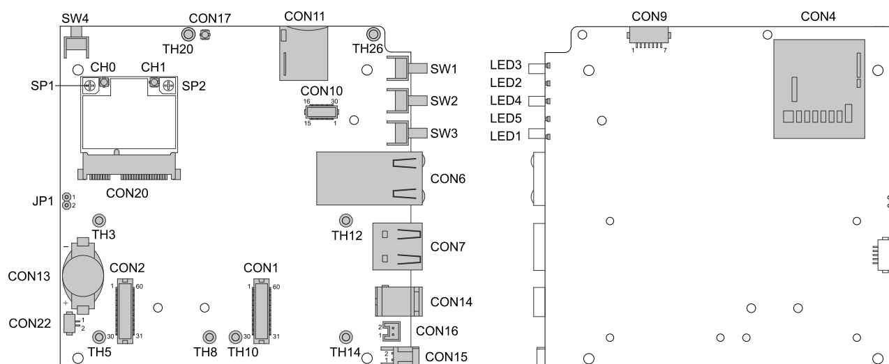
図 4.8 インターフェースレイアウト図(AGX3*2*) [5]
