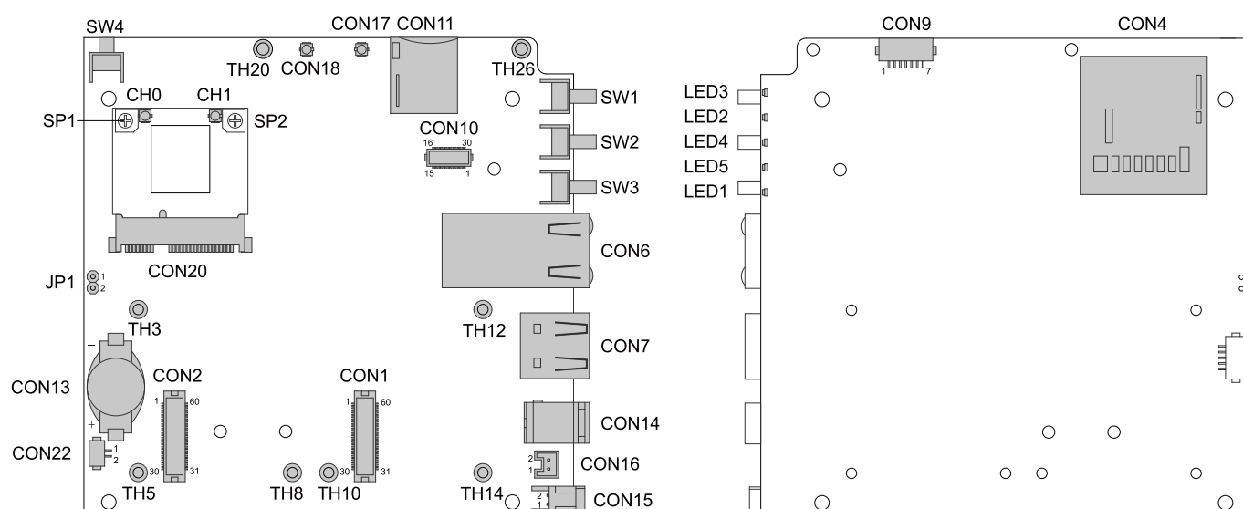
図 4.7 インターフェースレイアウト図(AGX314*、WPEB-265AXI(BT) [B33] 搭載) [4]
