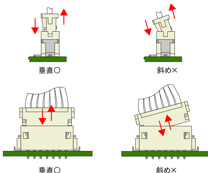
図 17.5 挿抜角度
