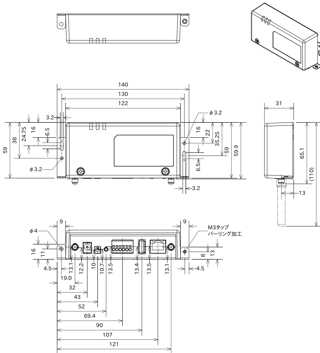
図 18.1 筐体形状図
