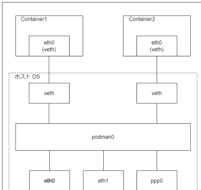
図 11.29 ブリッジモードの構成
