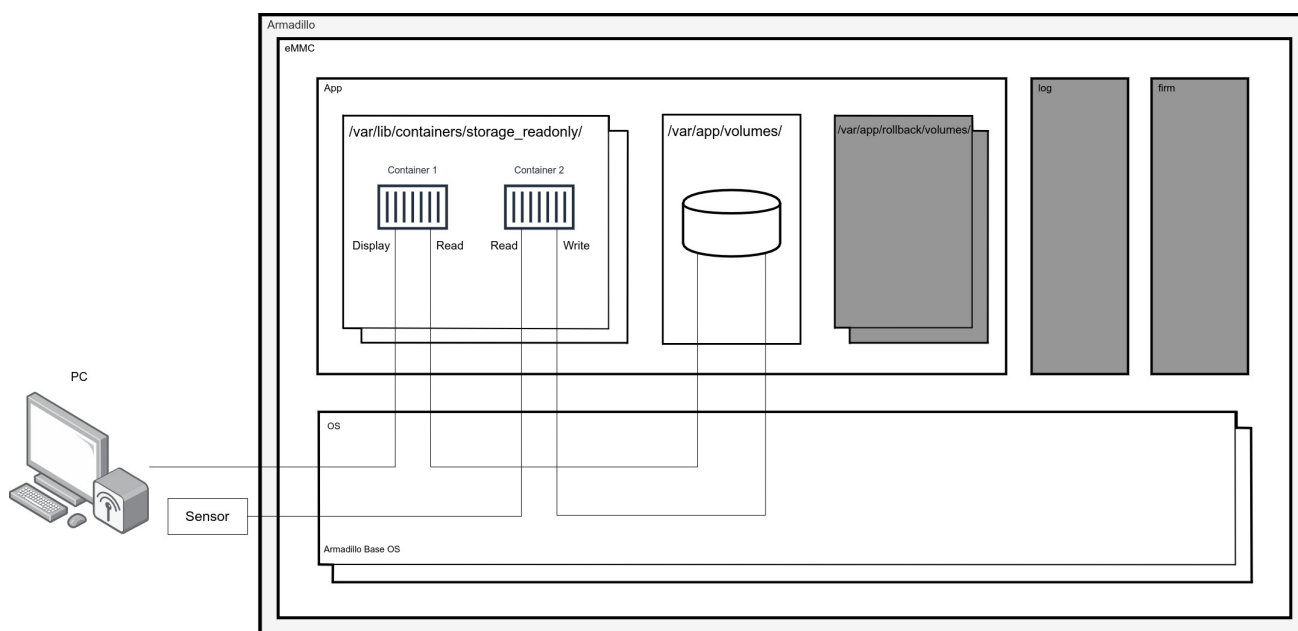
図 11.14 センサから読み取ったデータを PC に出力するシステム構成図
