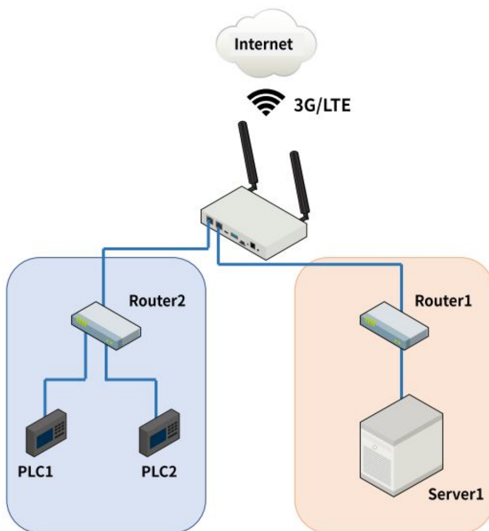
図 11.35 ネットワークの構成
