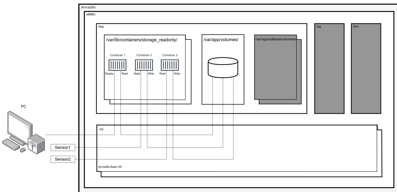
図 11.16 複数のセンサからデータを読み取るシステム構成図
