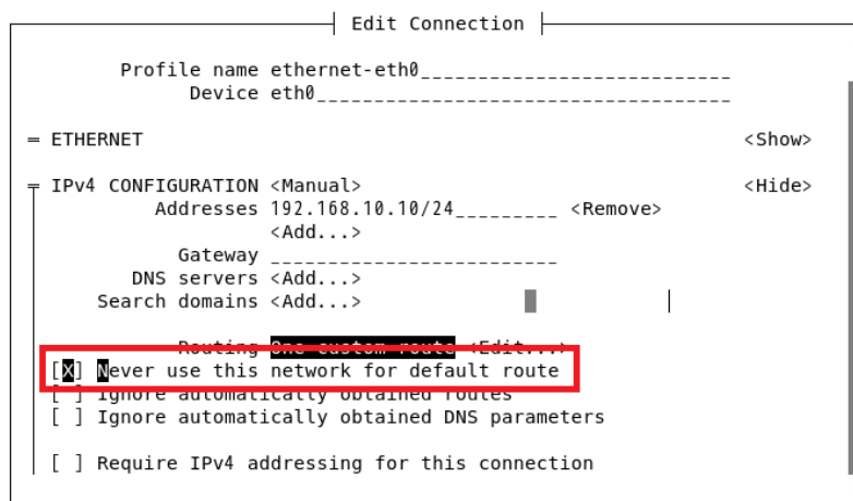
図 11.44 nmtui デフォルトゲートウェイ無効化
