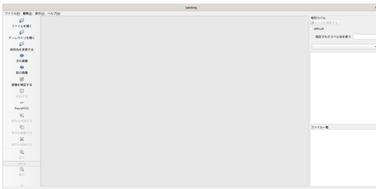
図 6.13 labellmg の起動
