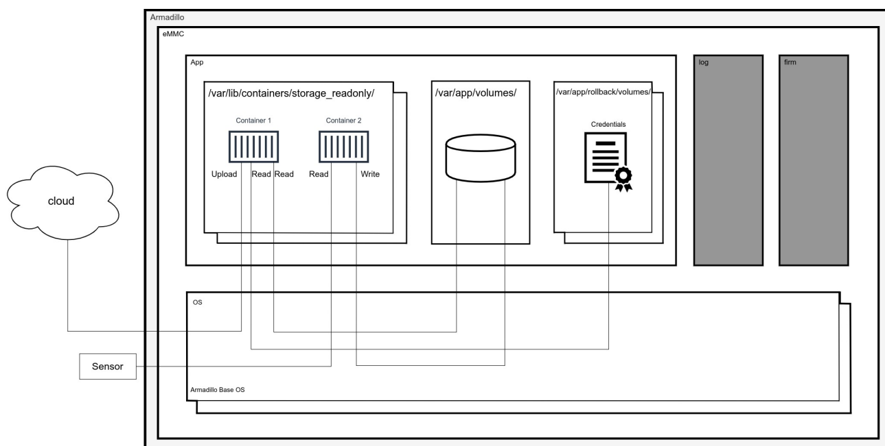
図 11.15 センサからデータを読み取りクラウドに出力するシステム構成図
