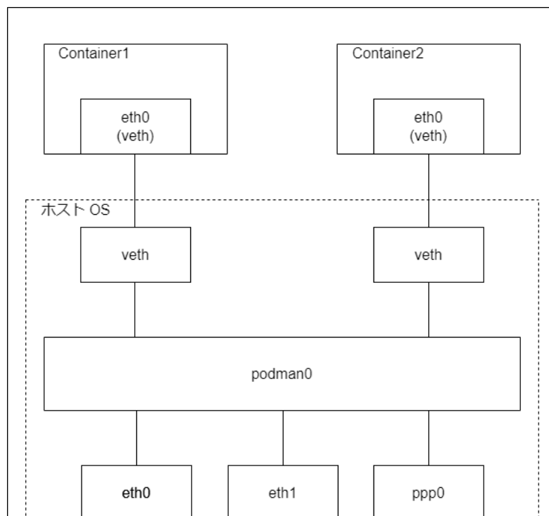
図 11.29 ブリッジモードの構成
